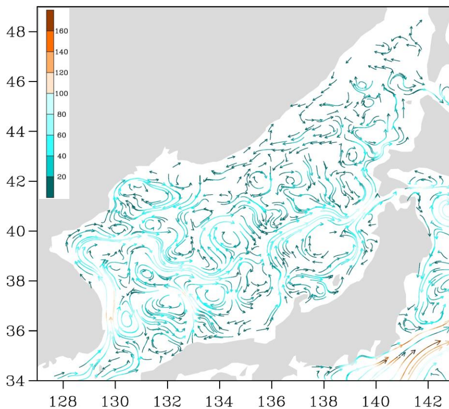
Рис. 3-3 Поверхностные течения Японского моря, 25 ноября 2019 г.
