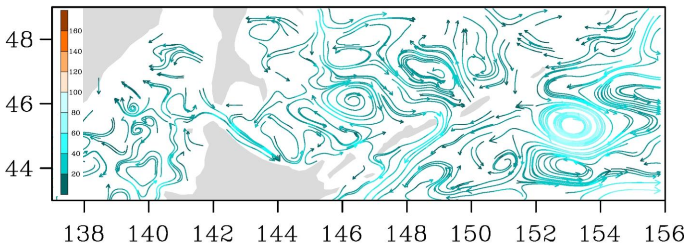
Рис. 3-9 Поверхностные течения, пролив Лаперуза, 25 ноября 2019 г.
