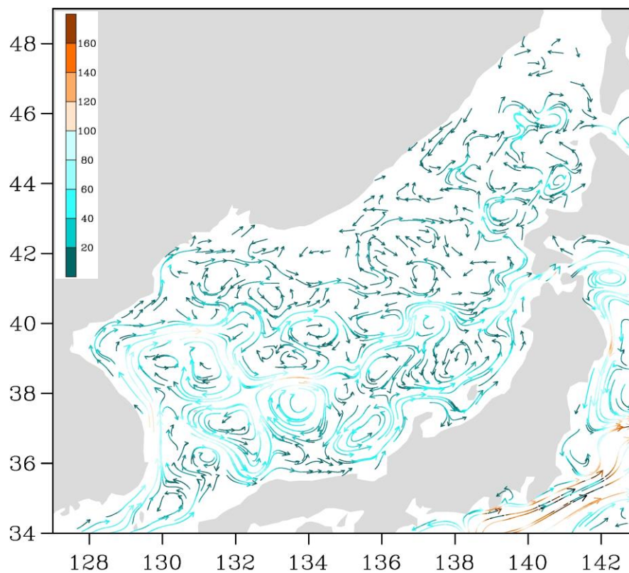
Рис. 3-1 Поверхностные течения Японского моря, 05 ноября 2019 г.
