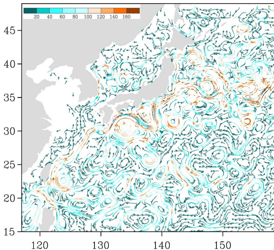
Рис. 3-4 Поверхностные течения западной части Тихого океана, 5 ноября 2019 г.
