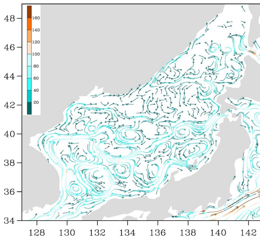
Рис. 3-2 Поверхностные течения Японского моря, 15 ноября 2019 г.
