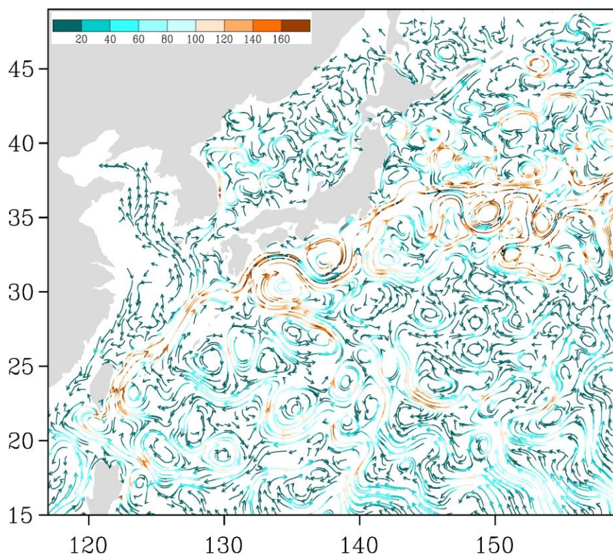
Рис. 3-6 Поверхностные течения западной части Тихого океана, 25 ноября 2019 г.
