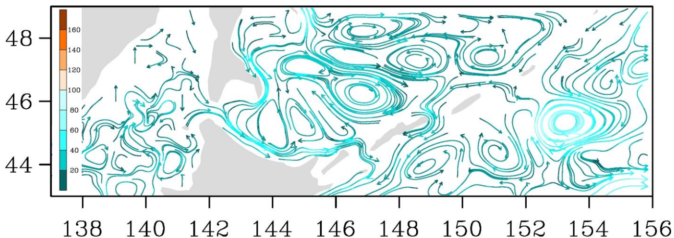
Рис. 3-7 Поверхностные течения, пролив Лаперуза, 5 ноября 2019 г.
