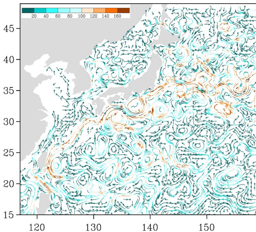
Рис. 3-5 Поверхностные течения западной части Тихого океана, 15 ноября 2019 г.
