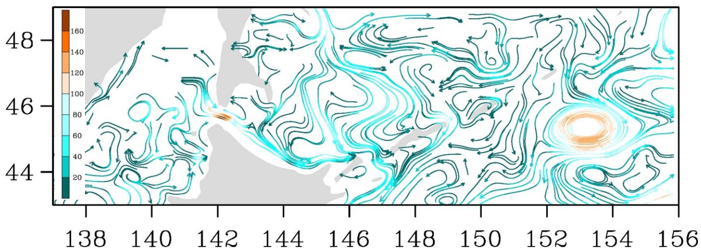
Рис. 3-8 Поверхностные течения, пролив Лаперуза, 15 ноября 2019 г.
