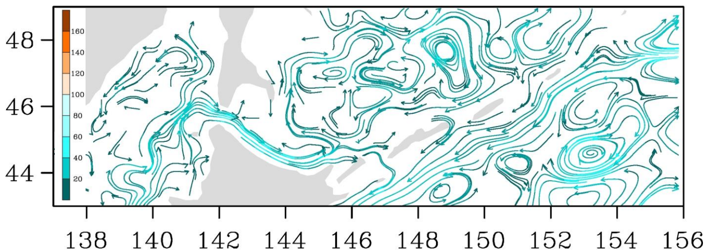
Рис. 3-7 Поверхностные течения, пролив Лаперуза, 5 сентября 2020 г.
