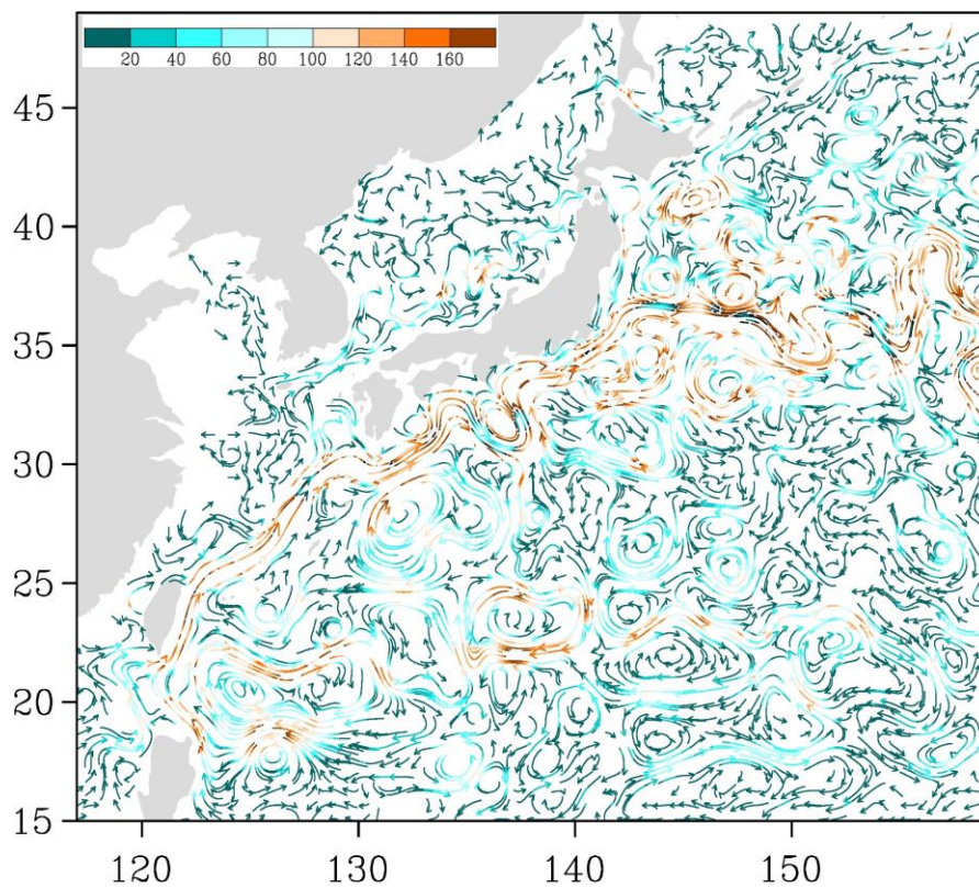
Рис. 3-4 Поверхностные течения западной части Тихого океана, 5 сентября 2020 г.
