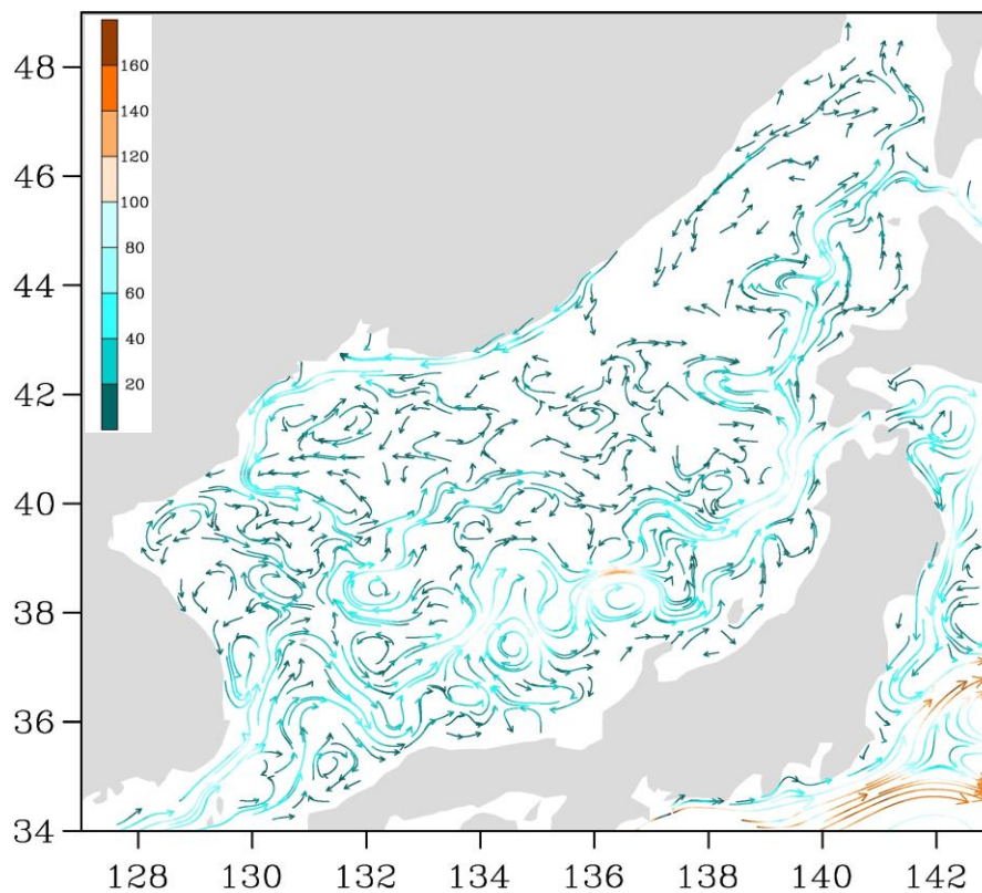
Рис. 3-2 Поверхностные течения Японского моря, 15 сентября 2020 г.
