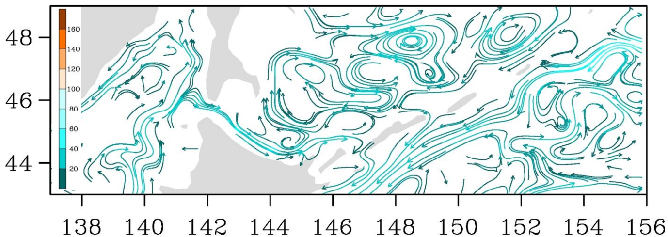
Рис. 3-9 Поверхностные течения, пролив Лаперуза, 25 сентября 2020 г.
