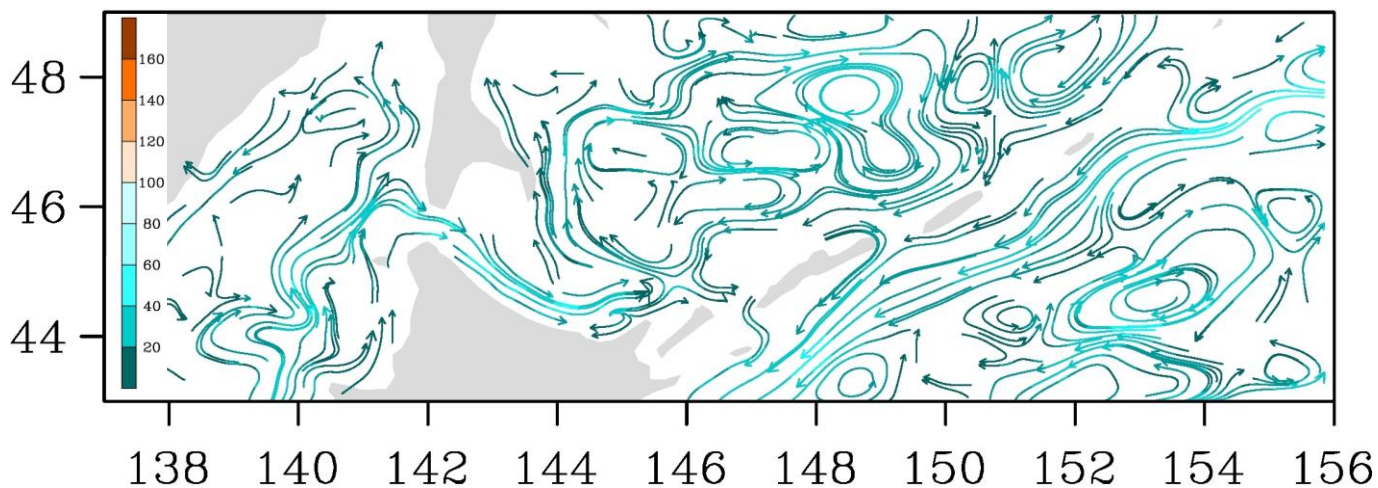
Рис. 3-8 Поверхностные течения, пролив Лаперуза, 15 сентября 2020 г.
