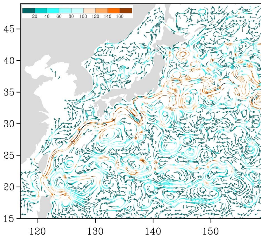
Рис. 3-5 Поверхностные течения западной части Тихого океана, 15 сентября 2020 г.
