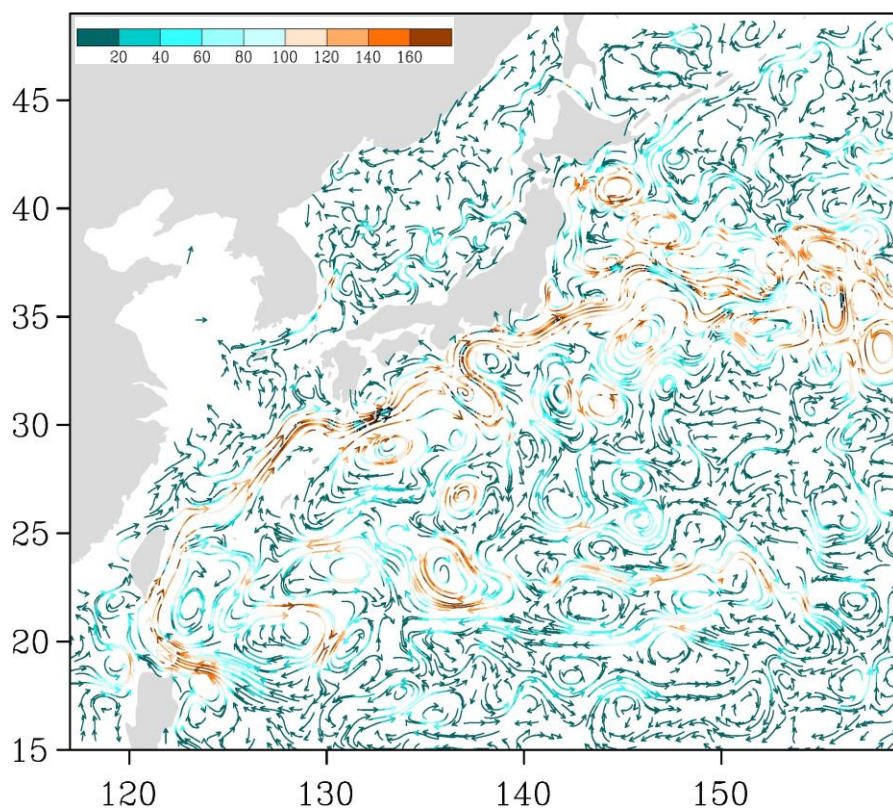
Рис. 3-6 Поверхностные течения западной части Тихого океана, 25 сентября 2020 г.
