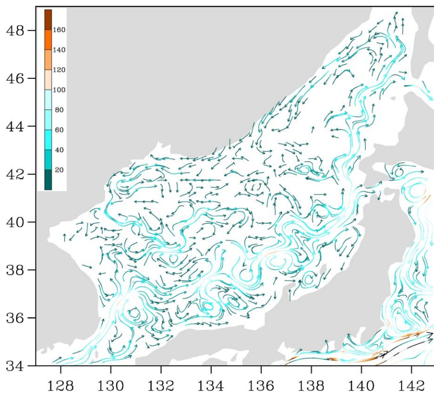
Рис. 3-3 Поверхностные течения Японского моря, 25 сентября 2020 г.
