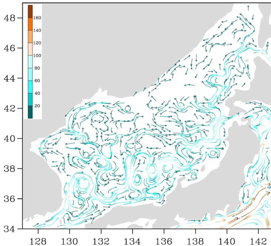
Рис. 3-1 Поверхностные течения Японского моря, 05 сентября 2020 г.
