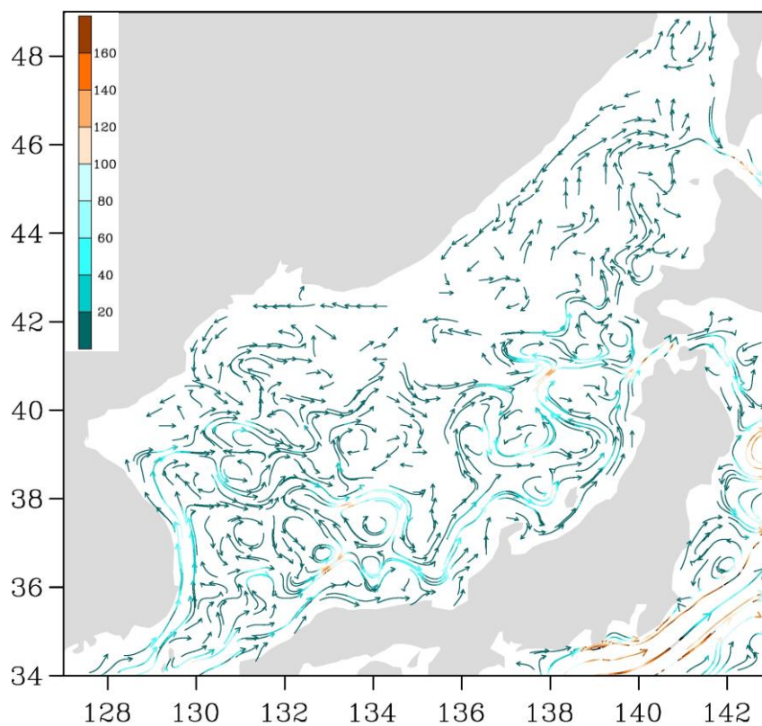
Рис. 3-3 Поверхностные течения Японского моря, 25 мая 2021 г.
