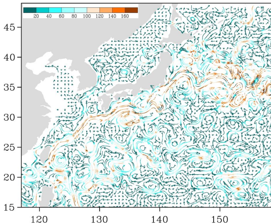
Рис. 3-4 Поверхностные течения западной части Тихого океана, 5 мая 2021 г.
