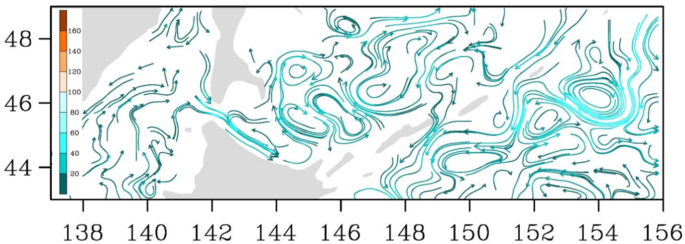
Рис. 3-9 Поверхностные течения, южная часть Охотского моря, 25 мая 2021 г.
