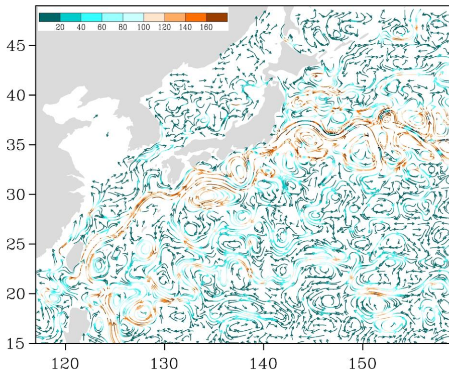
Рис. 3-5 Поверхностные течения западной части Тихого океана, 15 мая 2021 г.
