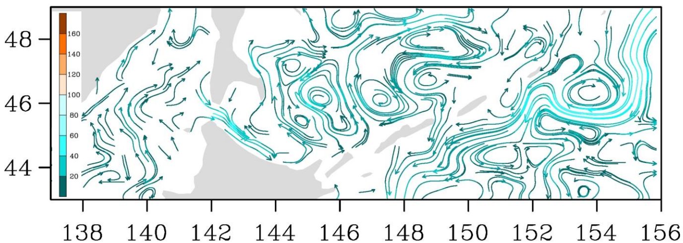
Рис. 3-8 Поверхностные течения, южная часть Охотского моря, 15 мая 2021 г.
