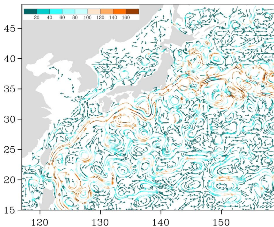
Рис. 3-6 Поверхностные течения западной части Тихого океана, 25 мая 2021 г.
