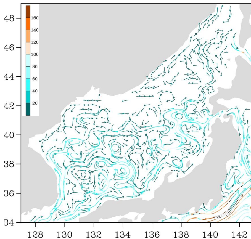
Рис. 3-2 Поверхностные течения Японского моря, 15 апреля 2021 г.
