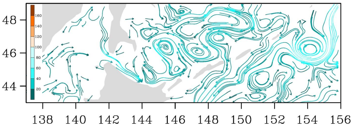
Рис. 3-7 Поверхностные течения, южная часть Охотского моря, 5 мая 2021 г.
