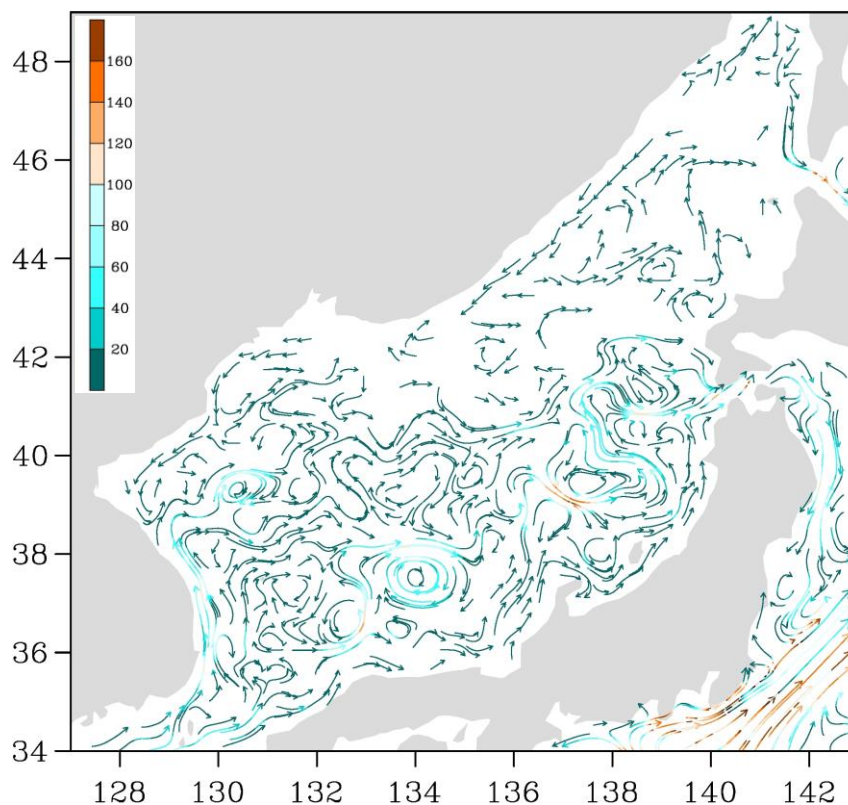
Рис. 3-1 Поверхностные течения Японского моря, 05 мая 2021 г.
