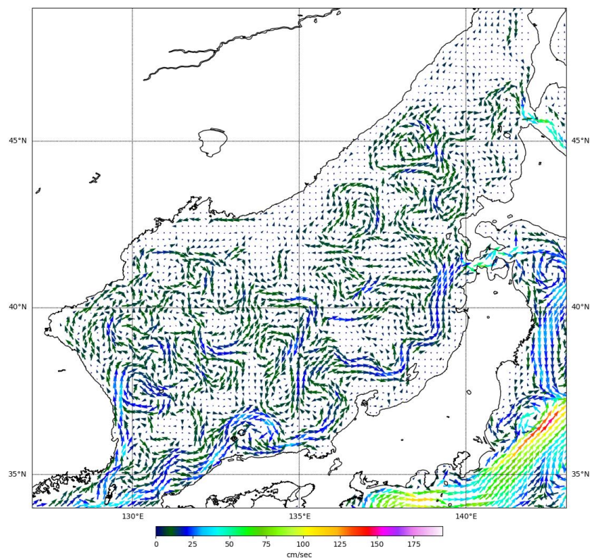
Рис. 3-1 Поверхностные течения Японского моря, 05 апреля 2025 г.
