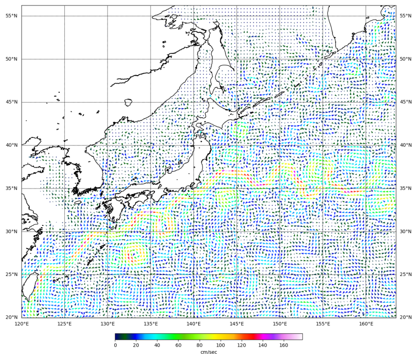
Рис. 3-5 Поверхностные течения западной части Тихого океана, 15 апреля 2025 г.
