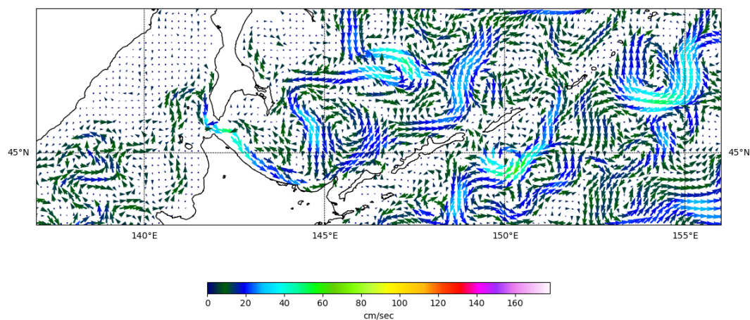
Рис. 3-8 Поверхностные течения, южная часть Охотского моря, 15 апреля 2025 г.
