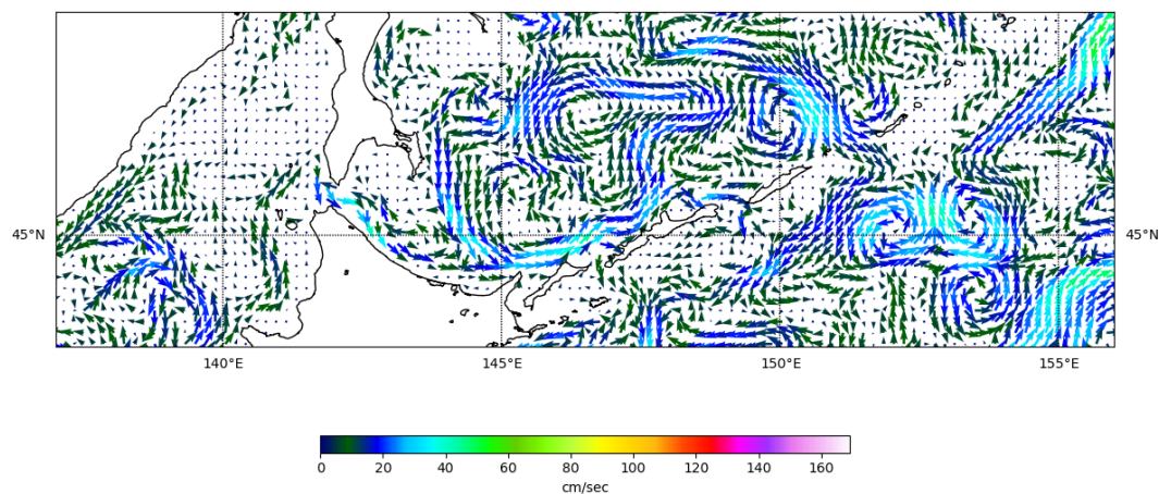
Рис. 3-9 Поверхностные течения, южная часть Охотского моря, 25 апреля 2025 г.
