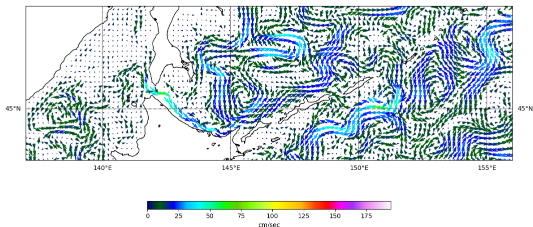
Рис. 3-7 Поверхностные течения, южная часть Охотского моря, 5 апреля 2025 г.
