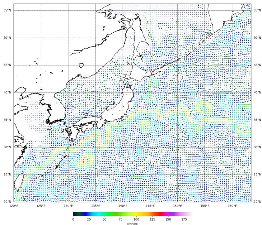
Рис. 3-4 Поверхностные течения западной части Тихого океана, 5 апреля 2025 г.
