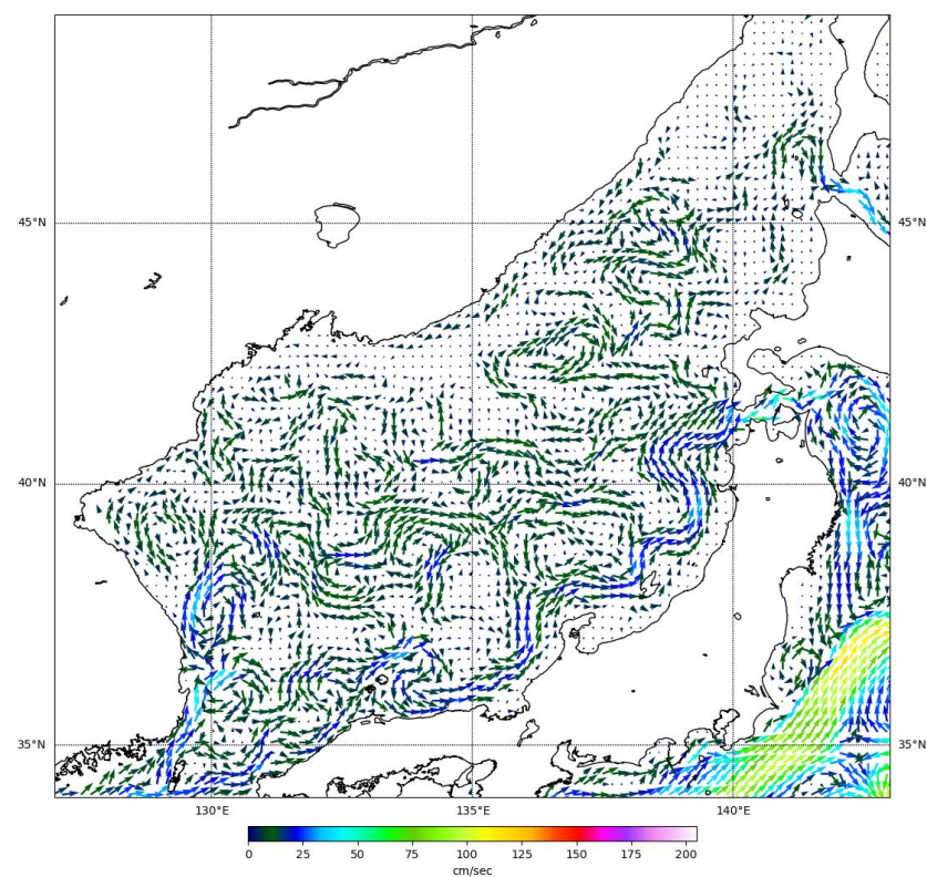
Рис. 3-3 Поверхностные течения Японского моря, 25 апреля 2025 г.
