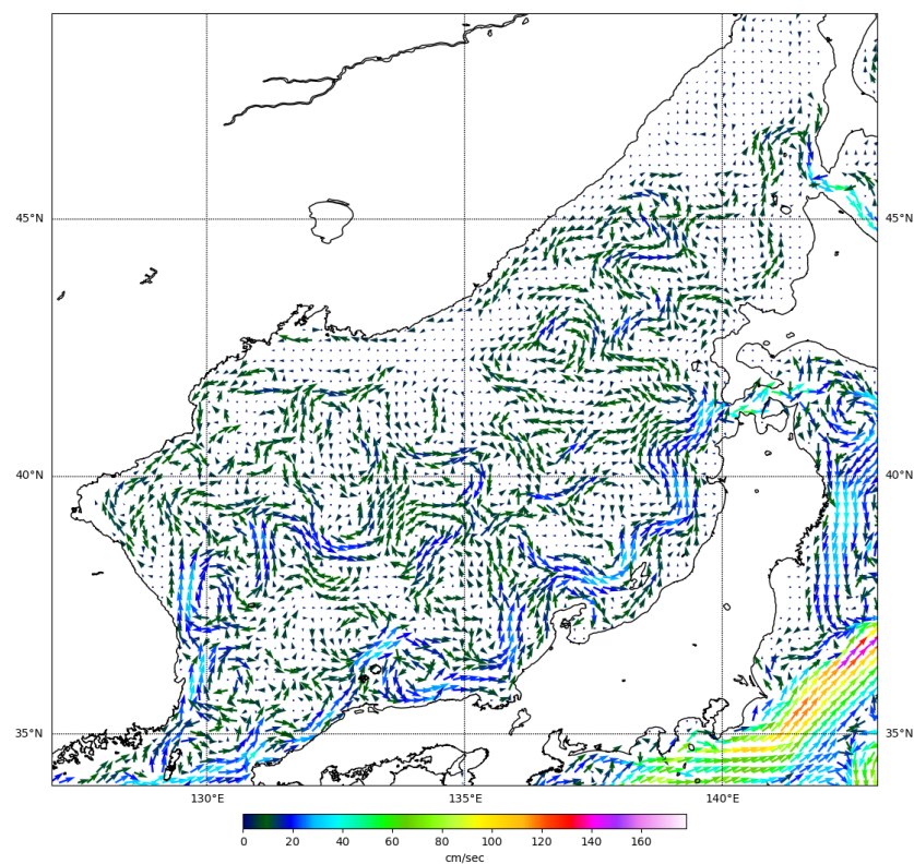
Рис. 3-2 Поверхностные течения Японского моря, 15 апреля 2025 г.
