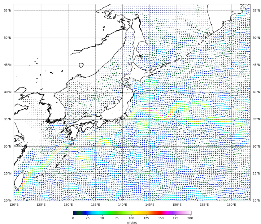
Рис. 3-6 Поверхностные течения западной части Тихого океана, 25 апреля 2025 г.
