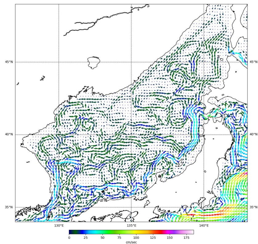
Рис. 3-3 Поверхностные течения Японского моря, 25 мая 2025 г.
