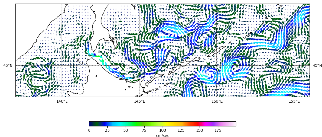
Рис. 3-7 Поверхностные течения, южная часть Охотского моря, 5 мая 2025 г.
