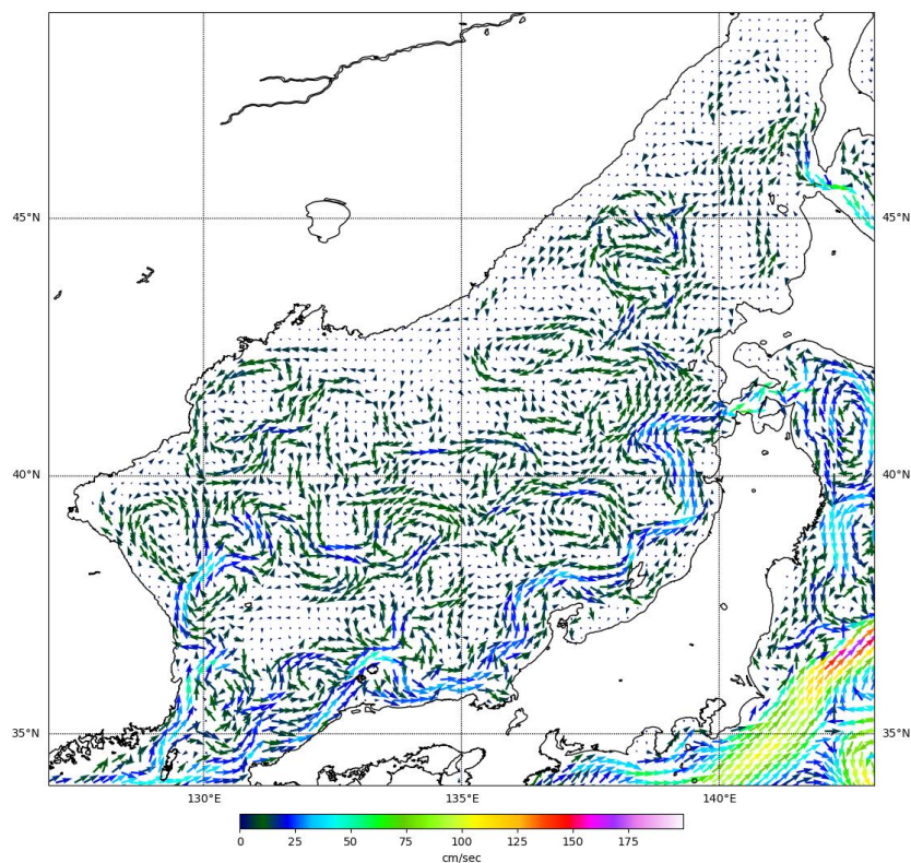
Рис. 3-1 Поверхностные течения Японского моря, 05 мая 2025 г.
