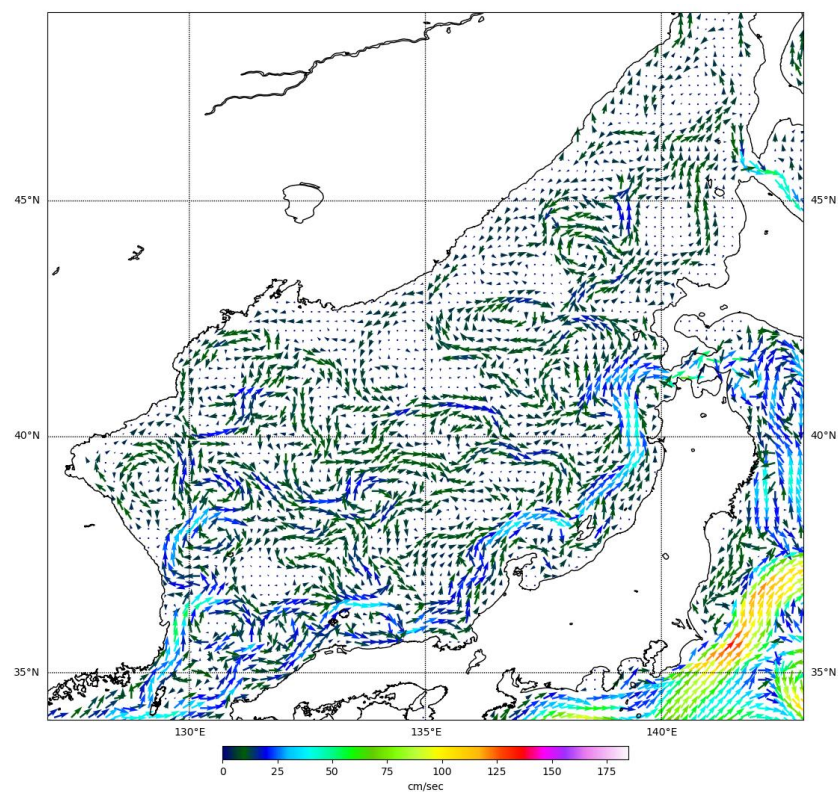
Рис. 3-2 Поверхностные течения Японского моря, 15 мая 2025 г.
