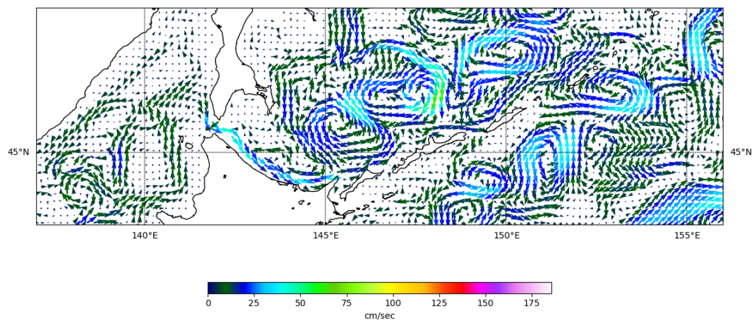
Рис. 3-9 Поверхностные течения, южная часть Охотского моря, 25 мая 2025 г.
