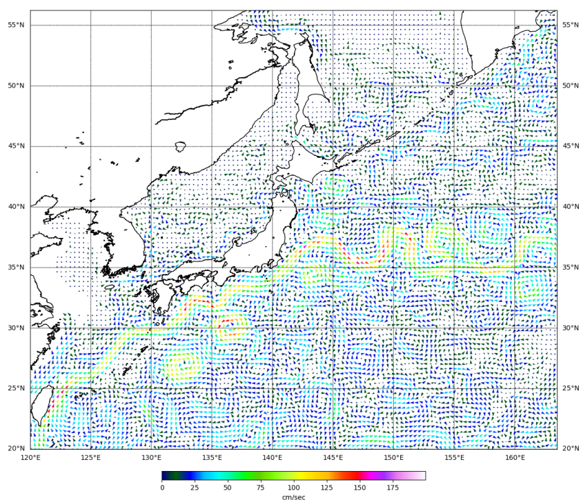
Рис. 3-4 Поверхностные течения западной части Тихого океана, 5 мая 2025 г.
