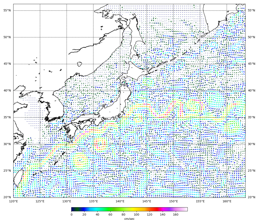
Рис. 3-5 Поверхностные течения западной части Тихого океана, 15 мая 2025 г.
