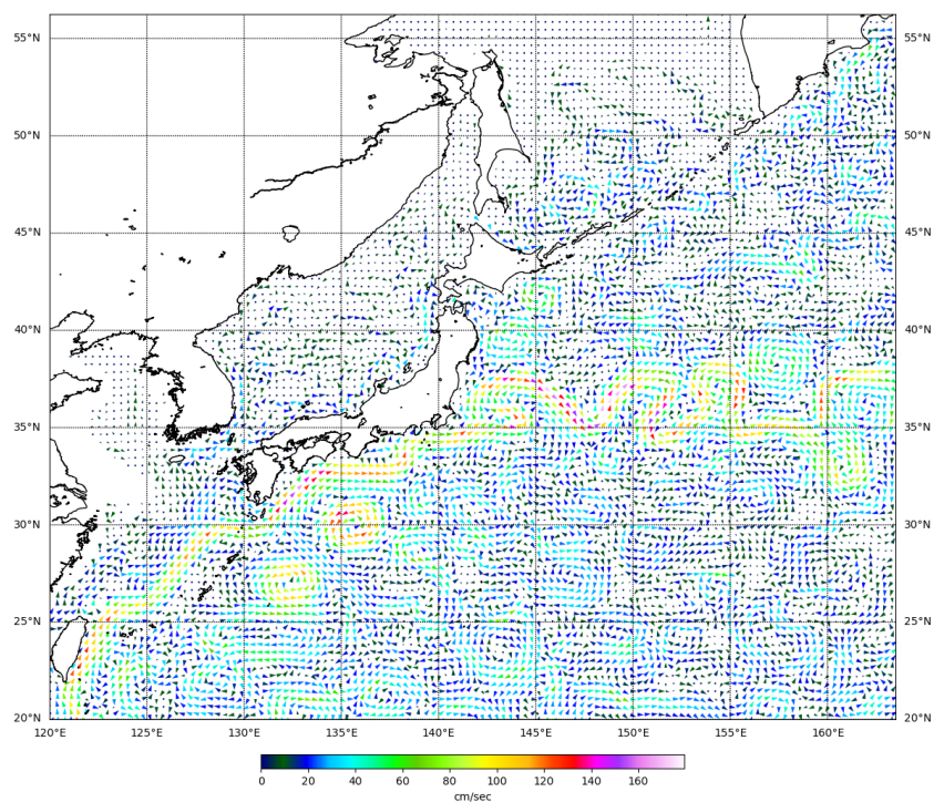
Рис. 3-6 Поверхностные течения западной части Тихого океана, 25 мая 2025 г.
