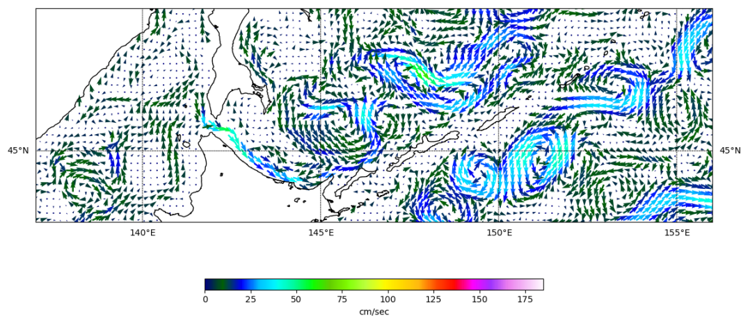
Рис. 3-8 Поверхностные течения, южная часть Охотского моря, 15 мая 2025 г.
