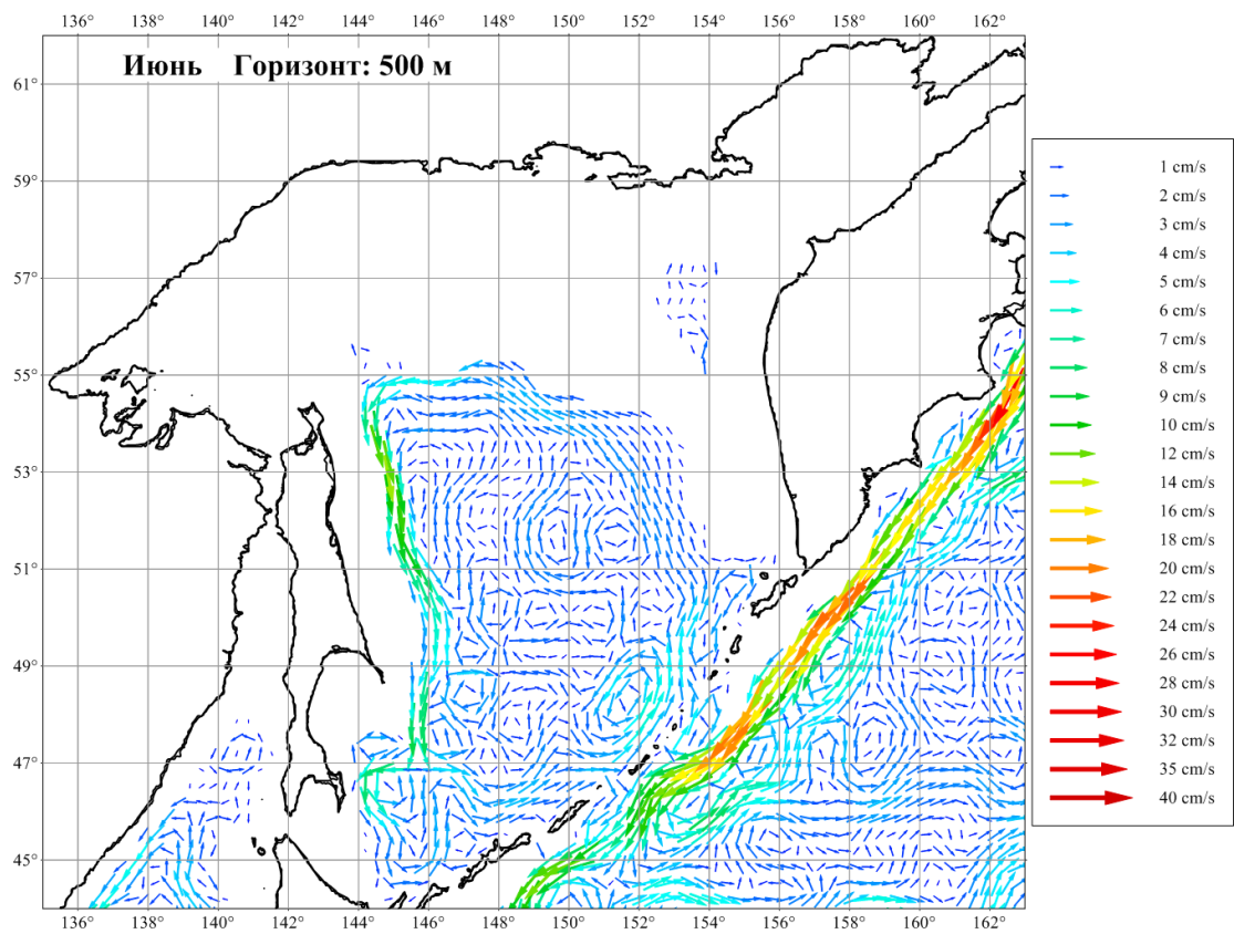
Рисунок 3.37. Течения Охотского моря в июне на горизонте 500 м
