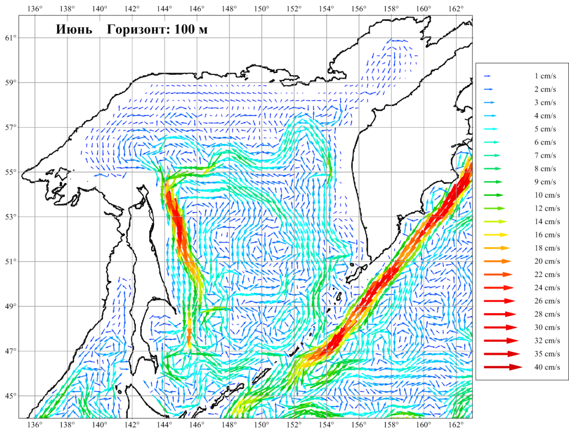
Рисунок 3.35. Течения Охотского моря в июне на горизонте 100 м
