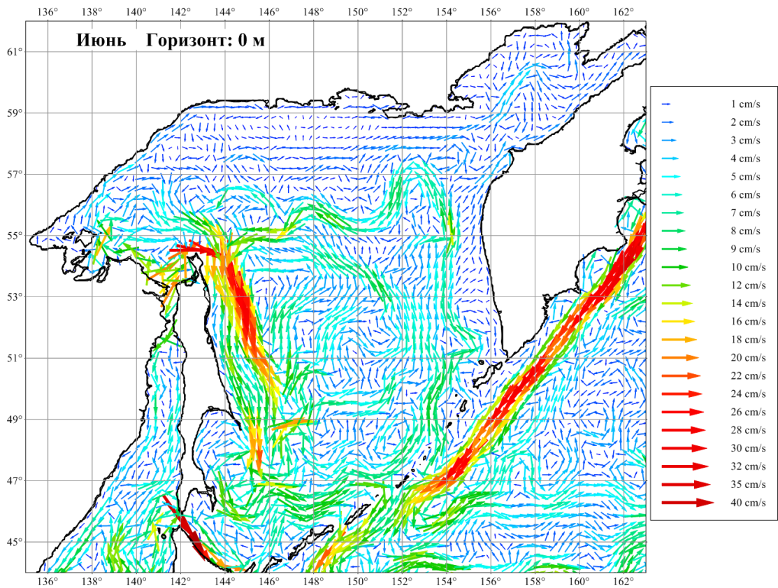
Рисунок 3.32. Течения Охотского моря в июне на горизонте 0 м
