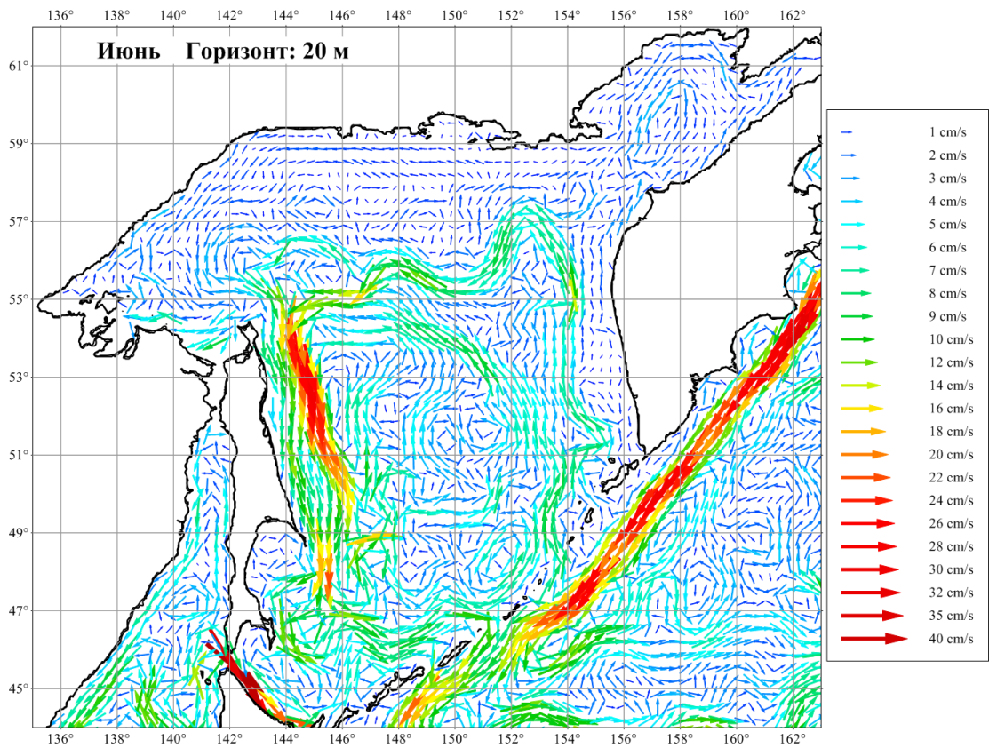
Рисунок 3.33. Течения Охотского моря в июне на горизонте 20 м
