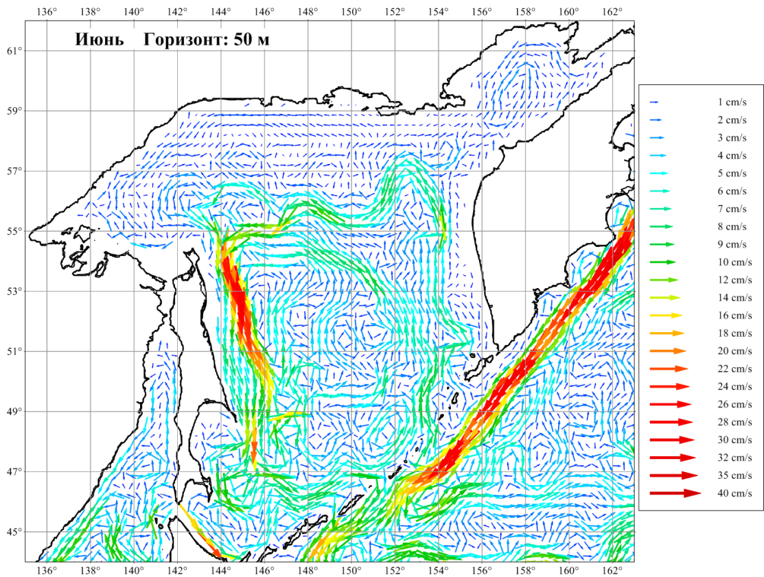
Рисунок 3.34. Течения Охотского моря в июне на горизонте 50 м
