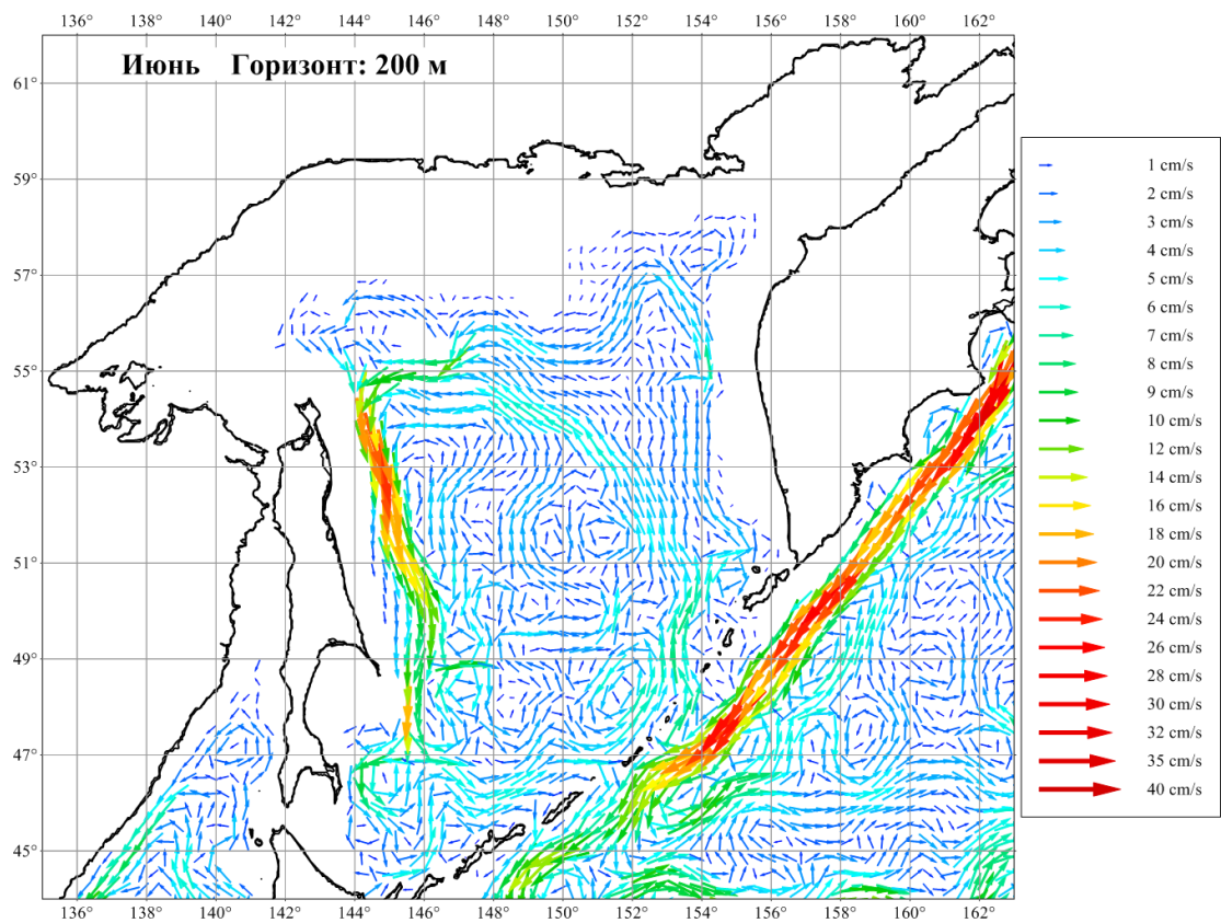
Рисунок 3.36. Течения Охотского моря в июне на горизонте 200 м
