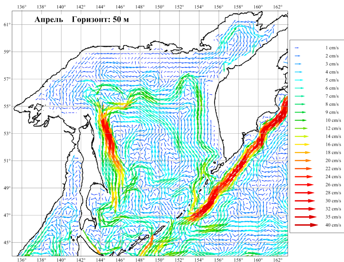
Рисунок 3.22. Течения Охотского моря в апреле на горизонте 50 м
