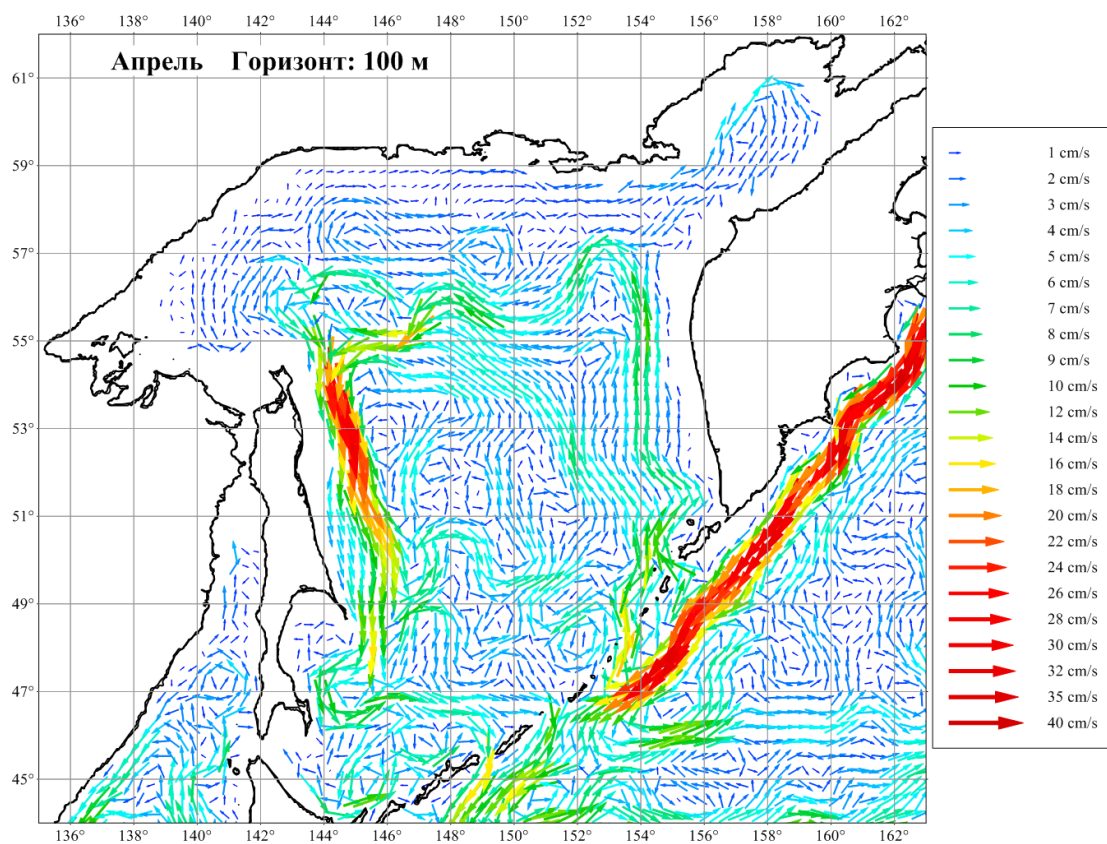
Рисунок 3.23. Течения Охотского моря в апреле на горизонте 100 м
