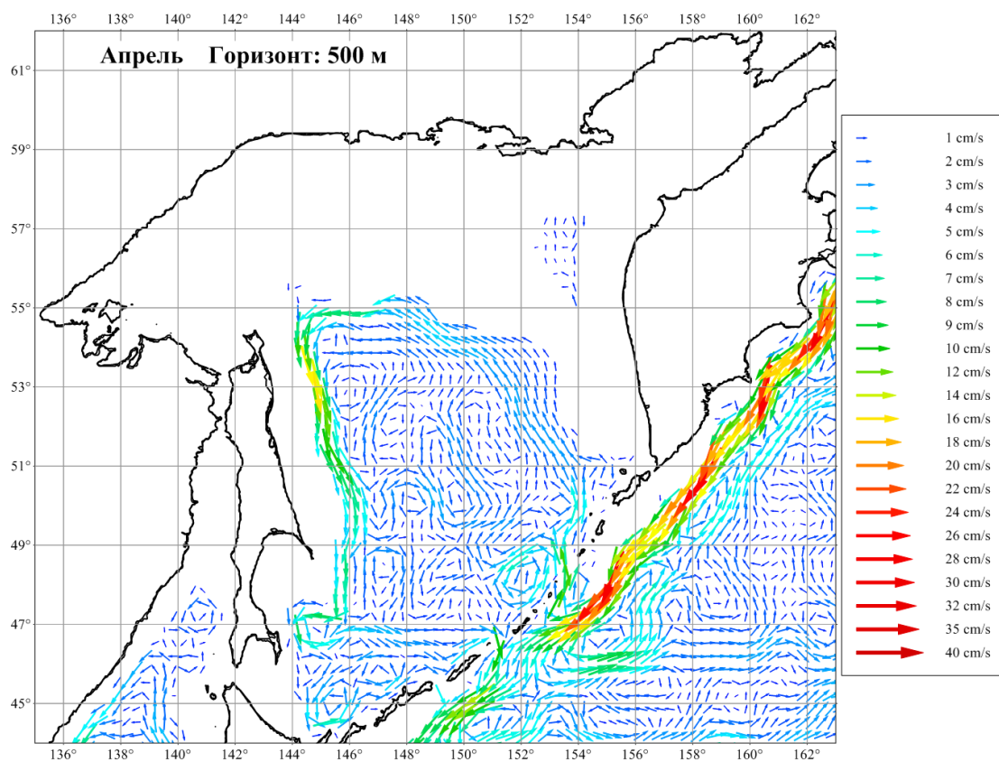
Рисунок 3.25. Течения Охотского моря в апреле на горизонте 500 м
