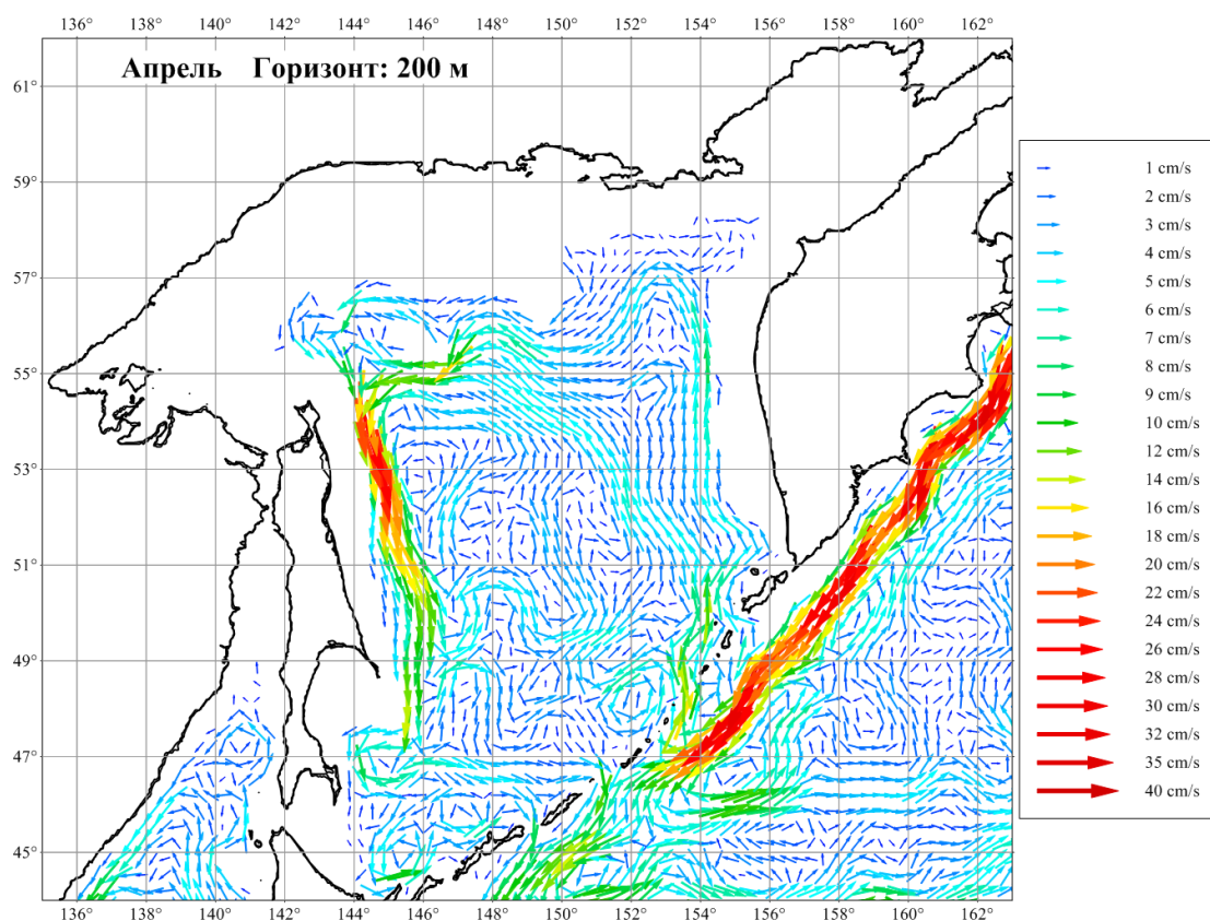
Рисунок 3.24. Течения Охотского моря в апреле на горизонте 200 м
