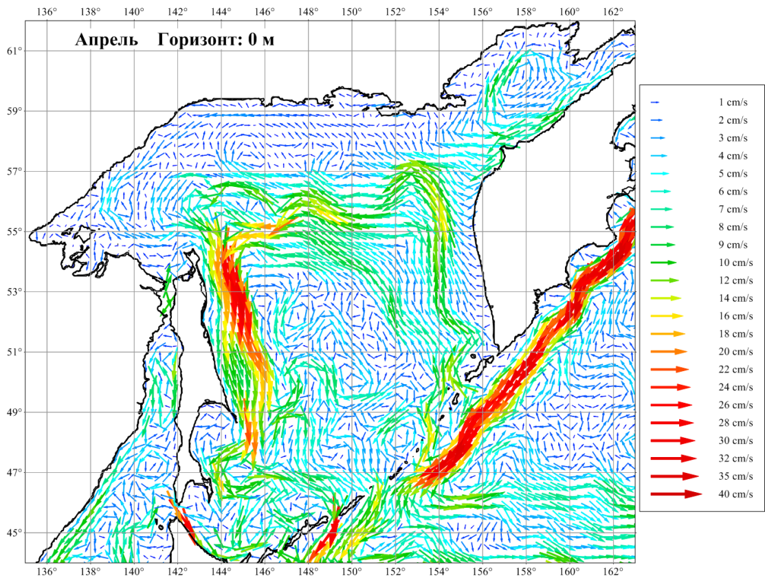
Рисунок 3.20. Течения Охотского моря в апреле на горизонте 0 м
