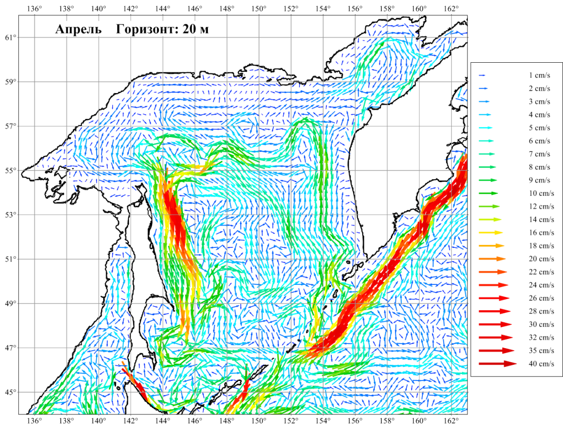
Рисунок 3.21. Течения Охотского моря в апреле на горизонте 20 м
