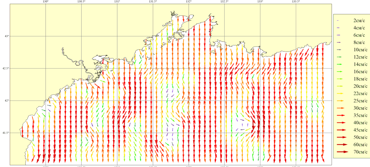
Рисунок 168. Месяц: Июль; Горизонт: 0м; Ветер: Северо-Западный умеренный (8 м/сек)
