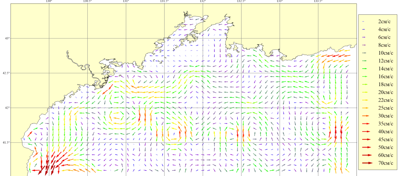
Рисунок 177. Месяц: Август; Горизонт: 0м; Ветер: Штиль
