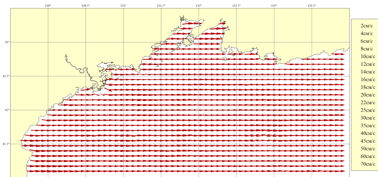
Рисунок 170. Месяц: Июль; Горизонт: 0м; Ветер: Юго-Западный сильный (16 м/сек)
