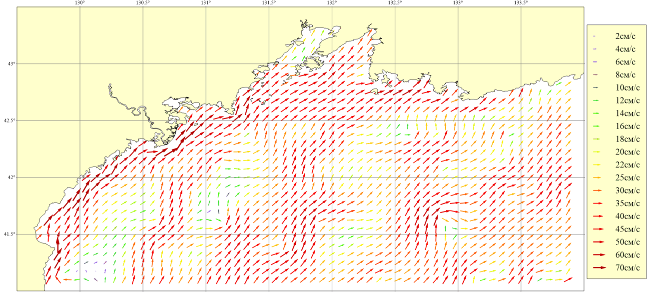
Рисунок 163. Месяц: Июль; Горизонт: 0м; Ветер: Южный умеренный (8 м/сек)
