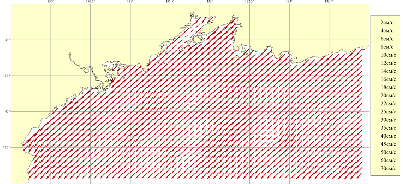
Рисунок 175. Месяц: Июль; Горизонт: 0м; Ветер: Северный сильный (16 м/сек)
