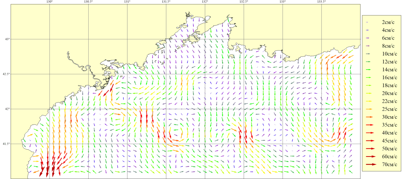
Рисунок 178. Месяц: Август; Горизонт: 0м; Ветер: Западный слабый (4 м/сек)
