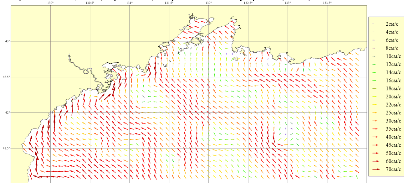
Рисунок 165. Месяц: Июль; Горизонт: 0м; Ветер: Восточный умеренный (8 м/сек)
