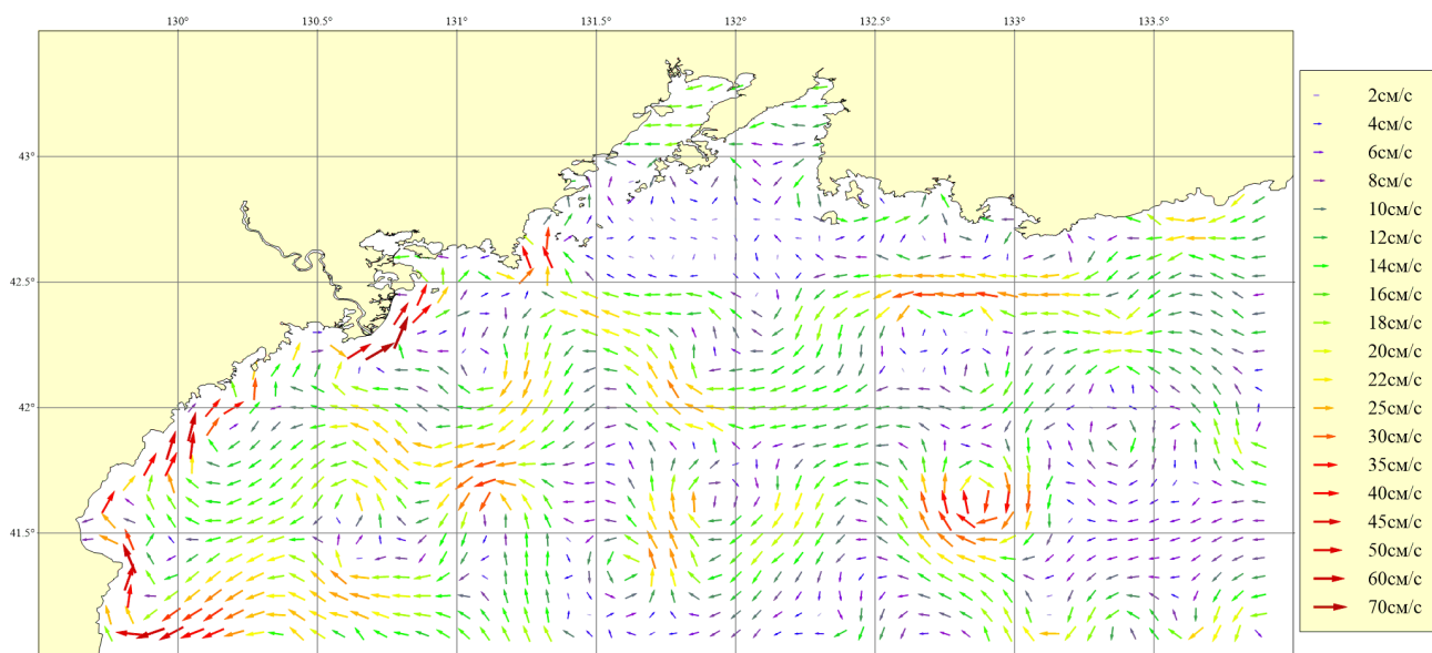
Рисунок 158. Месяц: Июль; Горизонт: 0м; Ветер: Северо-Восточный слабый (4 м/сек)
