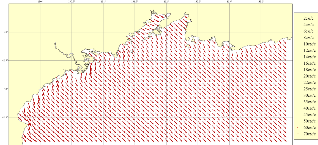
Рисунок 169. Месяц: Июль; Горизонт: 0м; Ветер: Западный сильный (16 м/сек)
