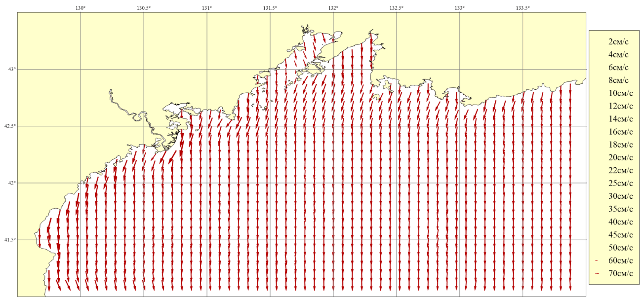
Рисунок 176. Месяц: Июль; Горизонт: 0м; Ветер: Северо-Западный сильный (16 м/сек)
