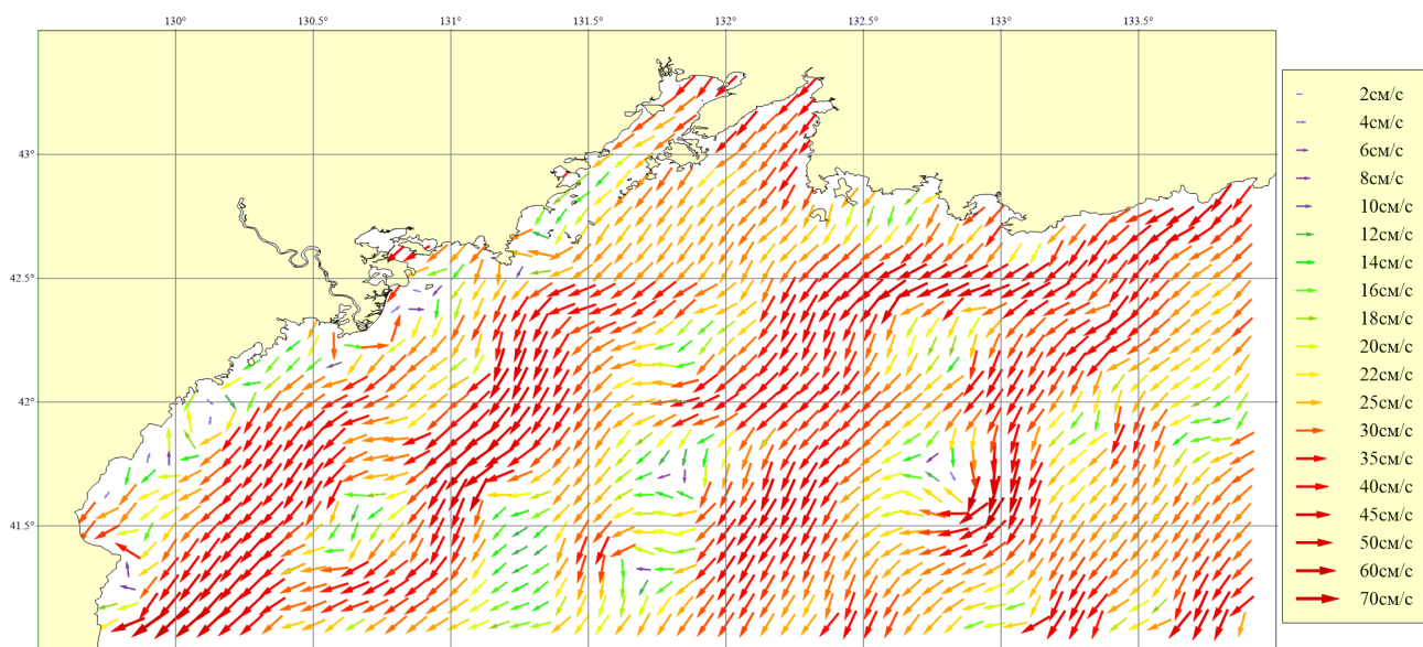
Рисунок 167. Месяц: Июль; Горизонт: 0м; Ветер: Северный умеренный (8 м/сек)
