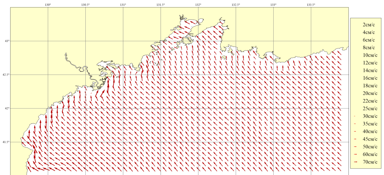
Рисунок 173. Месяц: Июль; Горизонт: 0м; Ветер: Восточный сильный (16 м/сек)
