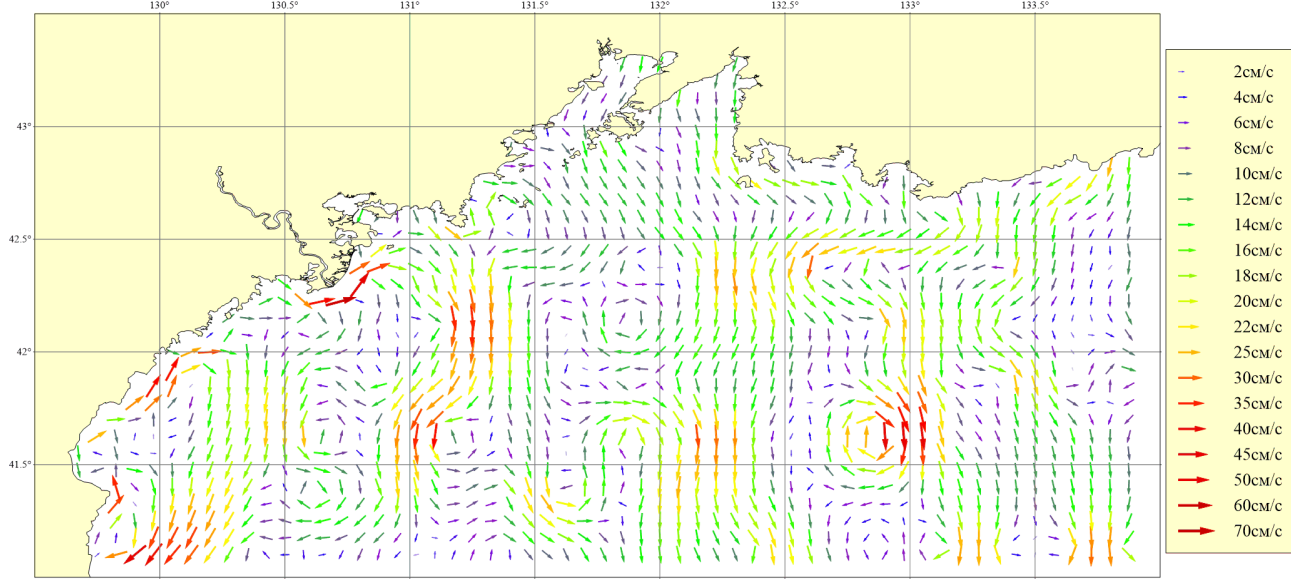
Рисунок 160. Месяц: Июль; Горизонт: 0м; Ветер: Северо-Западный слабый (4 м/сек)
