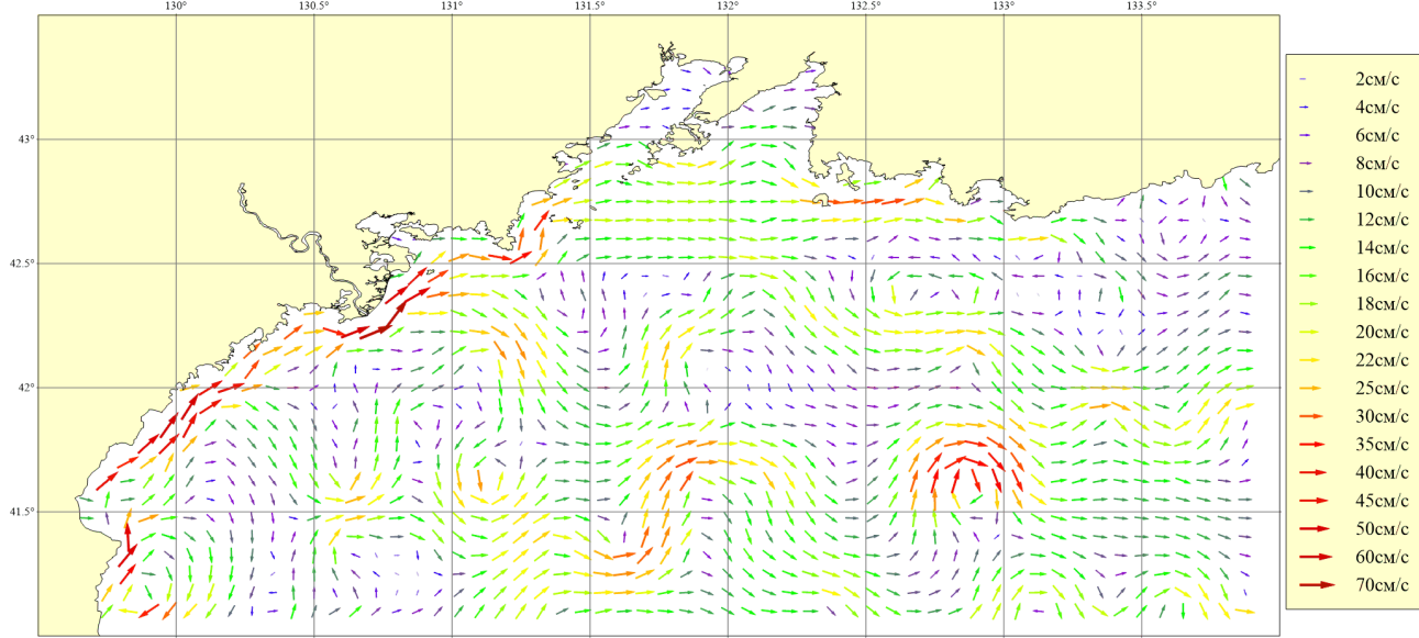
Рисунок 154. Месяц: Июль; Горизонт: 0м; Ветер: Юго-Западный слабый (4 м/сек)
