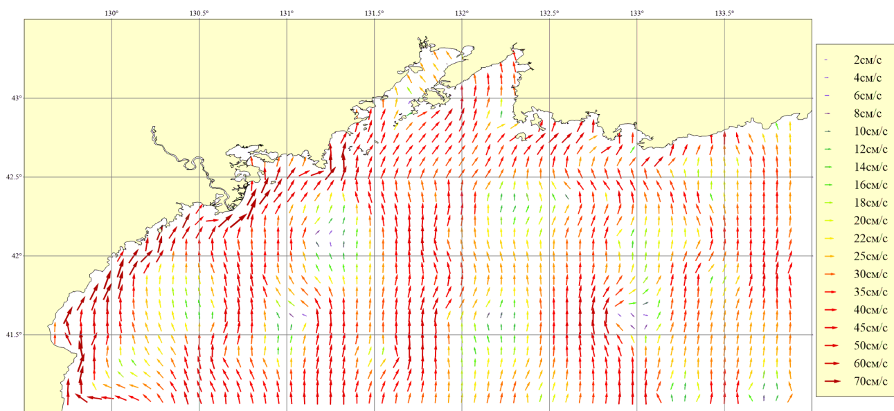
Рисунок 164. Месяц: Июль; Горизонт: 0м; Ветер: Юго-Восточный умеренный (8 м/сек)
