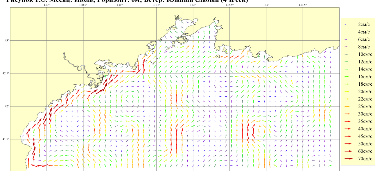
Рисунок 156. Месяц: Июль; Горизонт: 0м; Ветер: Юго-Восточный слабый (4 м/сек)
