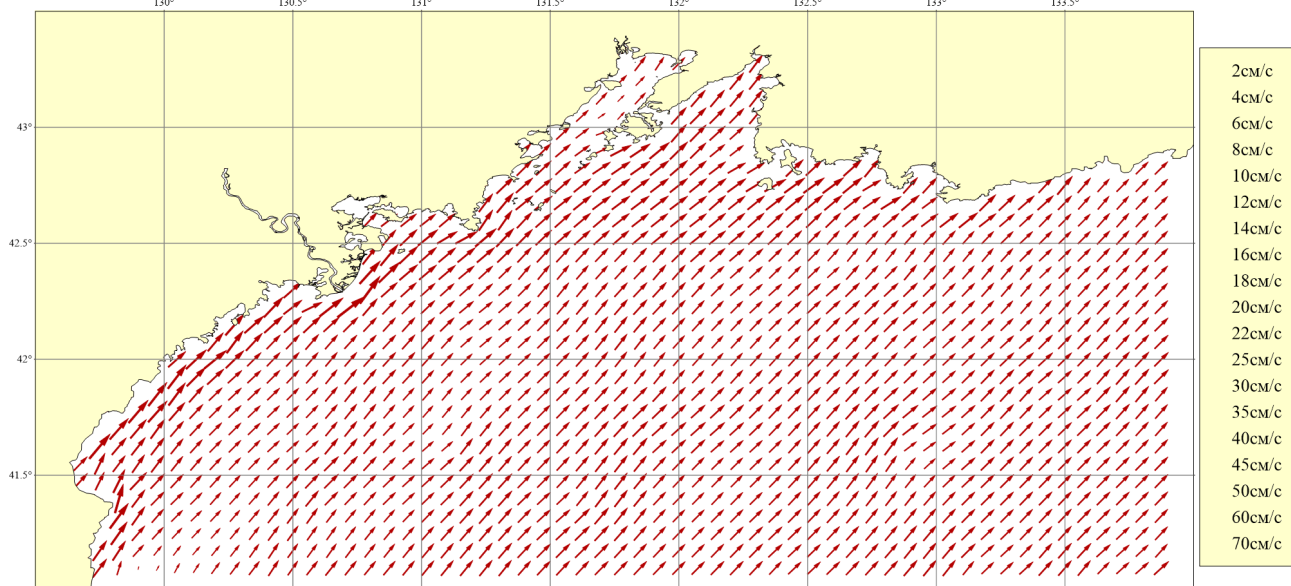
Рисунок 171. Месяц: Июль; Горизонт: 0м; Ветер: Южный сильный (16 м/сек)
