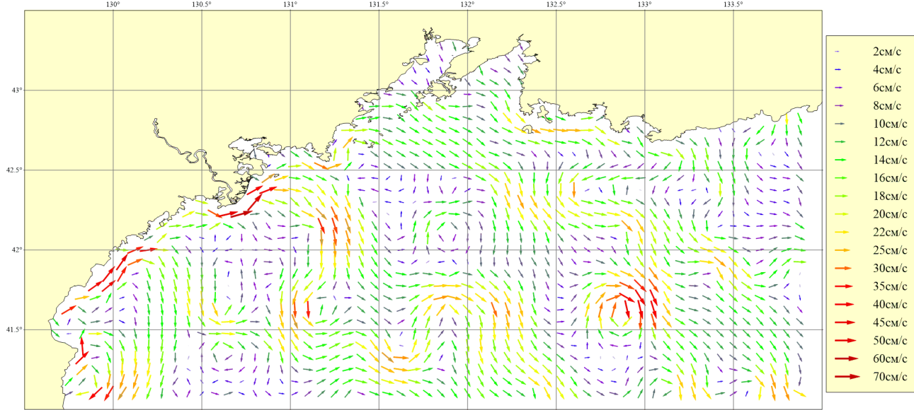
Рисунок 153. Месяц: Июль; Горизонт: 0м; Ветер: Западный слабый (4 м/сек)
