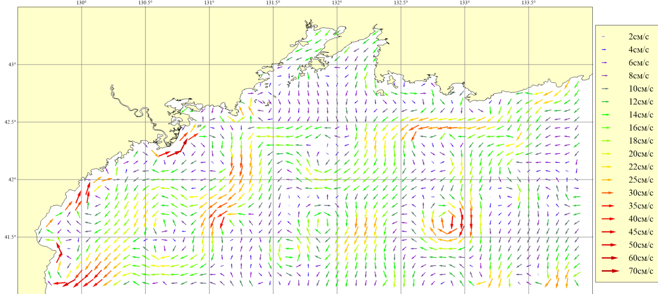
Рисунок 159. Месяц: Июль; Горизонт: 0м; Ветер: Северный слабый (4 м/сек)
