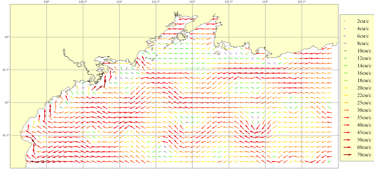
Рисунок 166. Месяц: Июль; Горизонт: 0м; Ветер: Северо-Восточный умеренный (8 м/сек)
