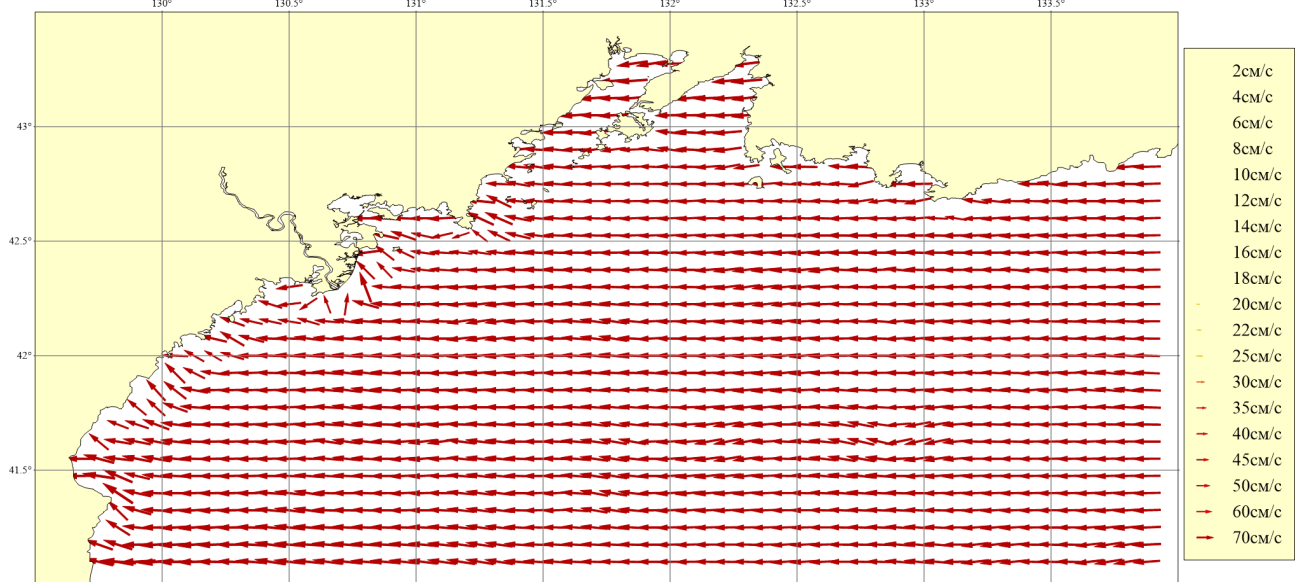
Рисунок 174. Месяц: Июль; Горизонт: 0м; Ветер: Северо-Восточный сильный (16 м/сек)
