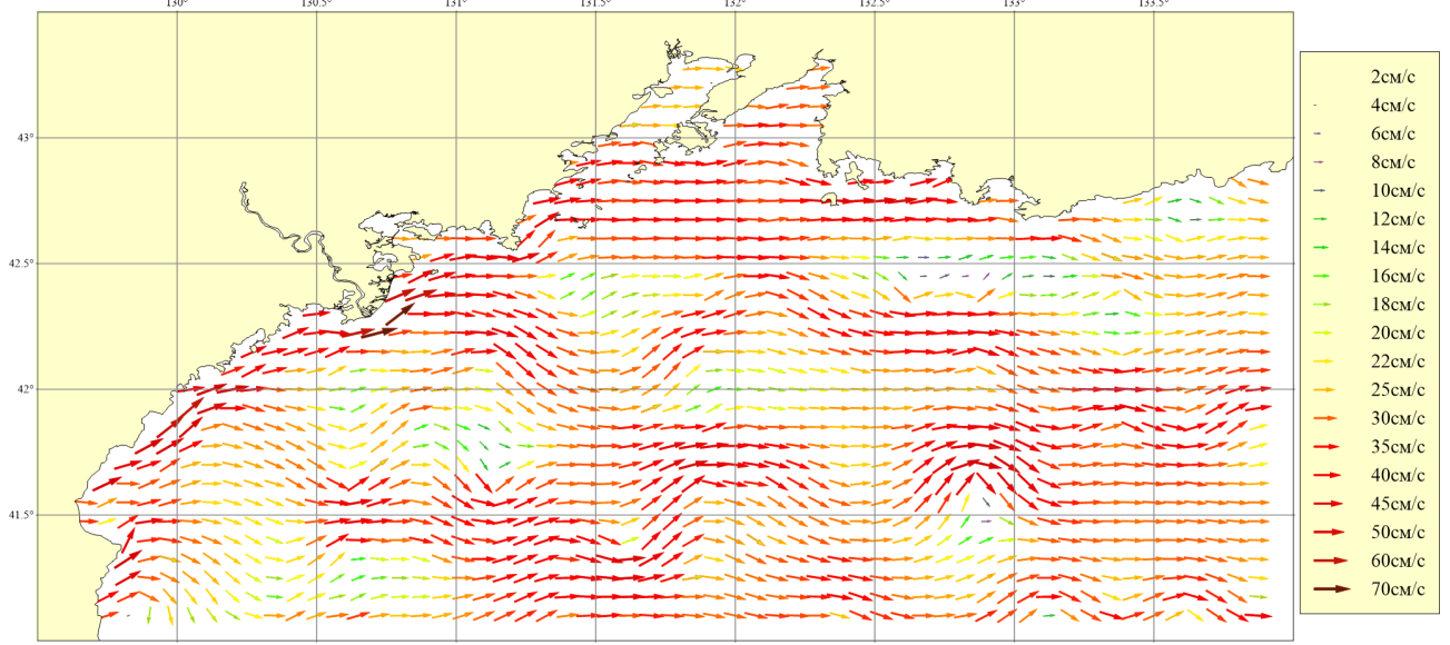
Рисунок 162. Месяц: Июль; Горизонт: 0м; Ветер: Юго-Западный умеренный (8 м/сек)
