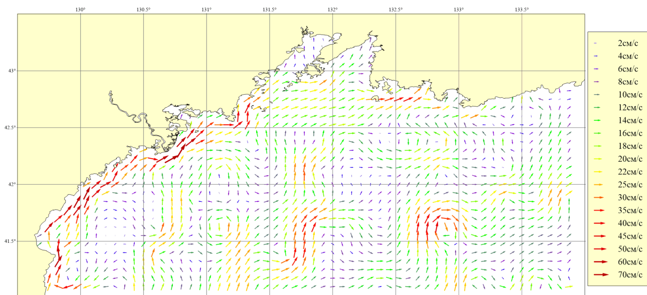
Рисунок 155. Месяц: Июль; Горизонт: 0м; Ветер: Южный слабый (4 м/сек)
