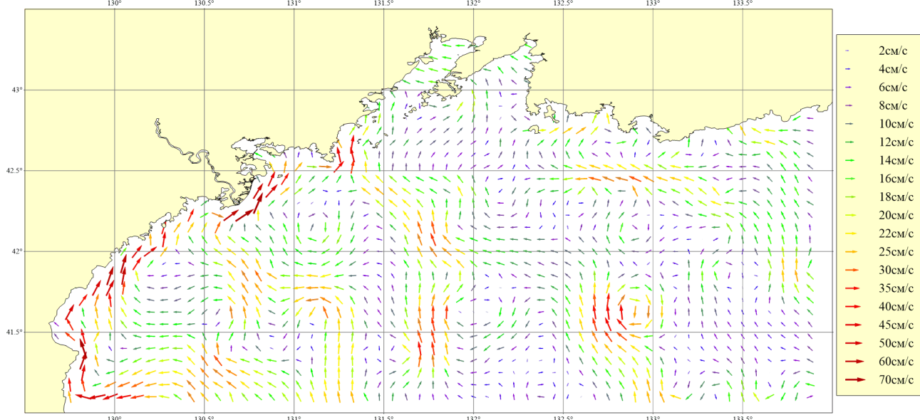
Рисунок 157. Месяц: Июль; Горизонт: 0м; Ветер: Восточный слабый (4 м/сек)
