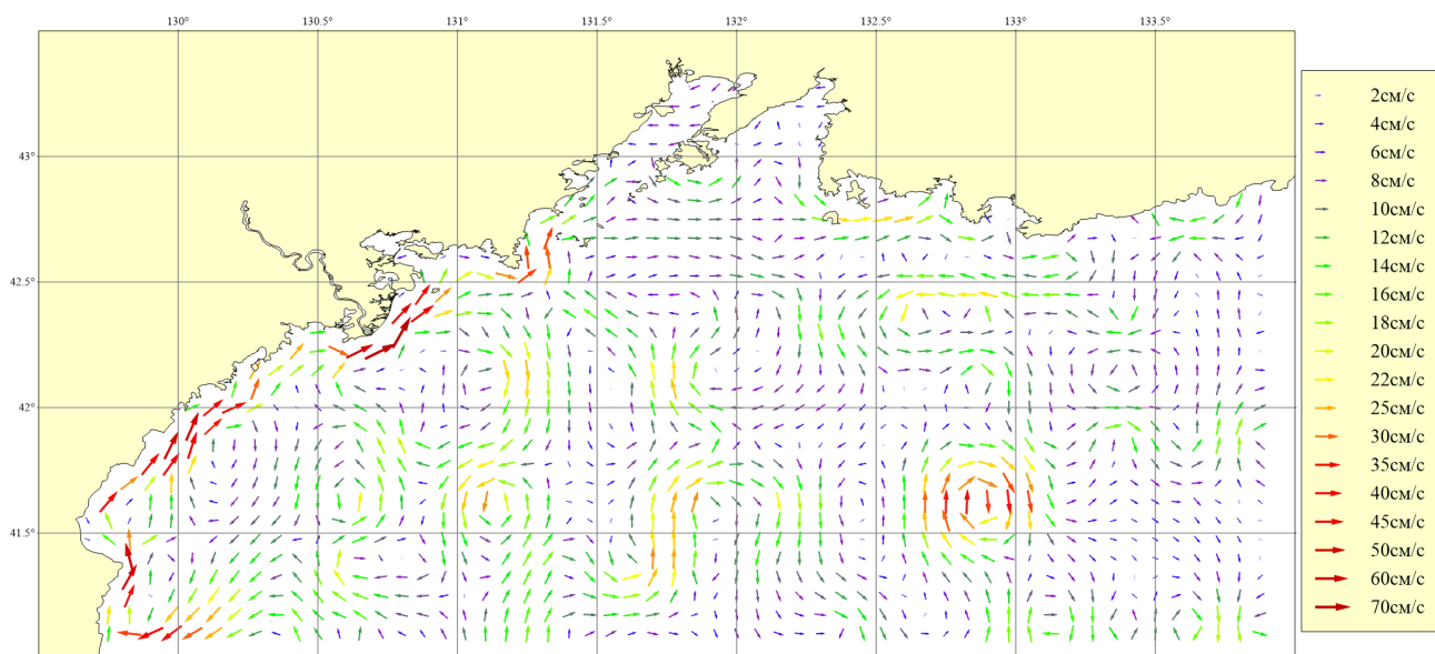
Рисунок 152. Месяц: Июль; Горизонт: 0м; Ветер: Штиль
