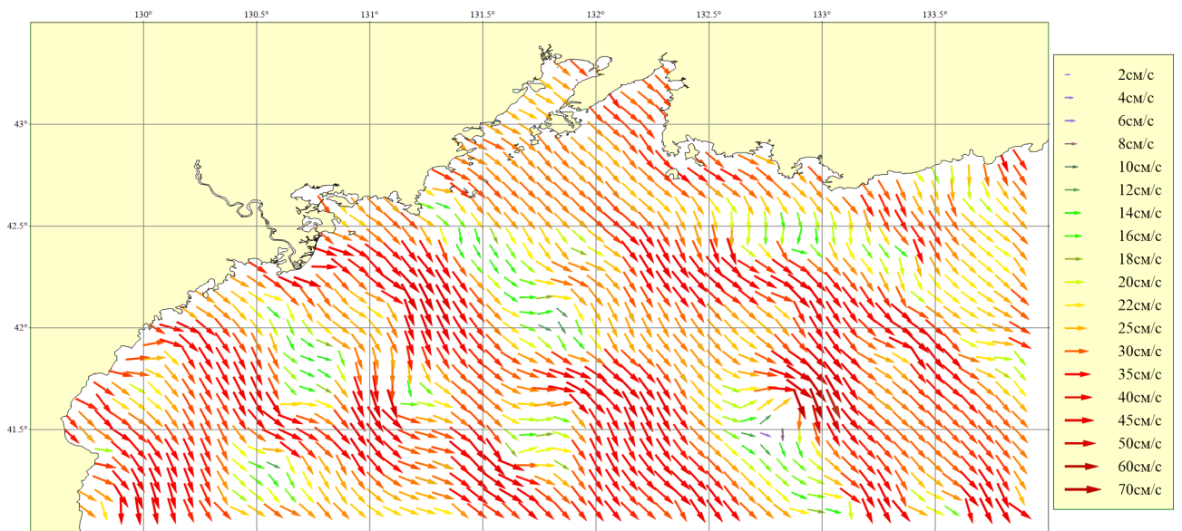
Рисунок 161. Месяц: Июль; Горизонт: 0м; Ветер: Западный умеренный (8 м/сек)
