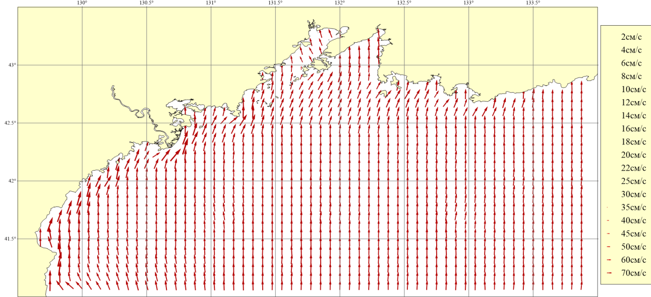
Рисунок 172. Месяц: Июль; Горизонт: 0м; Ветер: Юго-Восточный сильный (16 м/сек)
