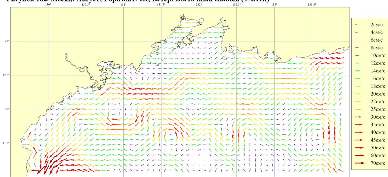
Рисунок 183. Месяц: Август; Горизонт: 0м; Ветер: Северо-Восточный слабый (4 м/сек)
