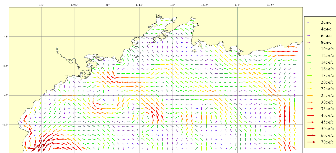
Рисунок 182. Месяц: Август; Горизонт: 0м; Ветер: Восточный слабый (4 м/сек)
