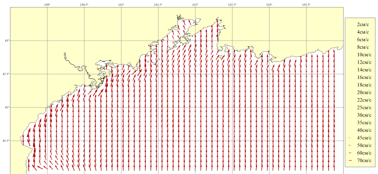
Рисунок 197. Месяц: Август; Горизонт: 0м; Ветер: Юго-Восточный сильный (16 м/сек)
