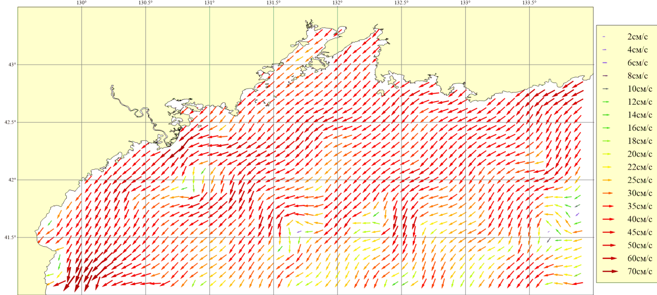
Рисунок 192. Месяц: Август; Горизонт: 0м; Ветер: Северный умеренный (8 м/сек)
