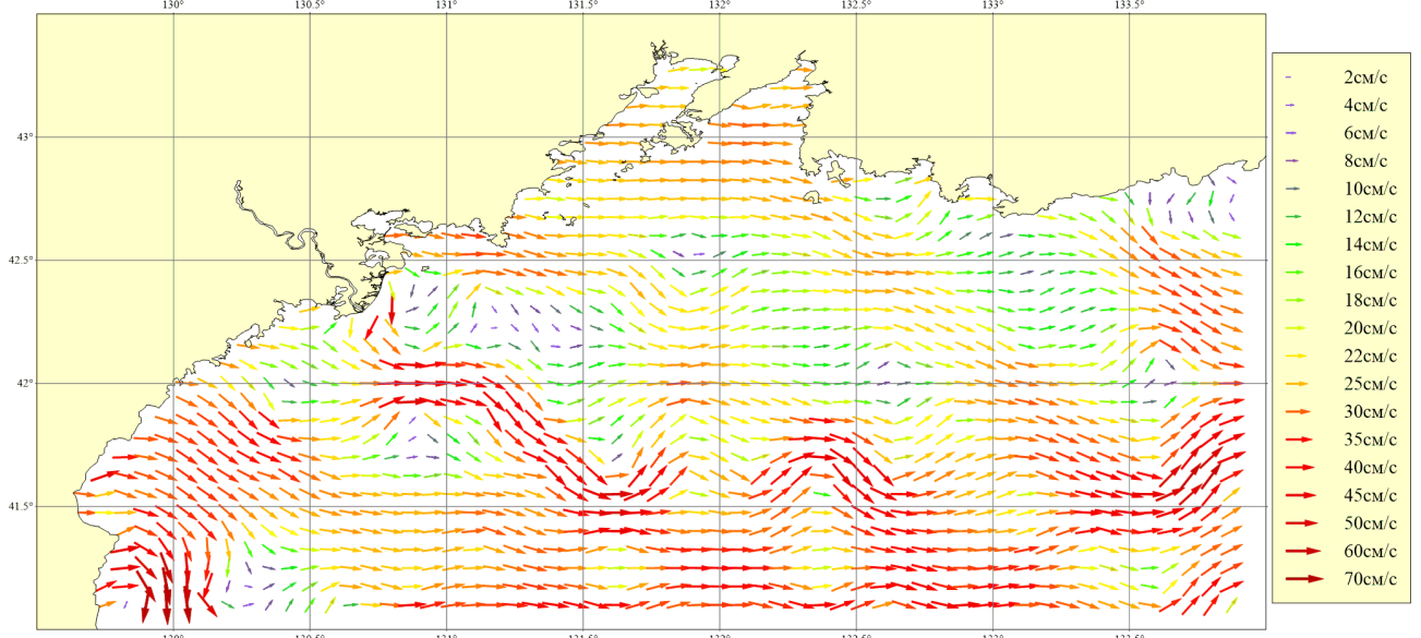
Рисунок 187. Месяц: Август; Горизонт: 0м; Ветер: Юго-Западный умеренный (8 м/сек)
