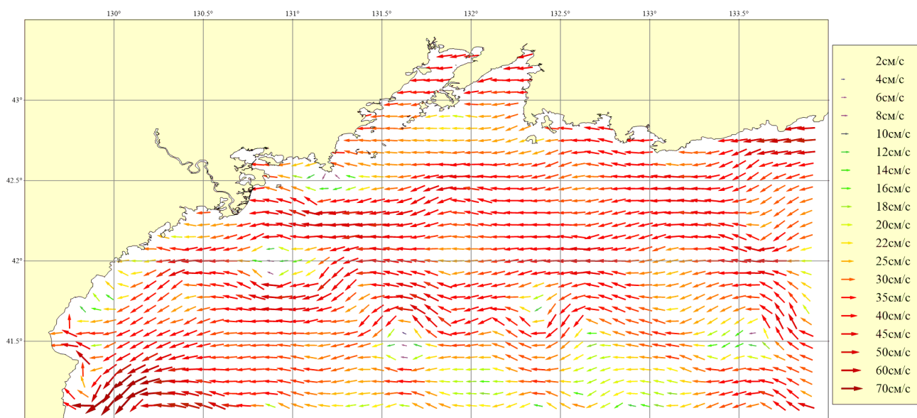
Рисунок 191. Месяц: Август; Горизонт: 0м; Ветер: Северо-Восточный умеренный (8 м/сек)
