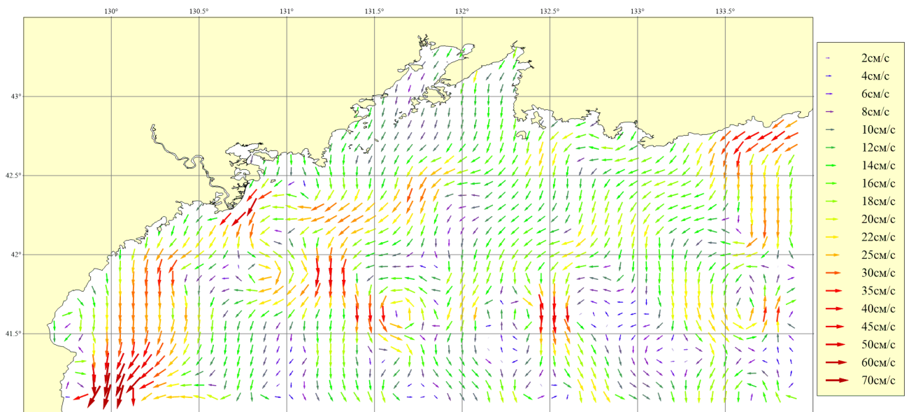
Рисунок 185. Месяц: Август; Горизонт: 0м; Ветер: Северо-Западный слабый (4 м/сек)
