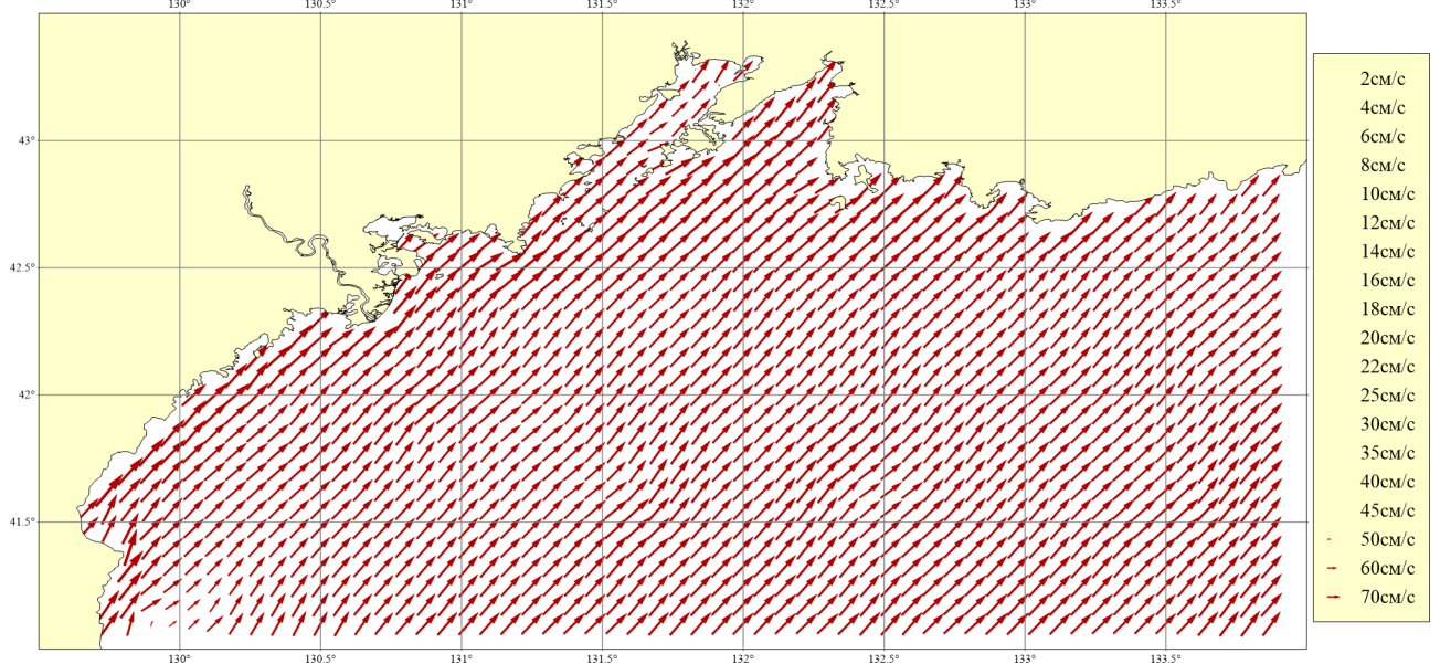
Рисунок 196. Месяц: Август; Горизонт: 0м; Ветер: Южный сильный (16 м/сек)
