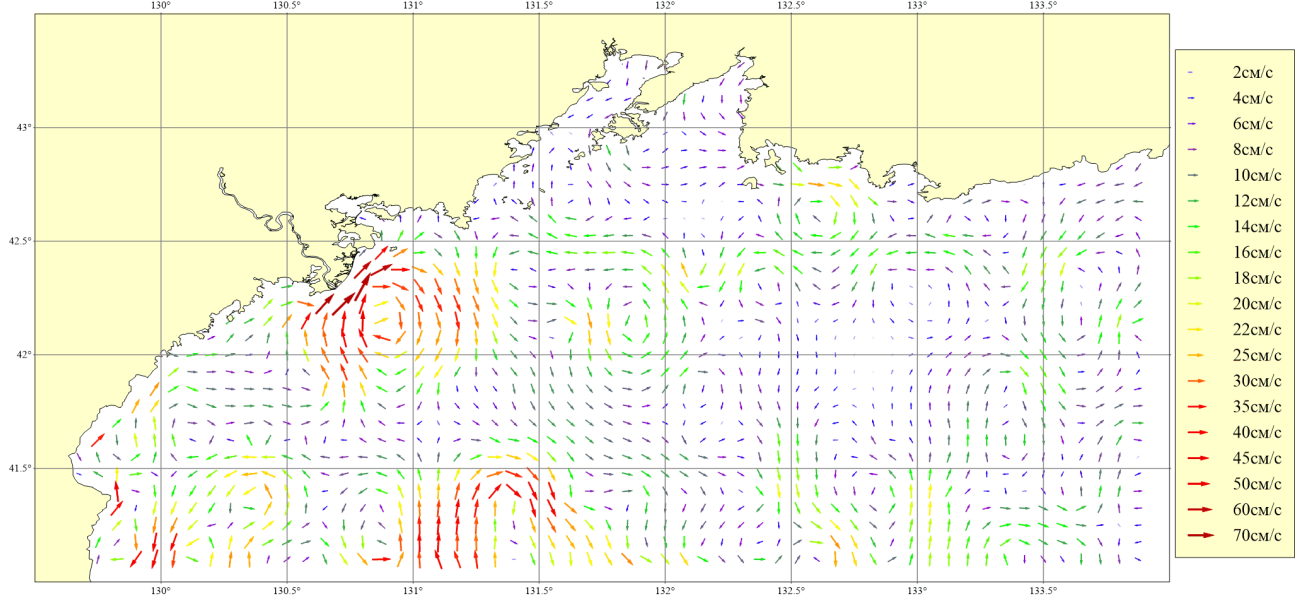
Рисунок 202. Месяц: Сентябрь; Горизонт: 0м; Ветер: Штиль
