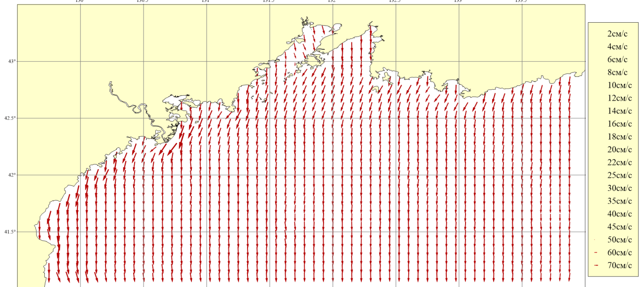
Рисунок 201. Месяц: Август; Горизонт: 0м; Ветер: Северо-Западный сильный (16 м/сек)
