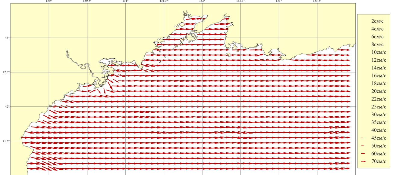
Рисунок 195. Месяц: Август; Горизонт: 0м; Ветер: Юго-Западный сильный (16 м/сек)
