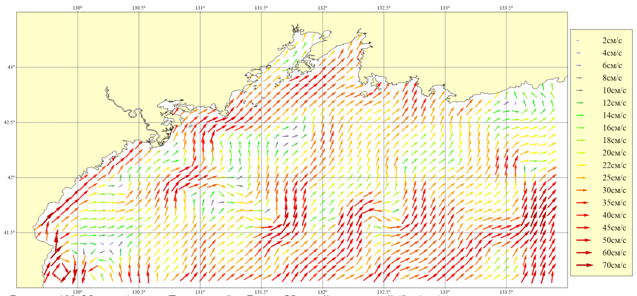
Рисунок 188. Месяц: Август; Горизонт: 0м; Ветер: Южный умеренный (8 м/сек)
