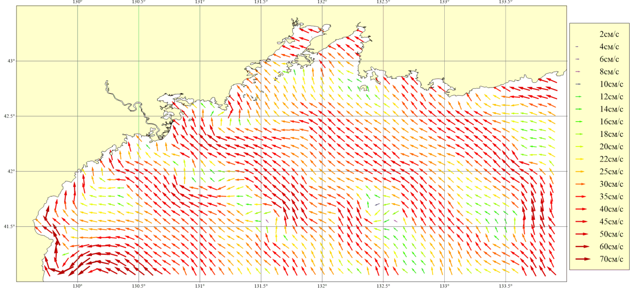
Рисунок 190. Месяц: Август; Горизонт: 0м; Ветер: Восточный умеренный (8 м/сек)
