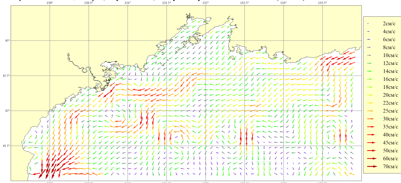
Рисунок 184. Месяц: Август; Горизонт: 0м; Ветер: Северный слабый (4 м/сек)
