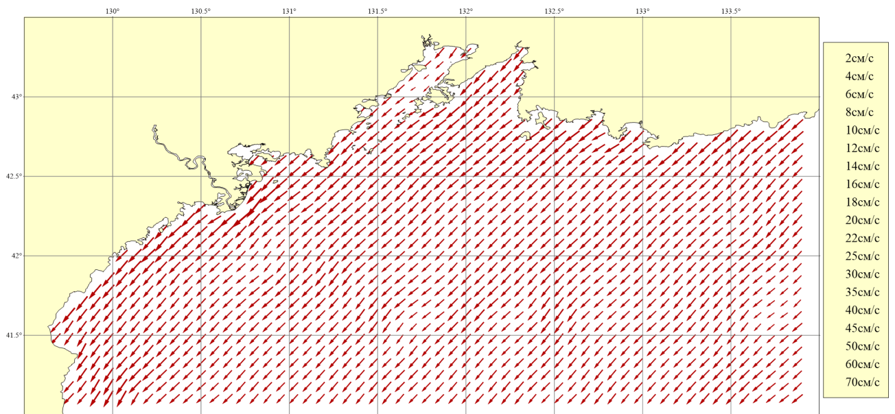
Рисунок 200. Месяц: Август; Горизонт: 0м; Ветер: Северный сильный (16 м/сек)
