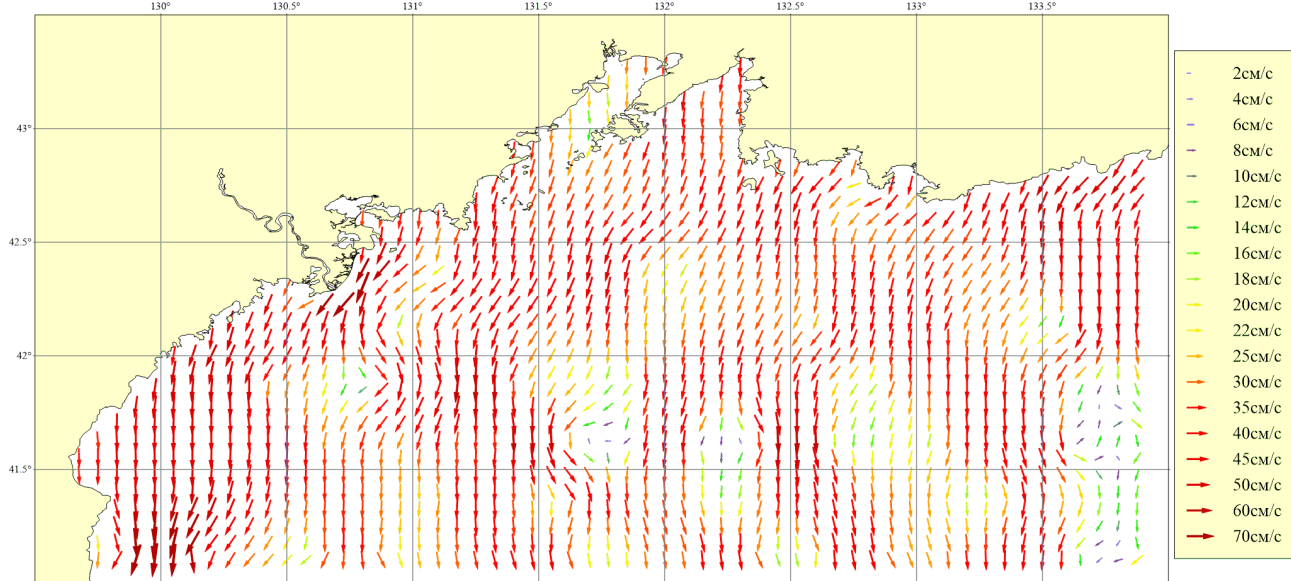
Рисунок 193. Месяц: Август; Горизонт: 0м; Ветер: Северо-Западный умеренный (8 м/сек)
