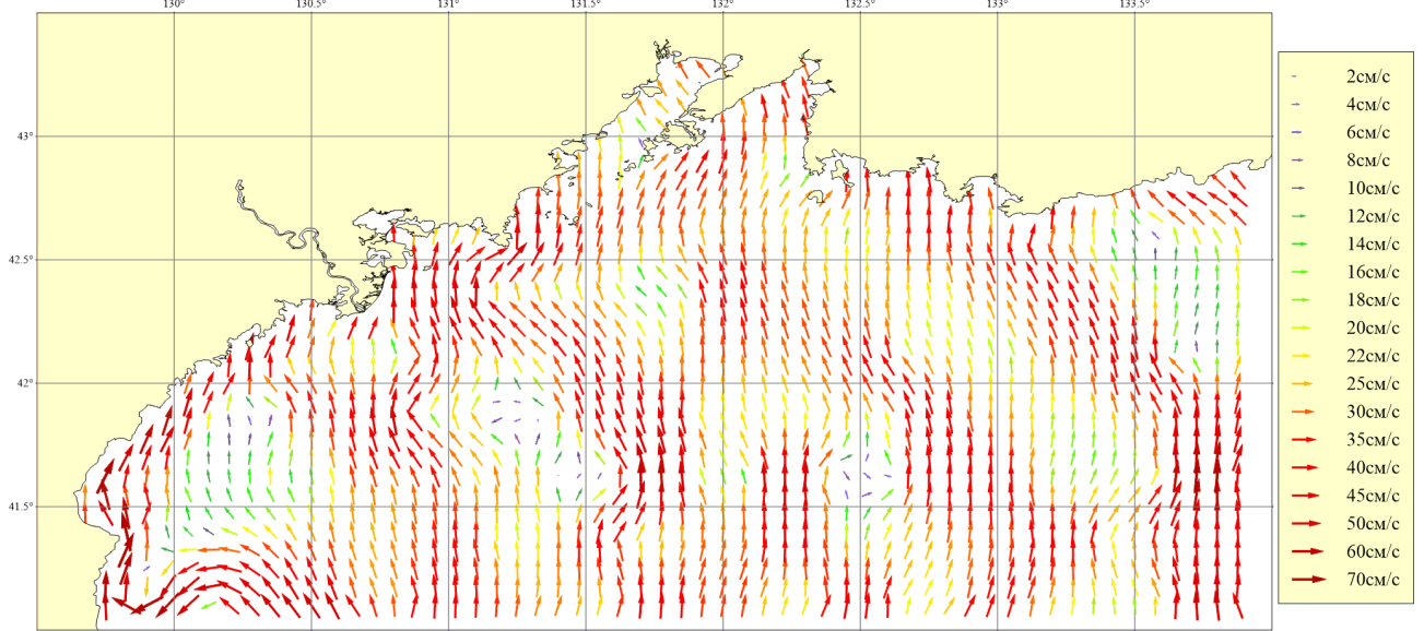
Рисунок 189. Месяц: Август; Горизонт: 0м; Ветер: Юго-Восточный умеренный (8 м/сек)
