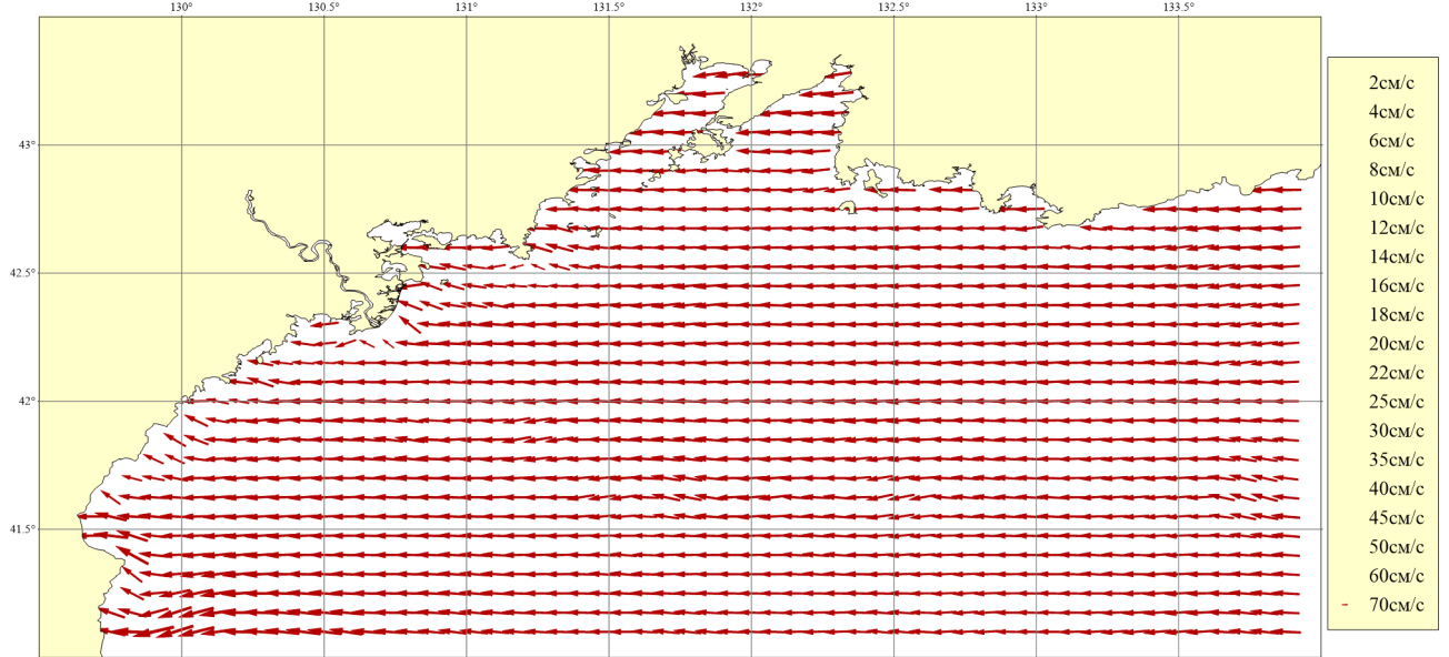
Рисунок 199. Месяц: Август; Горизонт: 0м; Ветер: Северо-Восточный сильный (16 м/сек)
