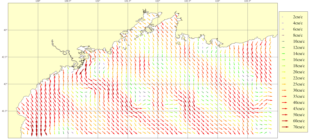
Рисунок 186. Месяц: Август; Горизонт: 0м; Ветер: Западный умеренный (8 м/сек)
