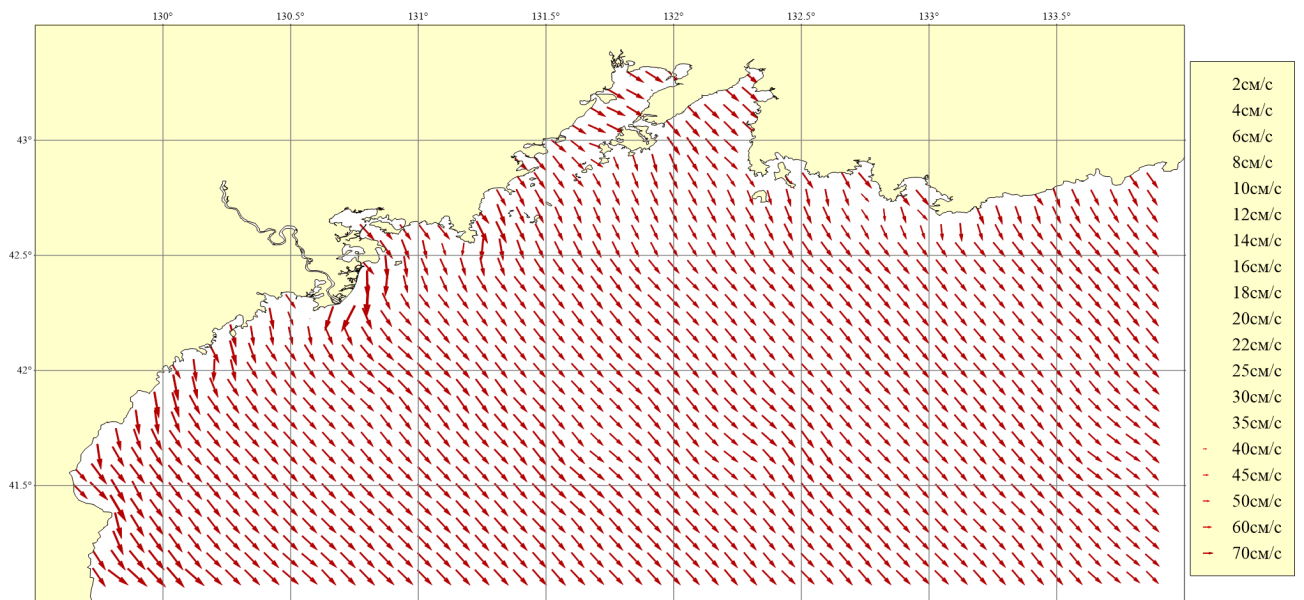
Рисунок 194. Месяц: Август; Горизонт: 0м; Ветер: Западный сильный (16 м/сек)
