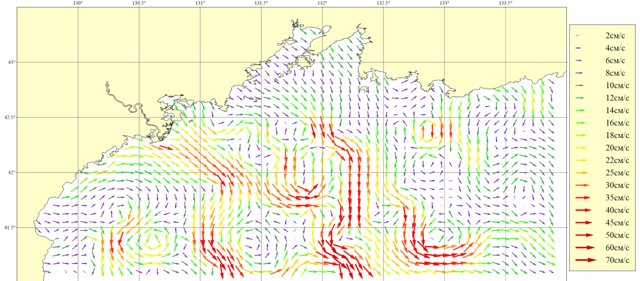
Рисунок 253. Месяц: Ноябрь; Горизонт: 0м; Ветер: Западный слабый (4 м/сек)
