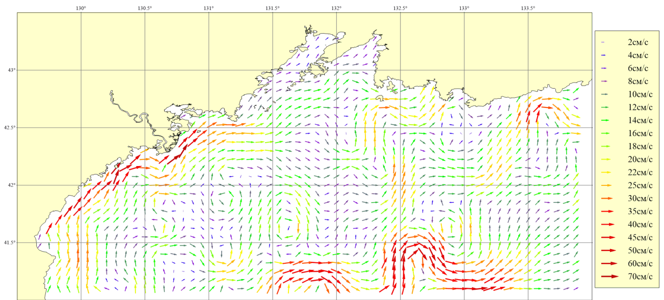
Рисунок 230. Месяц: Октябрь; Горизонт: 0м; Ветер: Южный слабый (4 м/сек)
