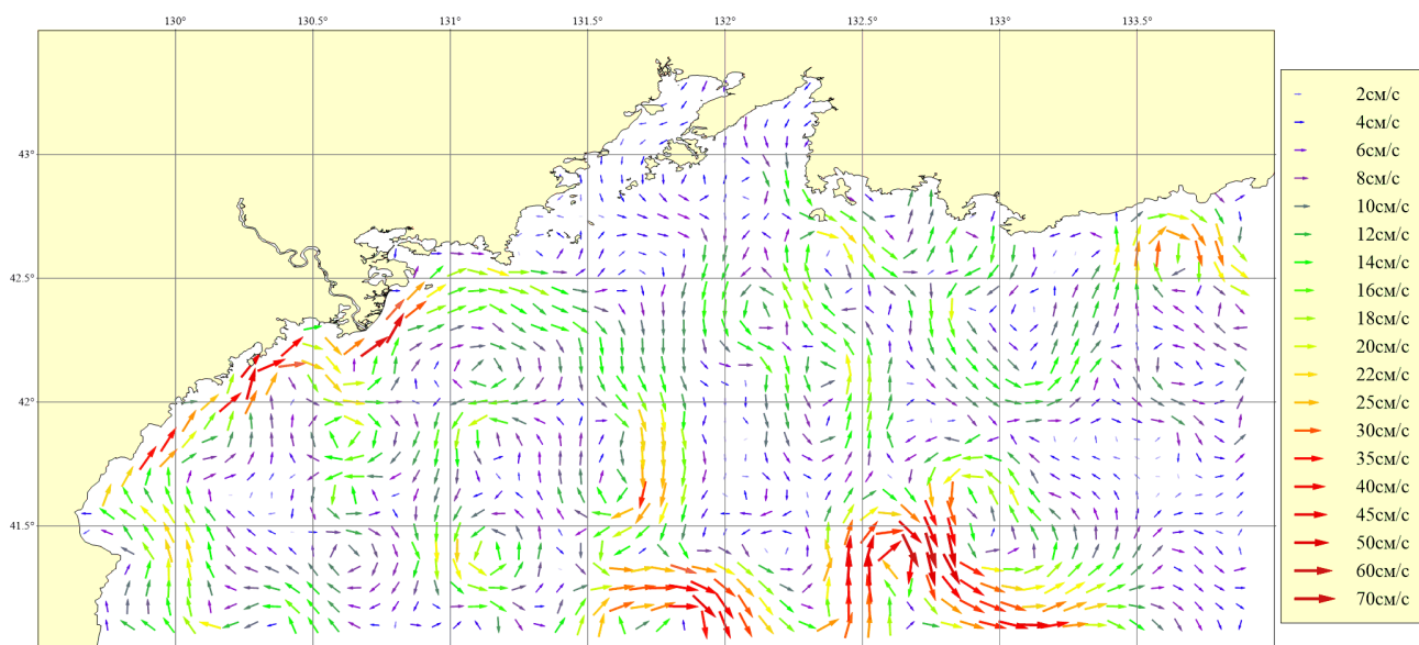
Рисунок 227. Месяц: Октябрь; Горизонт: 0м; Ветер: Штиль
