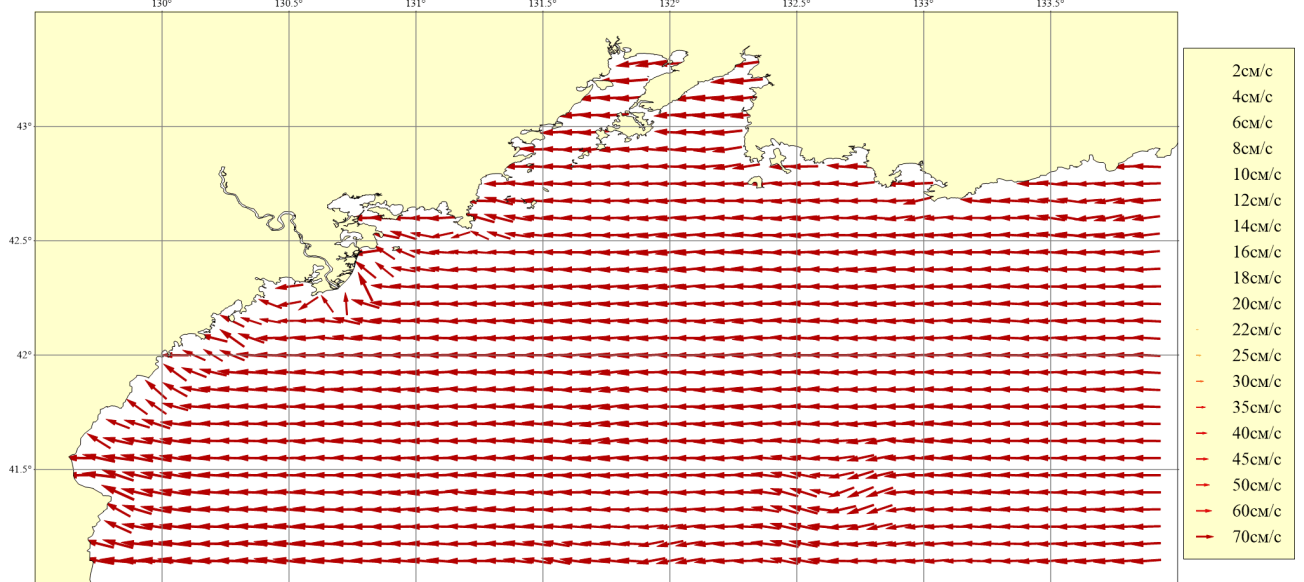
Рисунок 249. Месяц: Октябрь; Горизонт: 0м; Ветер: Северо-Восточный сильный (16 м/сек)
