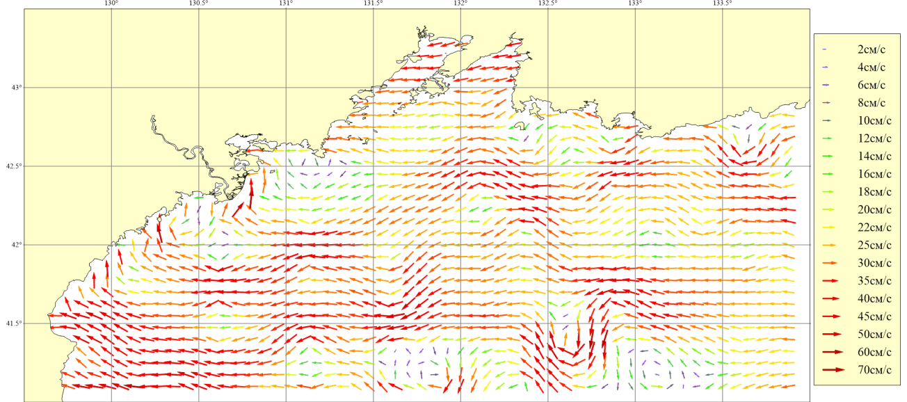
Рисунок 241. Месяц: Октябрь; Горизонт: 0м; Ветер: Северо-Восточный умеренный (8 м/сек)
