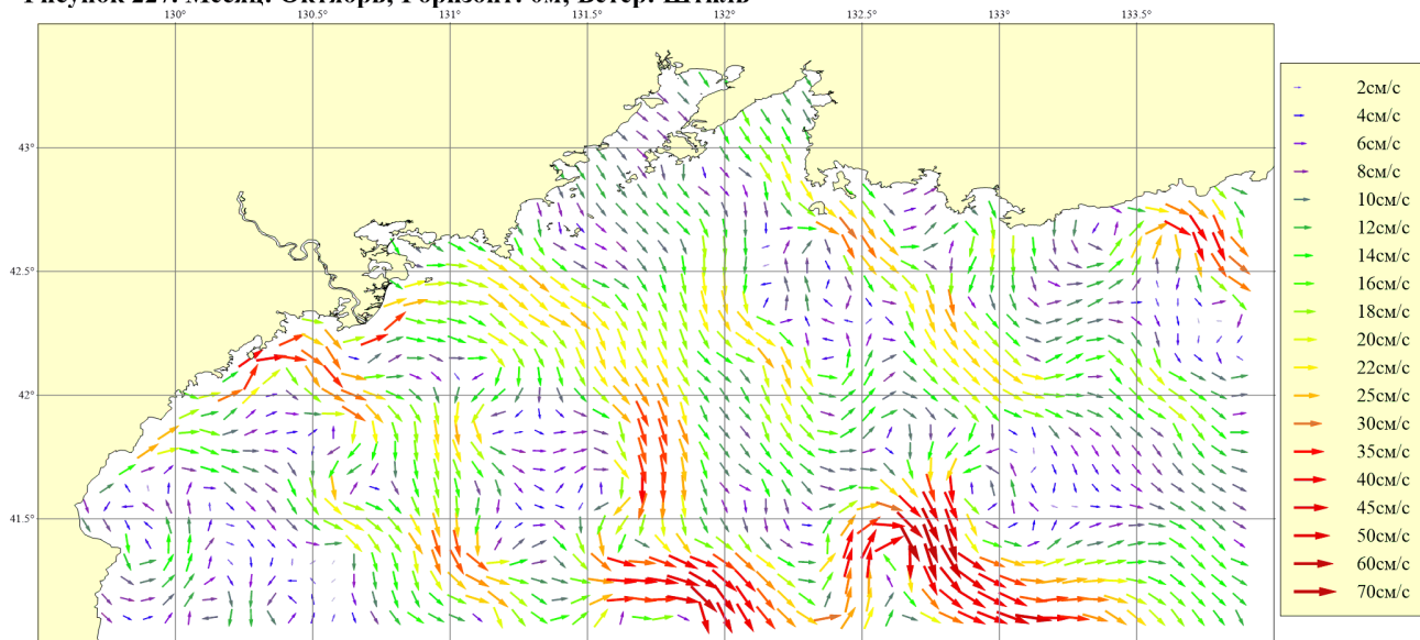
Рисунок 228. Месяц: Октябрь; Горизонт: 0м; Ветер: Западный слабый (4 м/сек)
