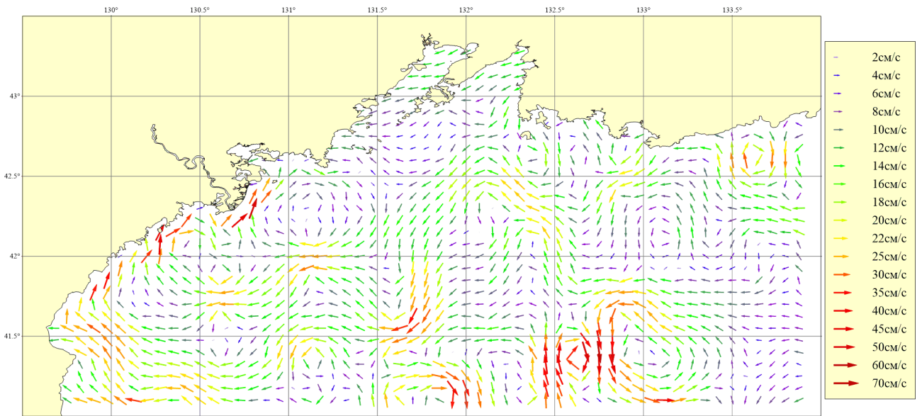
Рисунок 233. Месяц: Октябрь; Горизонт: 0м; Ветер: Северо-Восточный слабый (4 м/сек)
