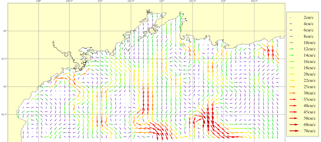
Рисунок 235. Месяц: Октябрь; Горизонт: 0м; Ветер: Северо-Западный слабый (4 м/сек)
