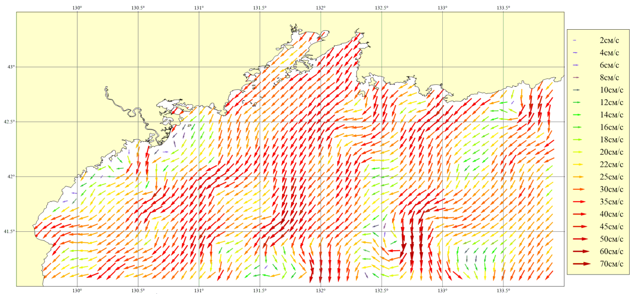
Рисунок 242. Месяц: Октябрь; Горизонт: 0м; Ветер: Северный умеренный (8 м/сек)
