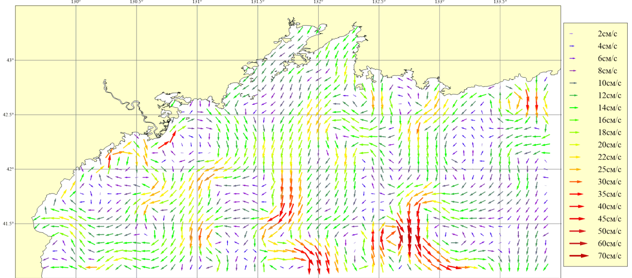
Рисунок 234. Месяц: Октябрь; Горизонт: 0м; Ветер: Северный слабый (4 м/сек)
