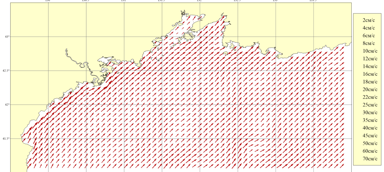
Рисунок 246. Месяц: Октябрь; Горизонт: 0м; Ветер: Южный сильный (16 м/сек)
