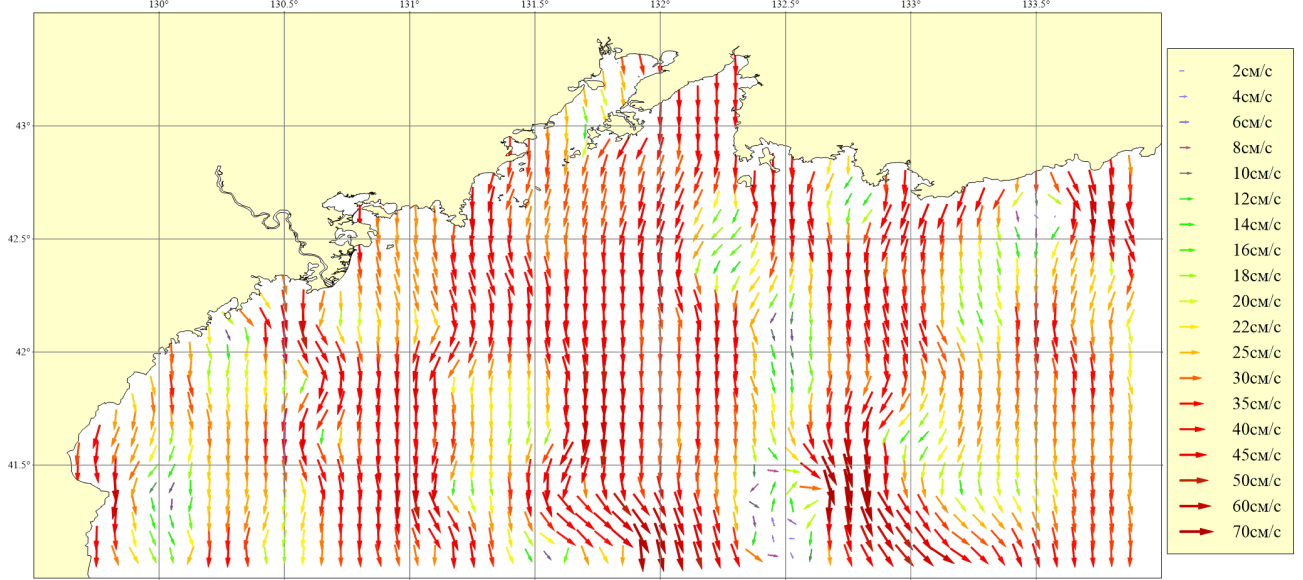
Рисунок 243. Месяц: Октябрь; Горизонт: 0м; Ветер: Северо-Западный умеренный (8 м/сек)
