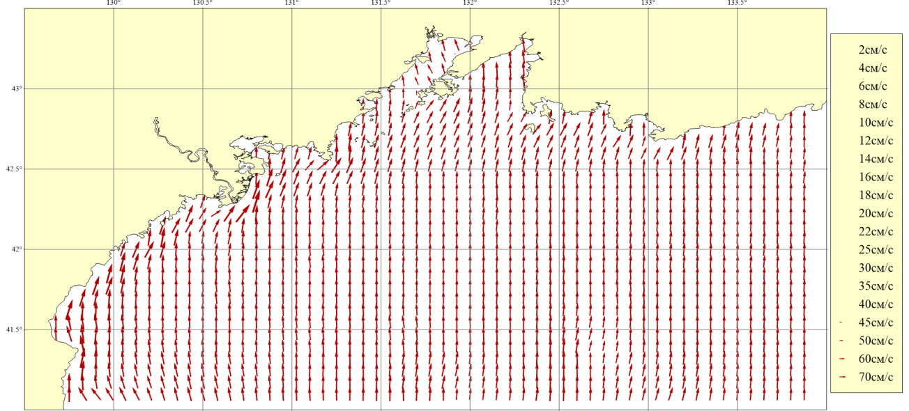
Рисунок 247. Месяц: Октябрь; Горизонт: 0м; Ветер: Юго-Восточный сильный (16 м/сек)
