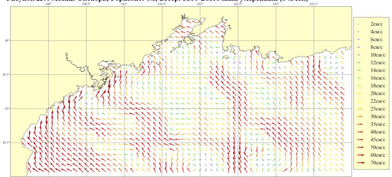
Рисунок 240. Месяц: Октябрь; Горизонт: 0м; Ветер: Восточный умеренный (8 м/сек)
