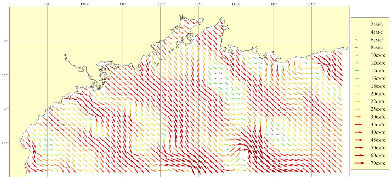
Рисунок 236. Месяц: Октябрь; Горизонт: 0м; Ветер: Западный умеренный (8 м/сек)
