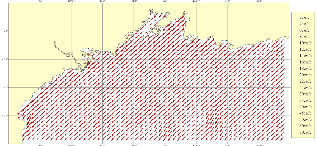
Рисунок 250. Месяц: Октябрь; Горизонт: 0м; Ветер: Северный сильный (16 м/сек)
