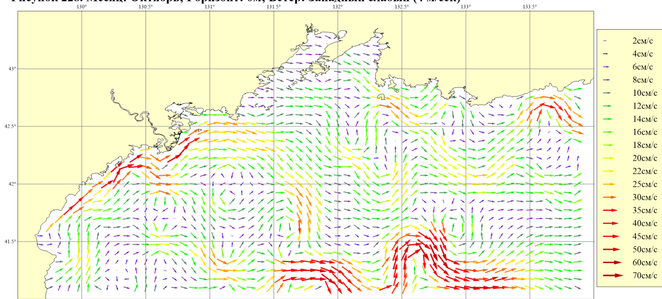
Рисунок 229. Месяц: Октябрь; Горизонт: 0м; Ветер: Юго-Западный слабый (4 м/сек)
