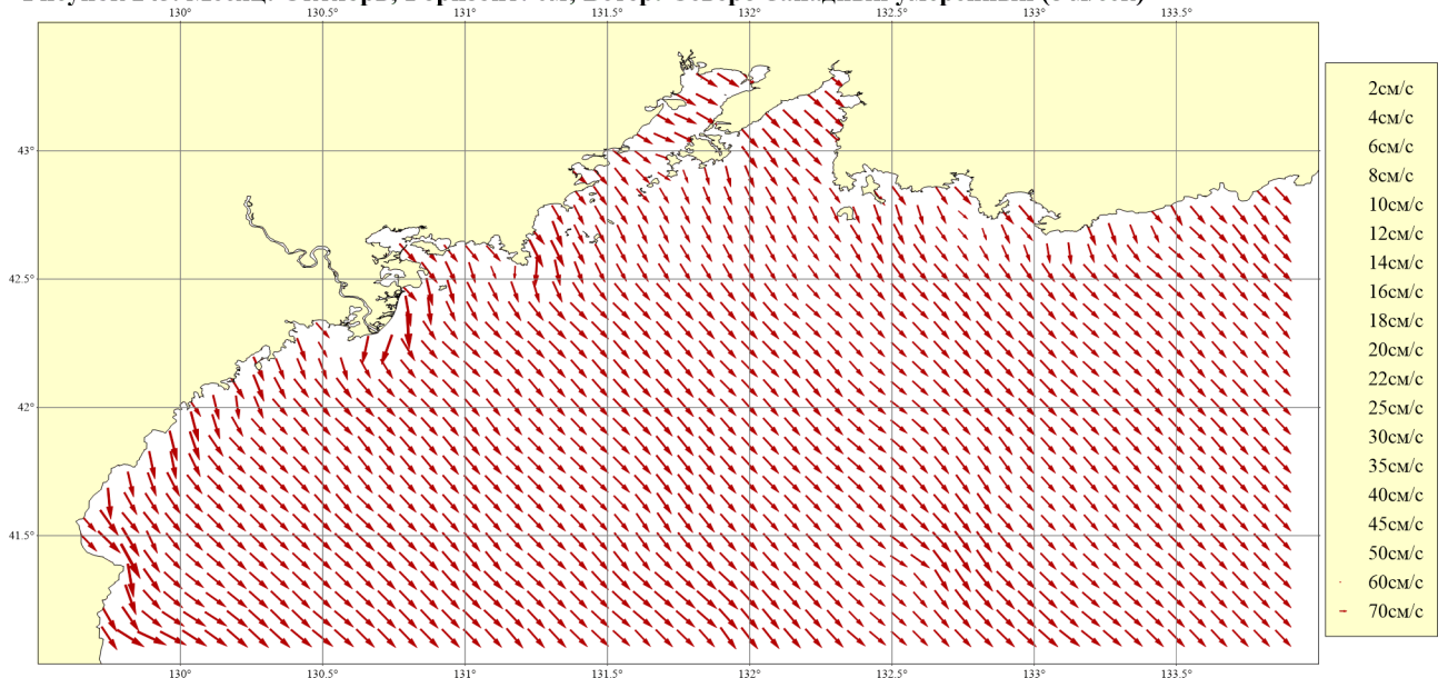
Рисунок 244. Месяц: Октябрь; Горизонт: 0м; Ветер: Западный сильный (16 м/сек)
