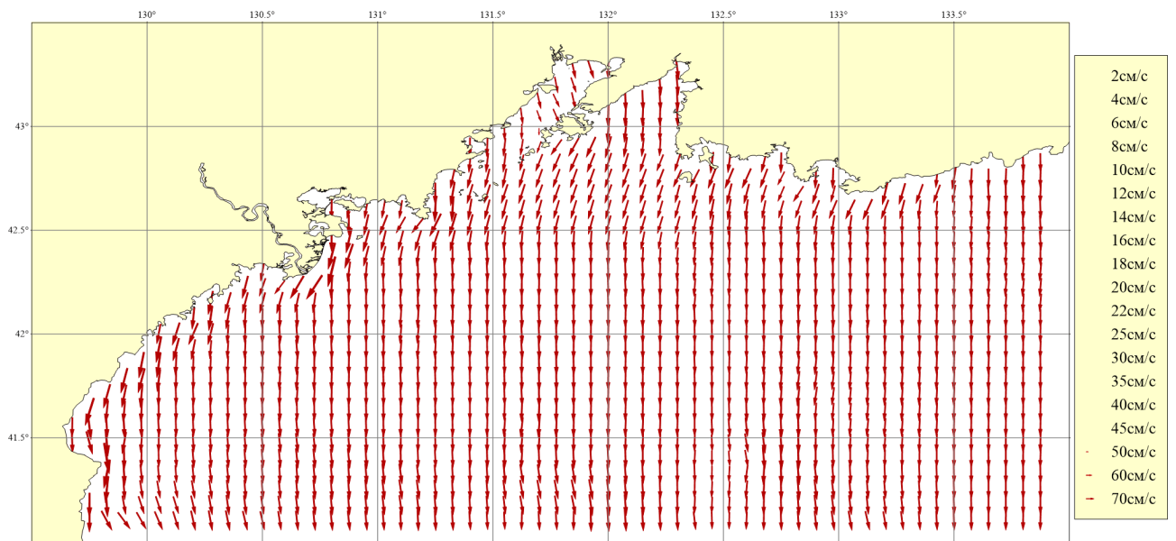
Рисунок 251. Месяц: Октябрь; Горизонт: 0м; Ветер: Северо-Западный сильный (16 м/сек)
