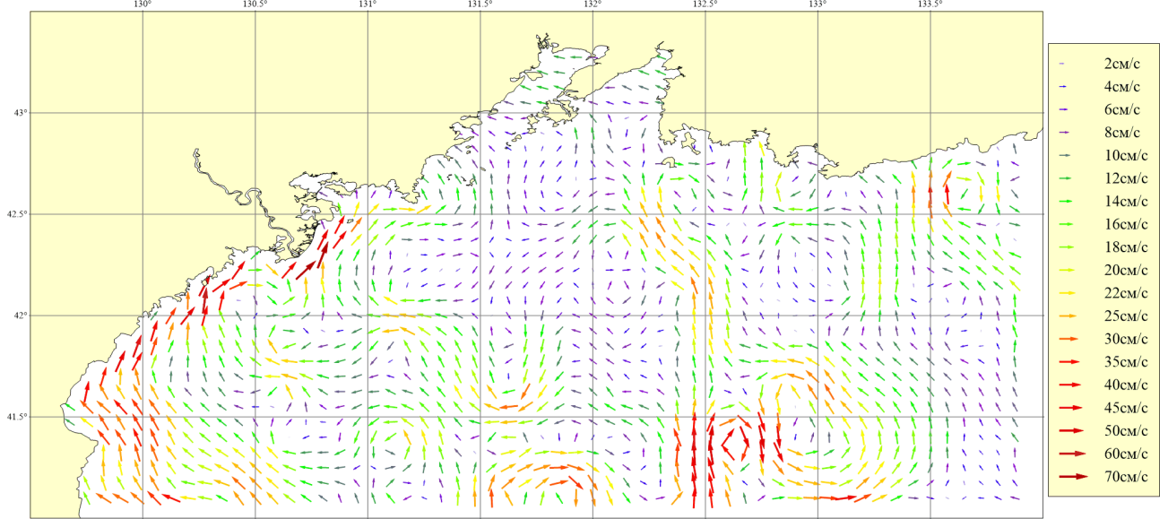
Рисунок 232. Месяц: Октябрь; Горизонт: 0м; Ветер: Восточный слабый (4 м/сек)
