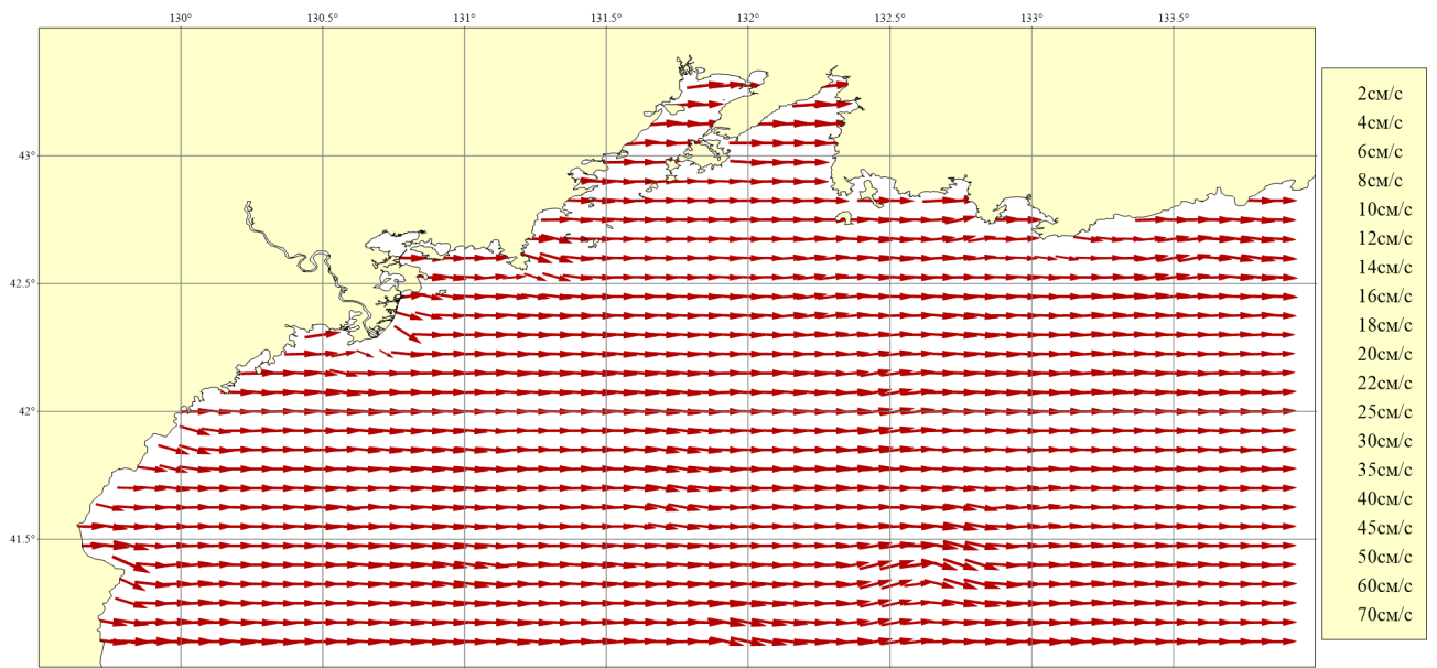
Рисунок 245. Месяц: Октябрь; Горизонт: 0м; Ветер: Юго-Западный сильный (16 м/сек)
