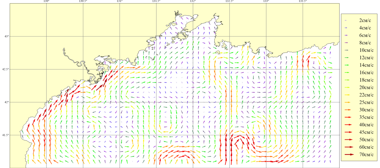
Рисунок 231. Месяц: Октябрь; Горизонт: 0м; Ветер: Юго-Восточный слабый (4 м/сек)
