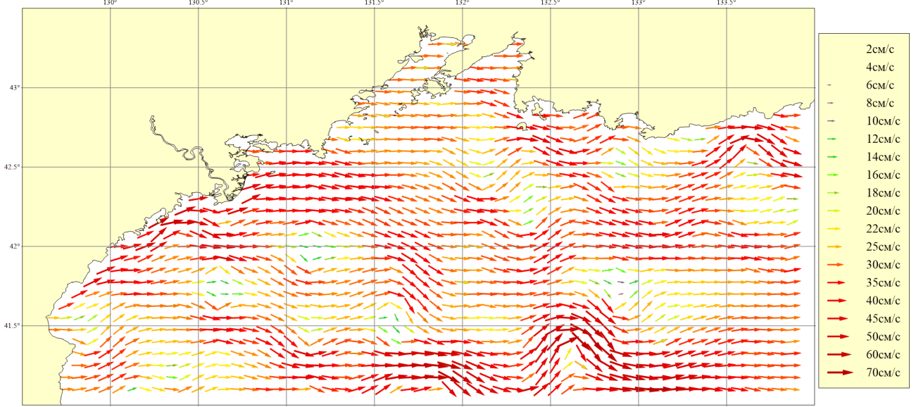
Рисунок 237. Месяц: Октябрь; Горизонт: 0м; Ветер: Юго-Западный умеренный (8 м/сек)
