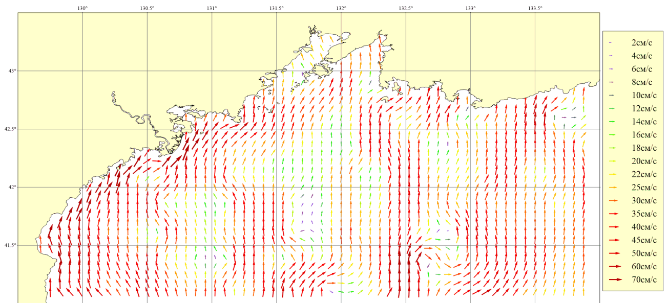
Рисунок 239. Месяц: Октябрь; Горизонт: 0м; Ветер: Юго-Восточный умеренный (8 м/сек)
