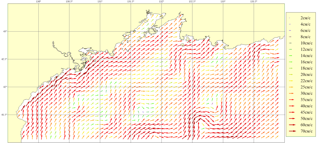
Рисунок 238. Месяц: Октябрь; Горизонт: 0м; Ветер: Южный умеренный (8 м/сек)
