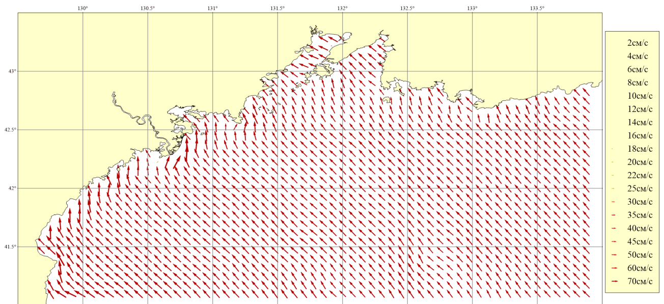
Рисунок 248. Месяц: Октябрь; Горизонт: 0м; Ветер: Восточный сильный (16 м/сек)
