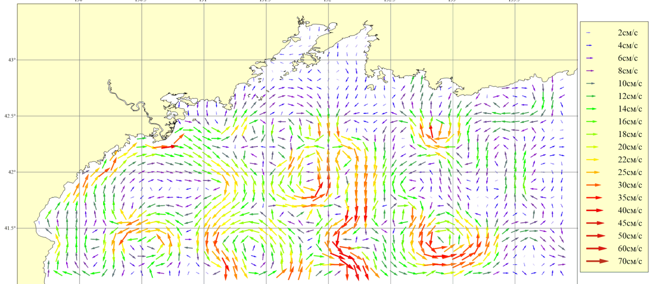
Рисунок 252. Месяц: Ноябрь; Горизонт: 0м; Ветер: Штиль
