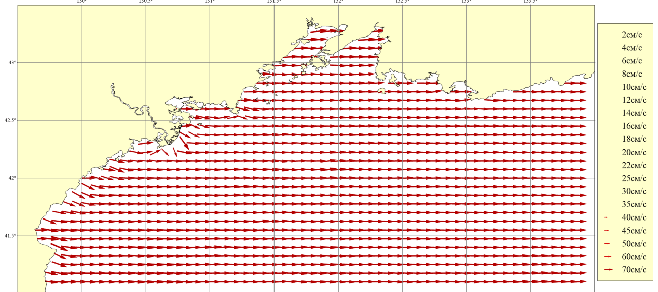
Рисунок 45. Месяц: Февраль; Горизонт: 0м; Ветер: Юго-Западный сильный (16 м/сек)
