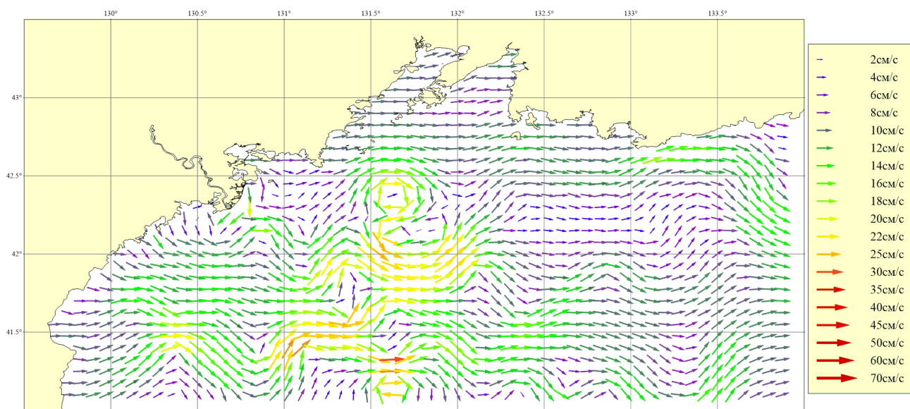
Рисунок 29. Месяц: Февраль; Горизонт: 0м; Ветер: Юго-Западный слабый (4 м/сек)
