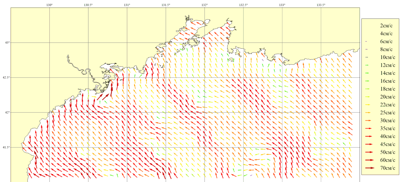
Рисунок 65. Месяц: Март; Горизонт: 0м; Ветер: Восточный умеренный (8 м/сек)
