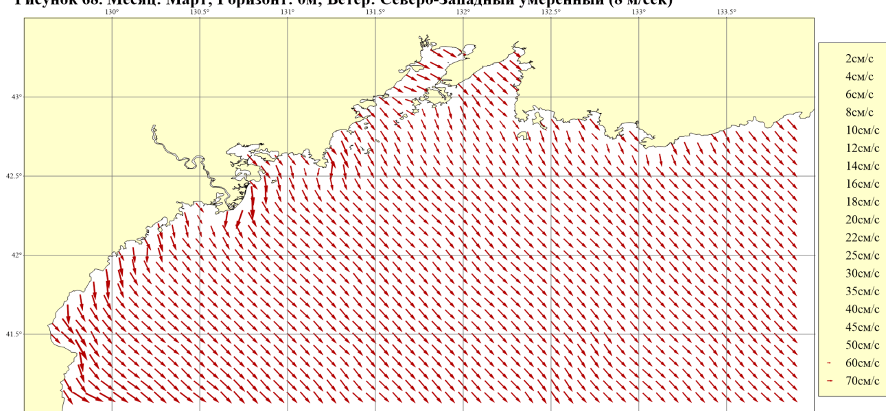
Рисунок 69. Месяц: Март; Горизонт: 0м; Ветер: Западный сильный (16 м/сек)
