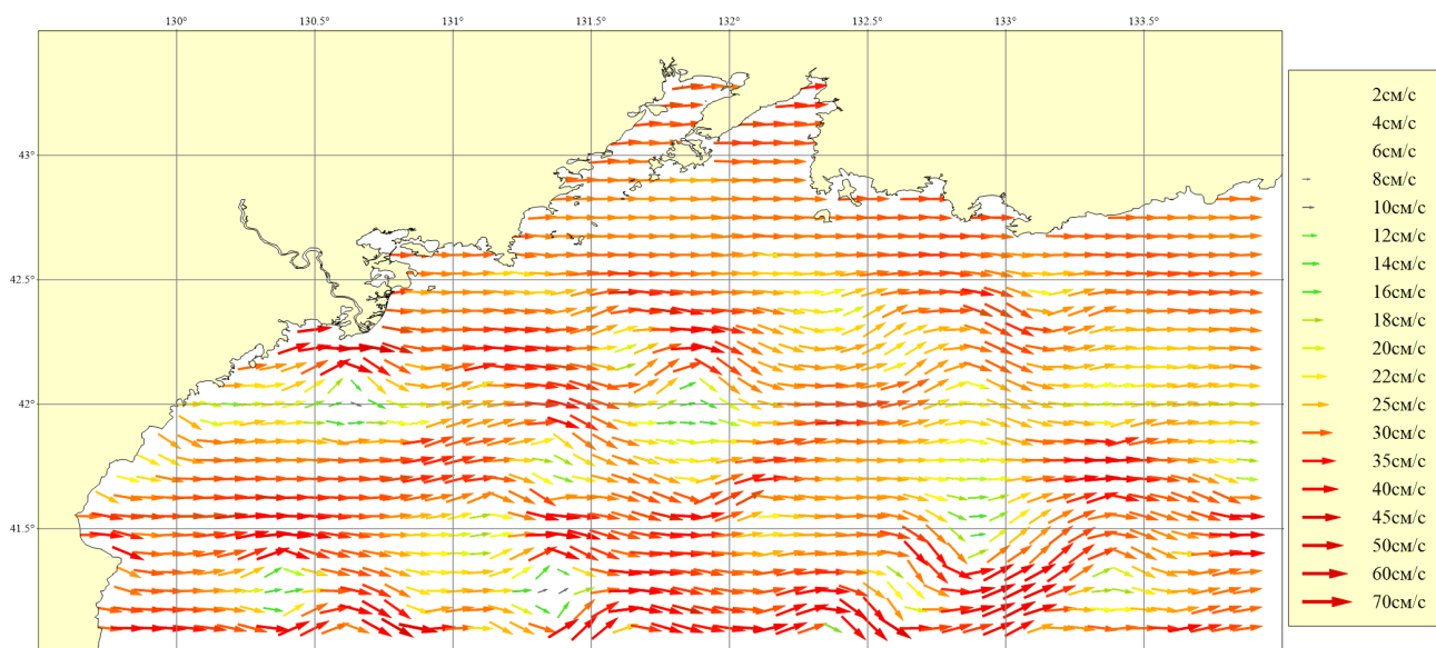
Рисунок 62. Месяц: Март; Горизонт: 0м; Ветер: Юго-Западный умеренный (8 м/сек)
