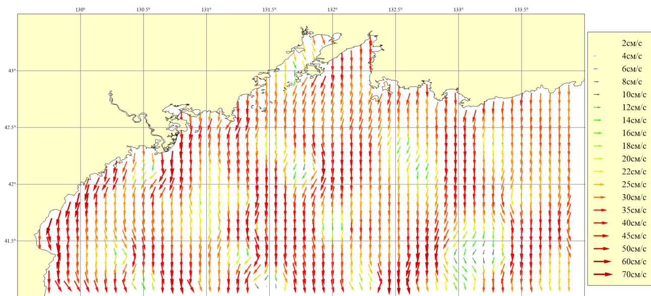
Рисунок 68. Месяц: Март; Горизонт: 0м; Ветер: Северо-Западный умеренный (8 м/сек)
