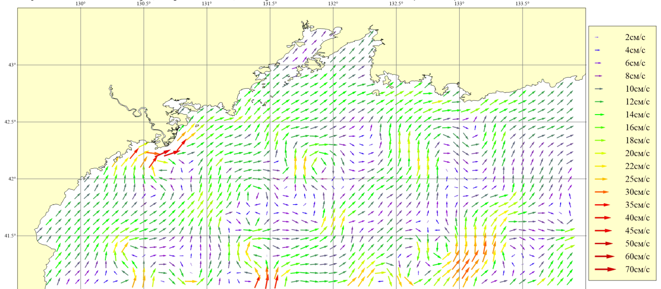
Рисунок 55. Месяц: Март; Горизонт: 0м; Ветер: Южный слабый (4 м/сек)
