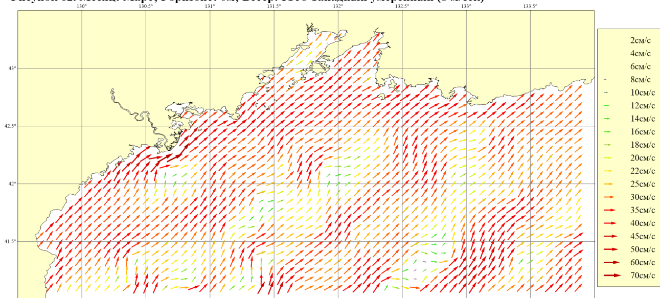
Рисунок 63. Месяц: Март; Горизонт: 0м; Ветер: Южный умеренный (8 м/сек)
