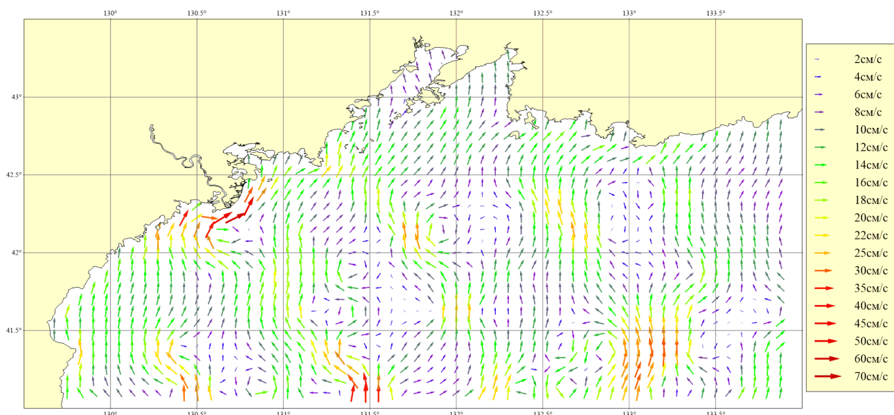
Рисунок 56. Месяц: Март; Горизонт: 0м; Ветер: Юго-Восточный слабый (4 м/сек)
