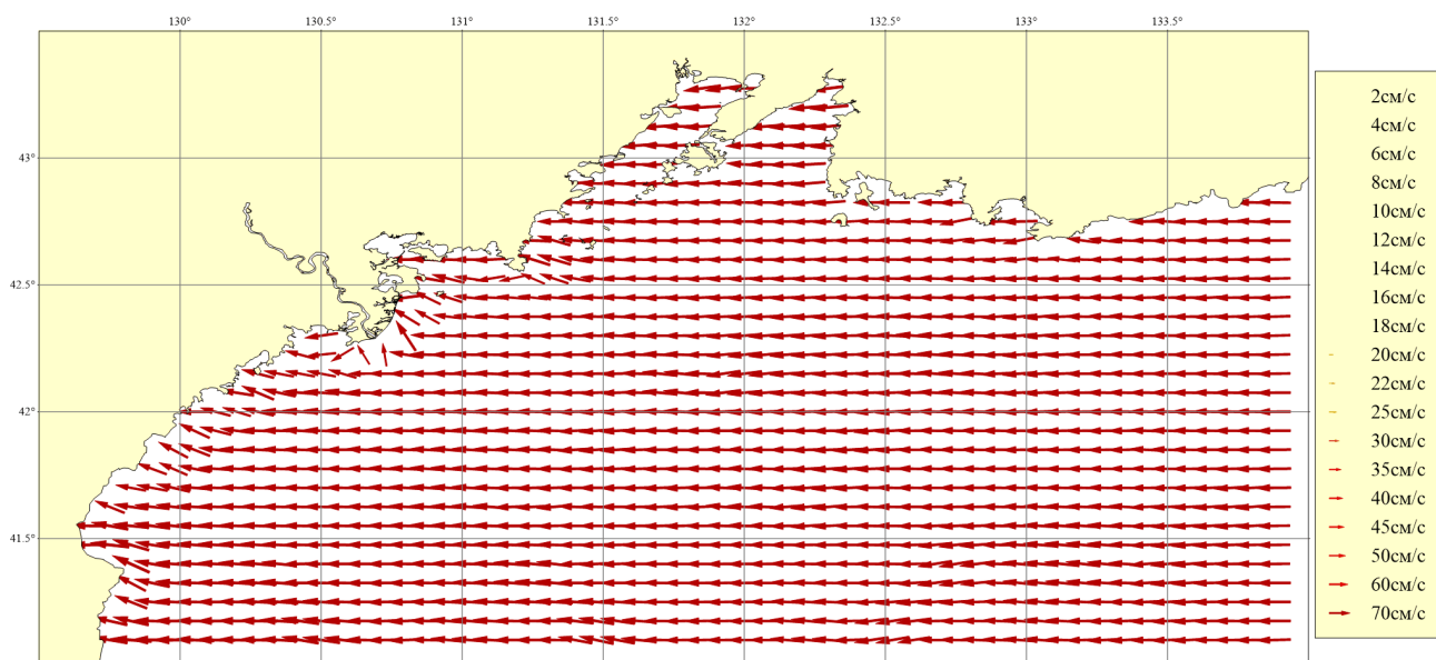
Рисунок 74. Месяц: Март; Горизонт: 0м; Ветер: Северо-Восточный сильный (16 м/сек)
