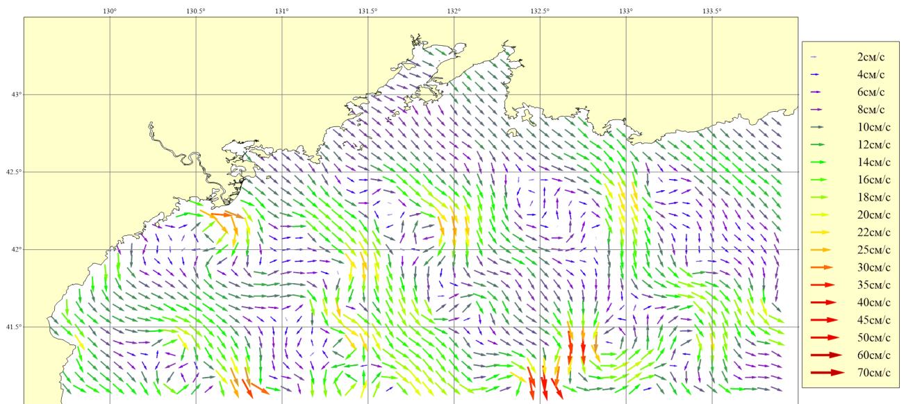
Рисунок 53. Месяц: Март; Горизонт: 0м; Ветер: Западный слабый (4 м/сек)
