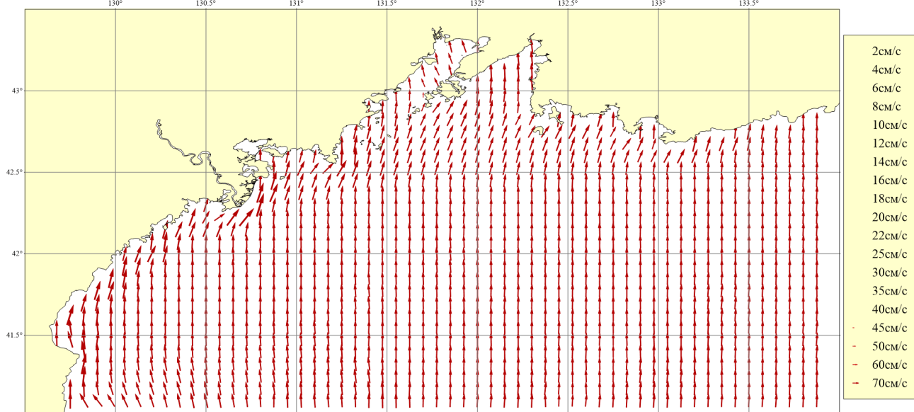
Рисунок 72. Месяц: Март; Горизонт: 0м; Ветер: Юго-Восточный сильный (16 м/сек)
