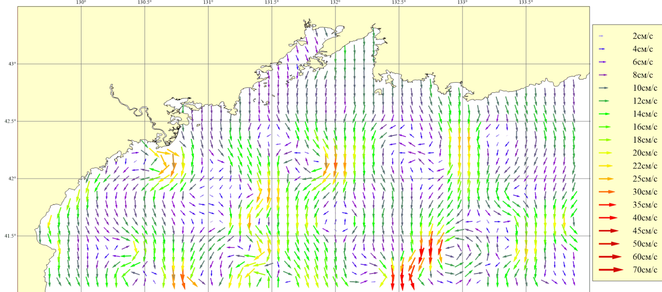
Рисунок 60. Месяц: Март; Горизонт: 0м; Ветер: Северо-Западный слабый (4 м/сек)
