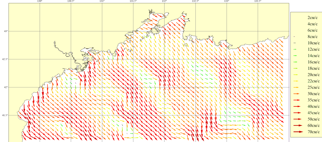
Рисунок 61. Месяц: Март; Горизонт: 0м; Ветер: Западный умеренный (8 м/сек)
