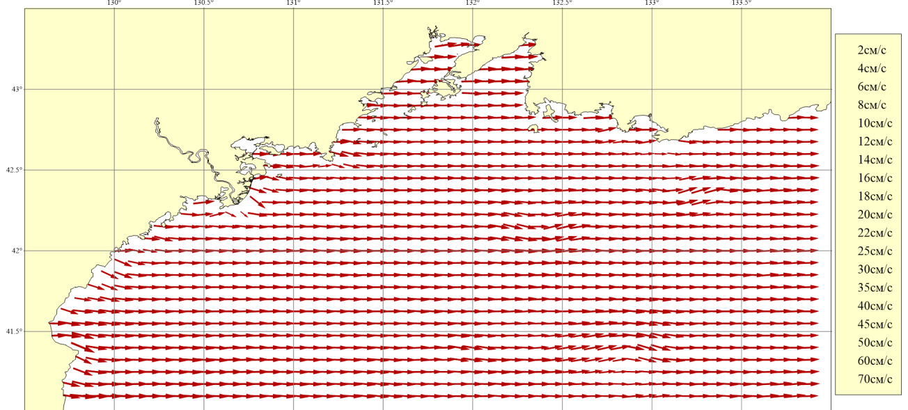
Рисунок 120. Месяц: Май; Горизонт: 0м; Ветер: Юго-Западный сильный (16 м/сек)
