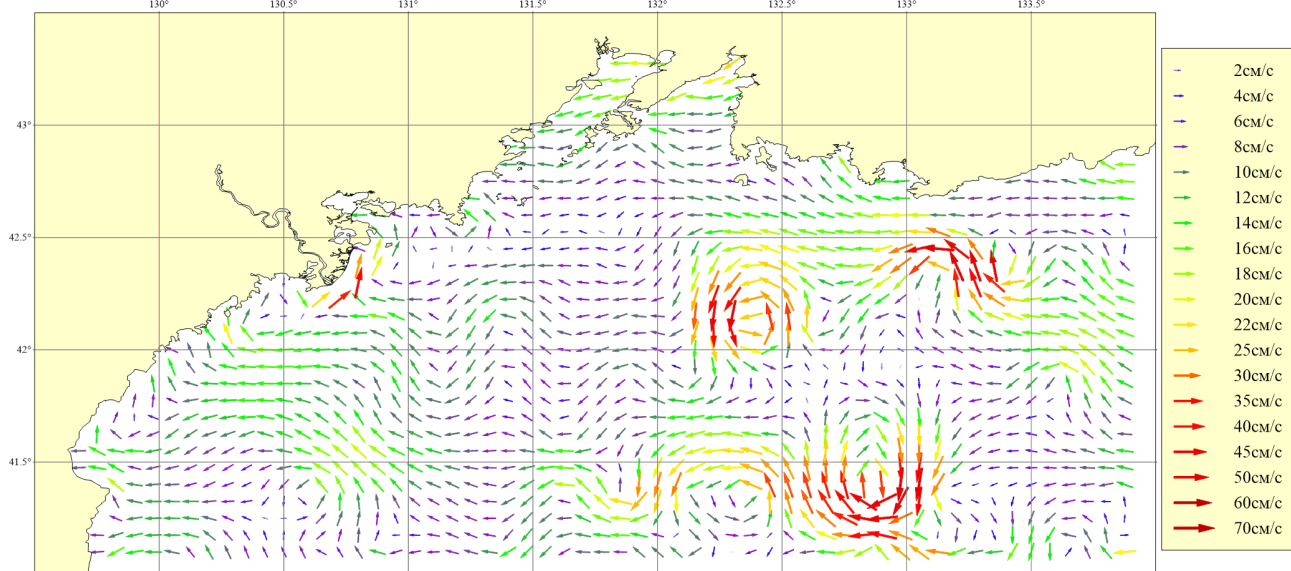
Рисунок 108. Месяц: Май; Горизонт: 0м; Ветер: Северо-Восточный слабый (4 м/сек)
