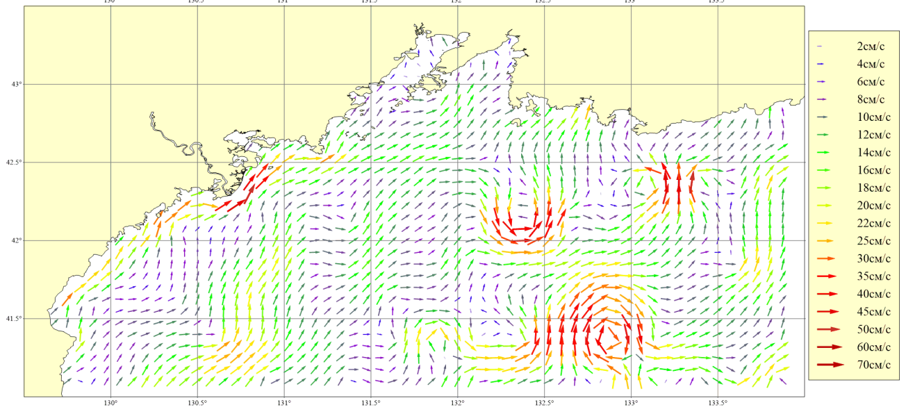
Рисунок 105. Месяц: Май; Горизонт: 0м; Ветер: Южный слабый (4 м/сек)
