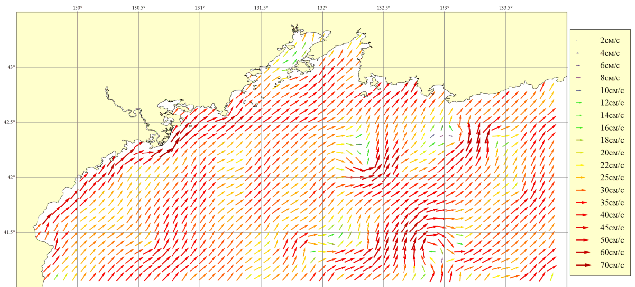
Рисунок 113. Месяц: Май; Горизонт: 0м; Ветер: Южный умеренный (8 м/сек)
