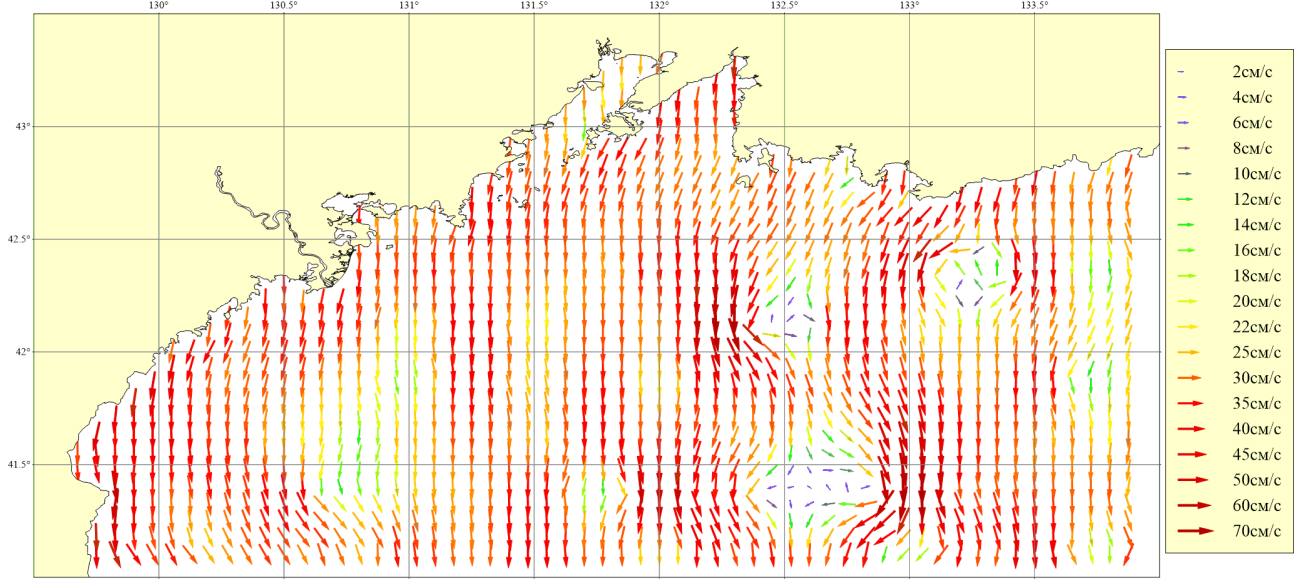
Рисунок 118. Месяц: Май; Горизонт: 0м; Ветер: Северо-Западный умеренный (8 м/сек)
