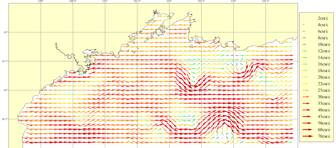
Рисунок 112. Месяц: Май; Горизонт: 0м; Ветер: Юго-Западный умеренный (8 м/сек)
