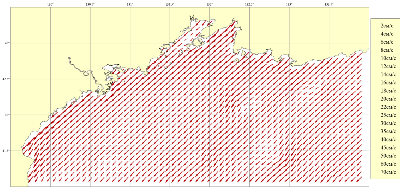
Рисунок 125. Месяц: Май; Горизонт: 0м; Ветер: Северный сильный (16 м/сек)
