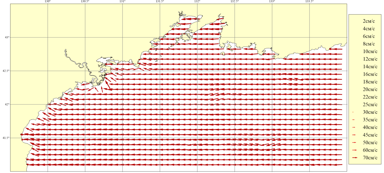
Рисунок 124. Месяц: Май; Горизонт: 0м; Ветер: Северо-Восточный сильный (16 м/сек)
