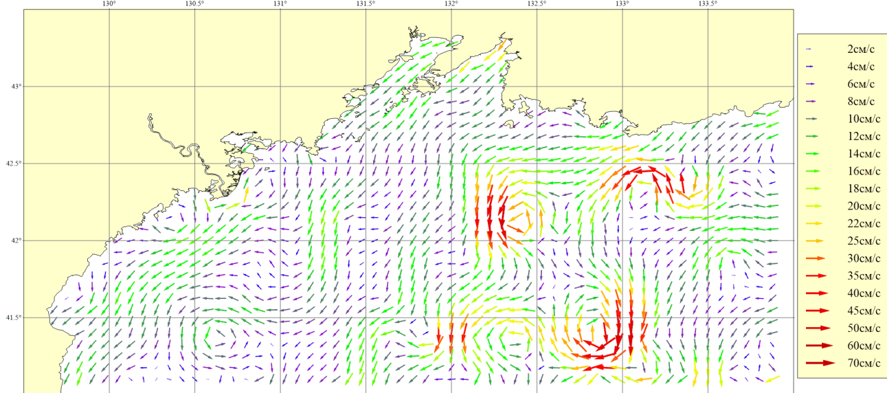
Рисунок 109. Месяц: Май; Горизонт: 0м; Ветер: Северный слабый (4 м/сек)
