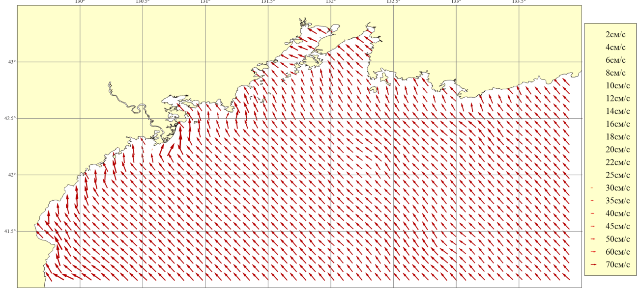
Рисунок 123. Месяц: Май; Горизонт: 0м; Ветер: Восточный сильный (16 м/сек)
