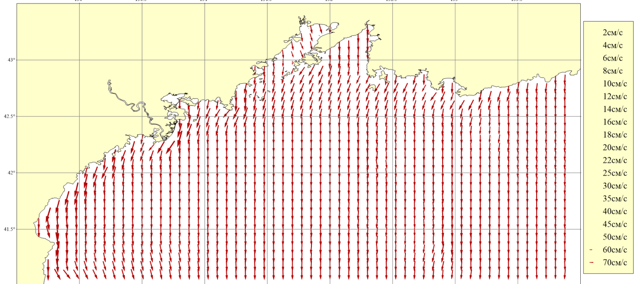
Рисунок 126. Месяц: Май; Горизонт: 0м; Ветер: Северо-Западный сильный (16 м/сек)
