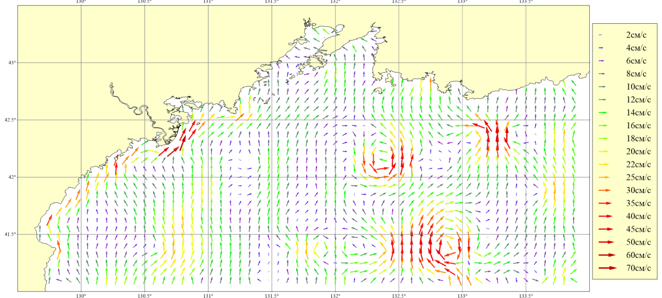
Рисунок 106. Месяц: Май; Горизонт: 0м; Ветер: Юго-Восточный слабый (4 м/сек)
