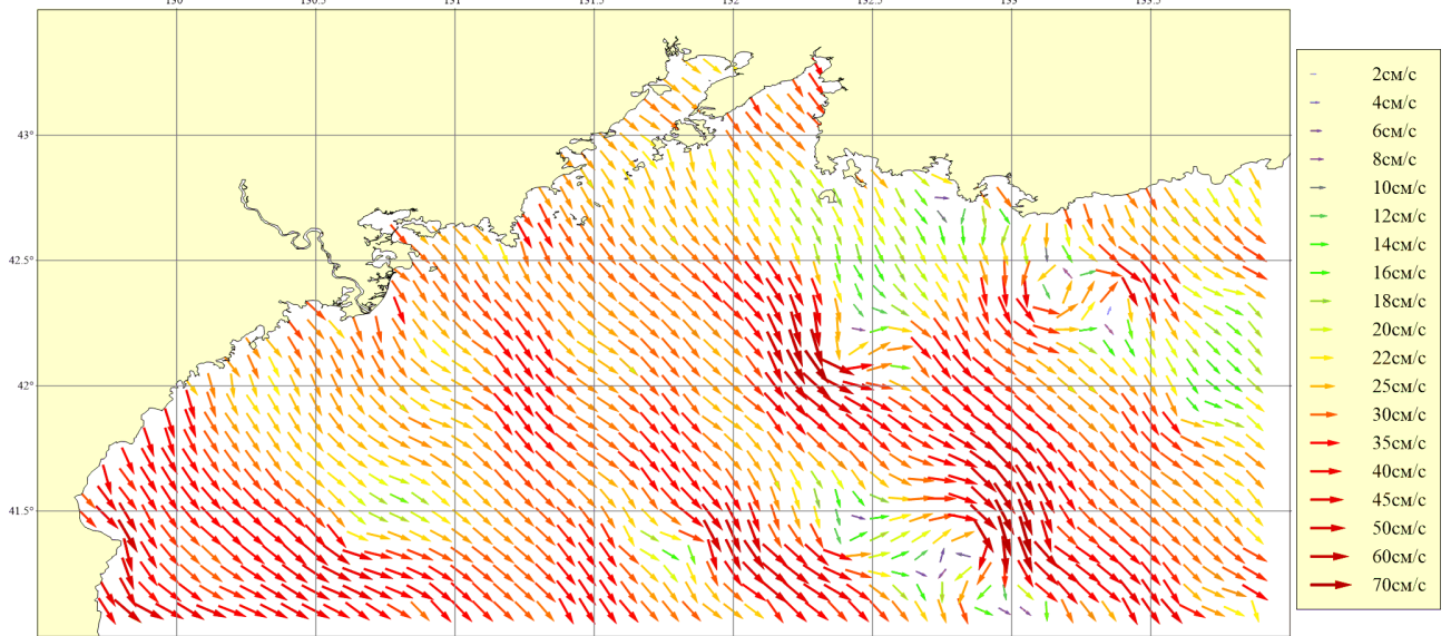
Рисунок 111. Месяц: Май; Горизонт: 0м; Ветер: Западный умеренный (8 м/сек)
