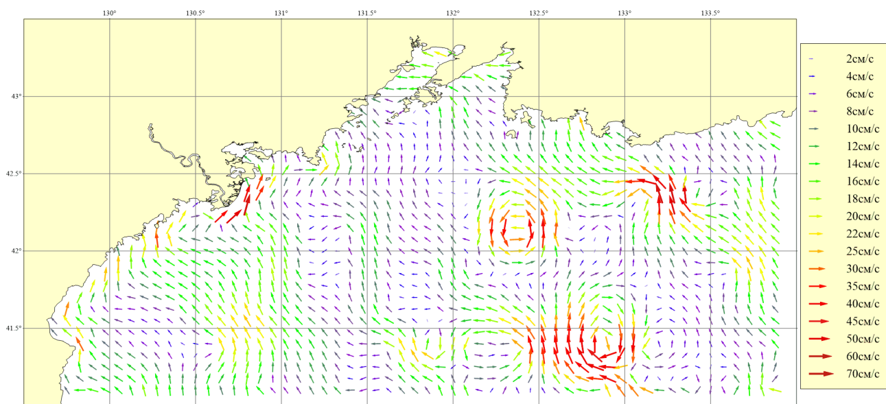
Рисунок 107. Месяц: Май; Горизонт: 0м; Ветер: Восточный слабый (4 м/сек)
