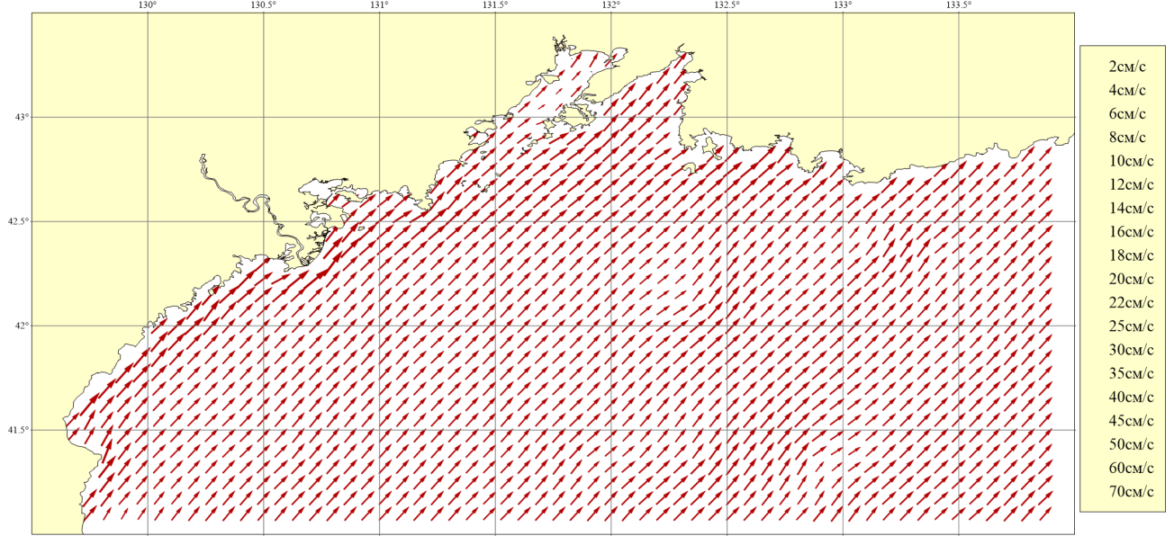
Рисунок 121. Месяц: Май; Горизонт: 0м; Ветер: Южный сильный (16 м/сек)
