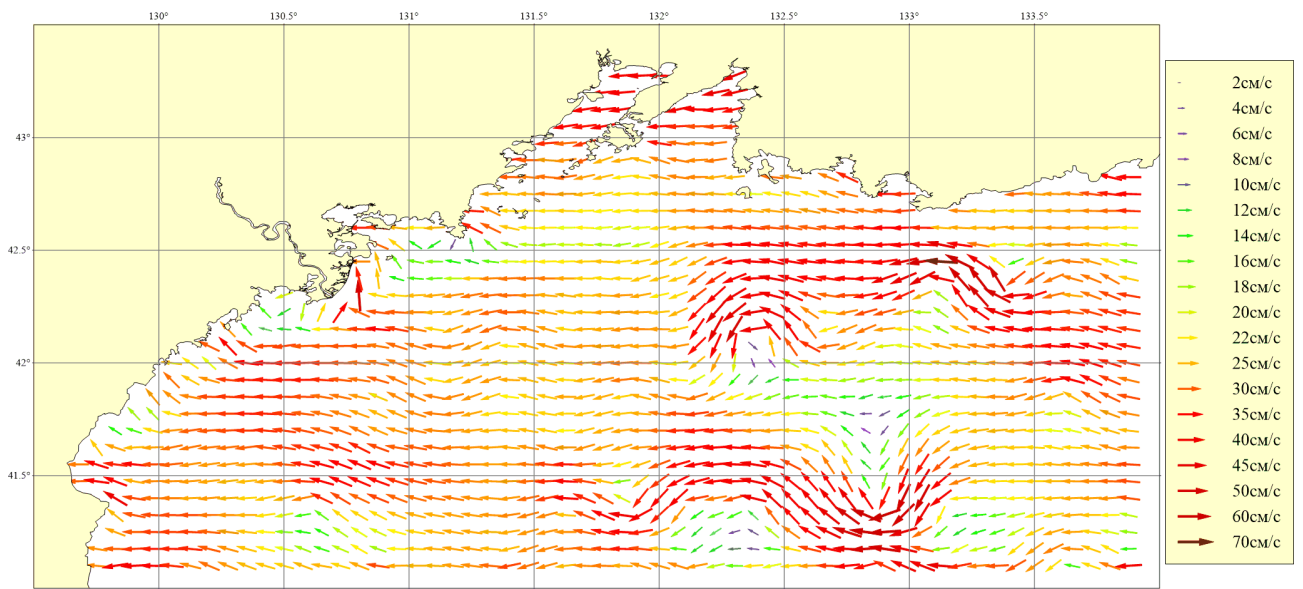
Рисунок 116. Месяц: Май; Горизонт: 0м; Ветер: Северо-Восточный умеренный (8 м/сек)
