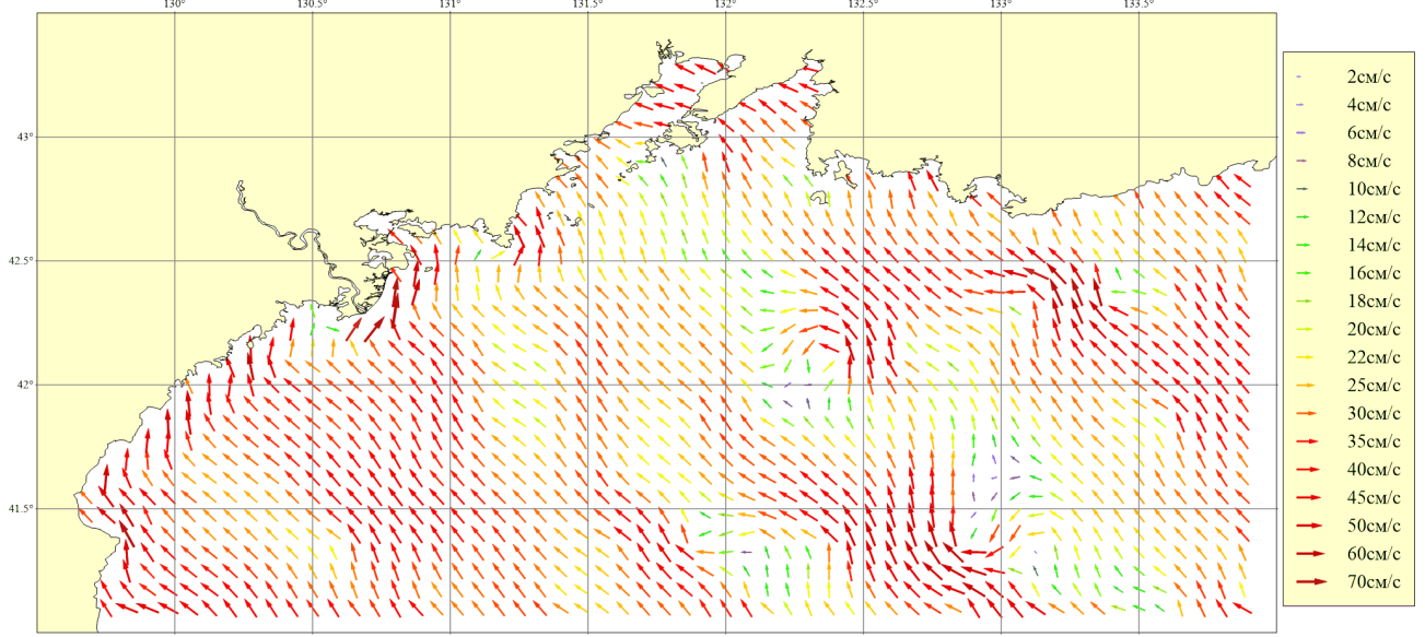
Рисунок 115. Месяц: Май; Горизонт: 0м; Ветер: Восточный умеренный (8 м/сек)
