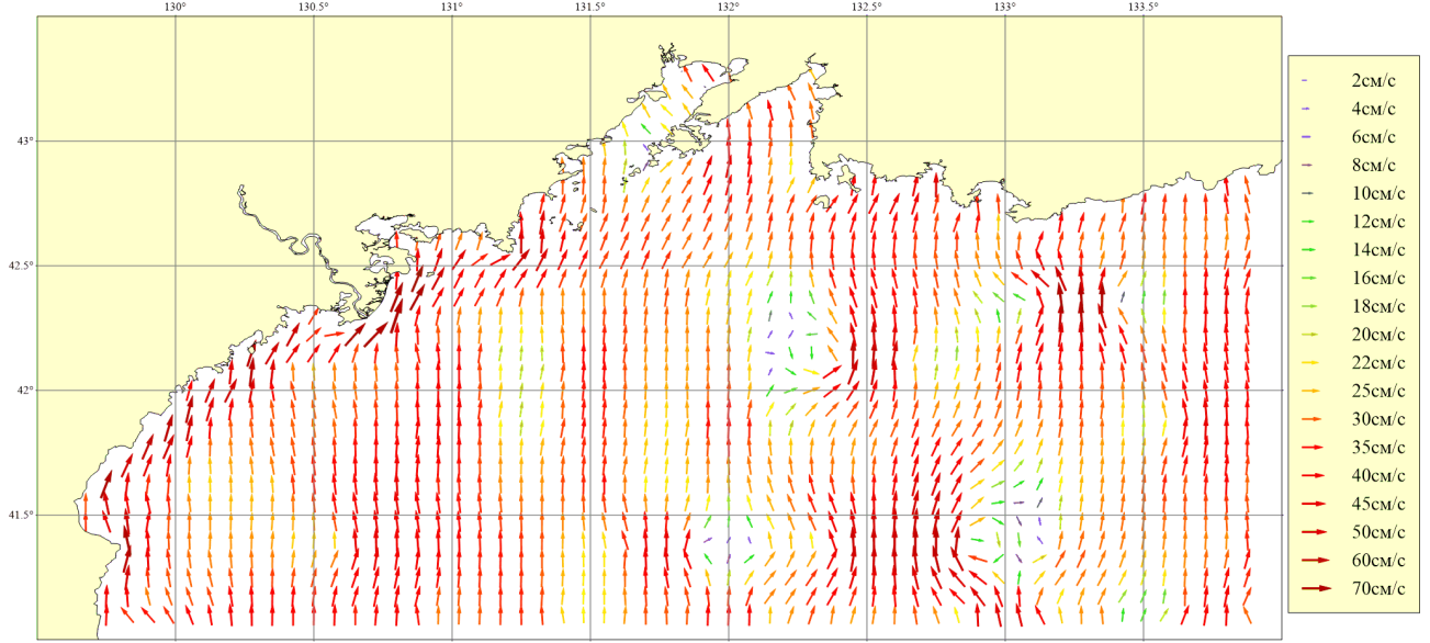
Рисунок 114. Месяц: Май; Горизонт: 0м; Ветер: Юго-Восточный умеренный (8 м/сек)
