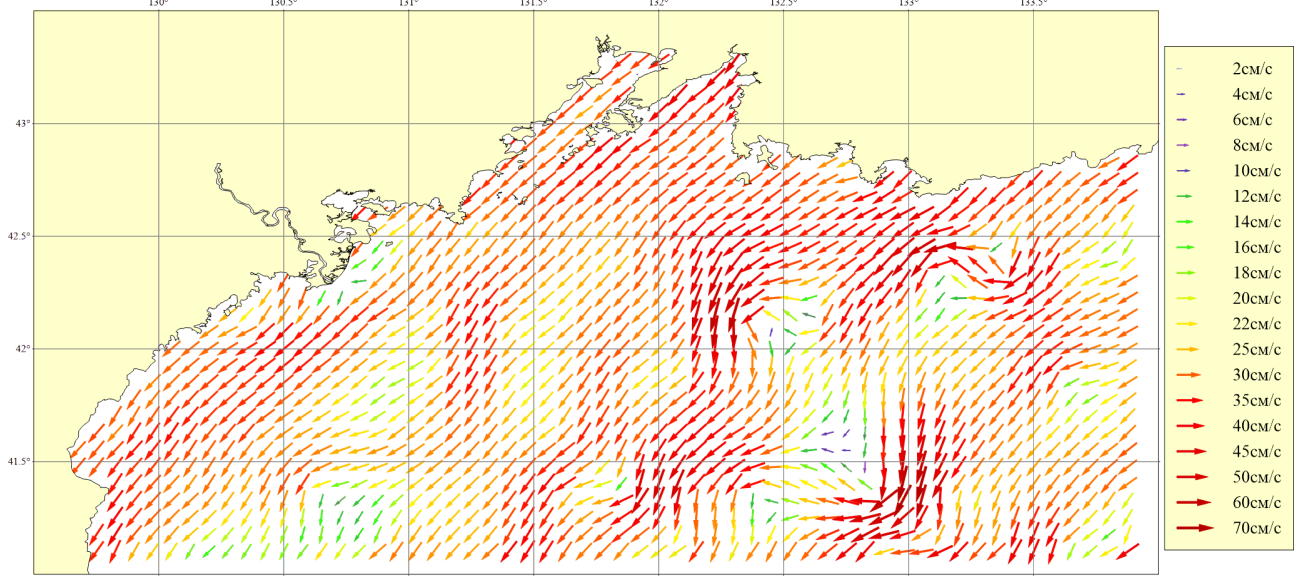
Рисунок 117. Месяц: Май; Горизонт: 0м; Ветер: Северный умеренный (8 м/сек)
