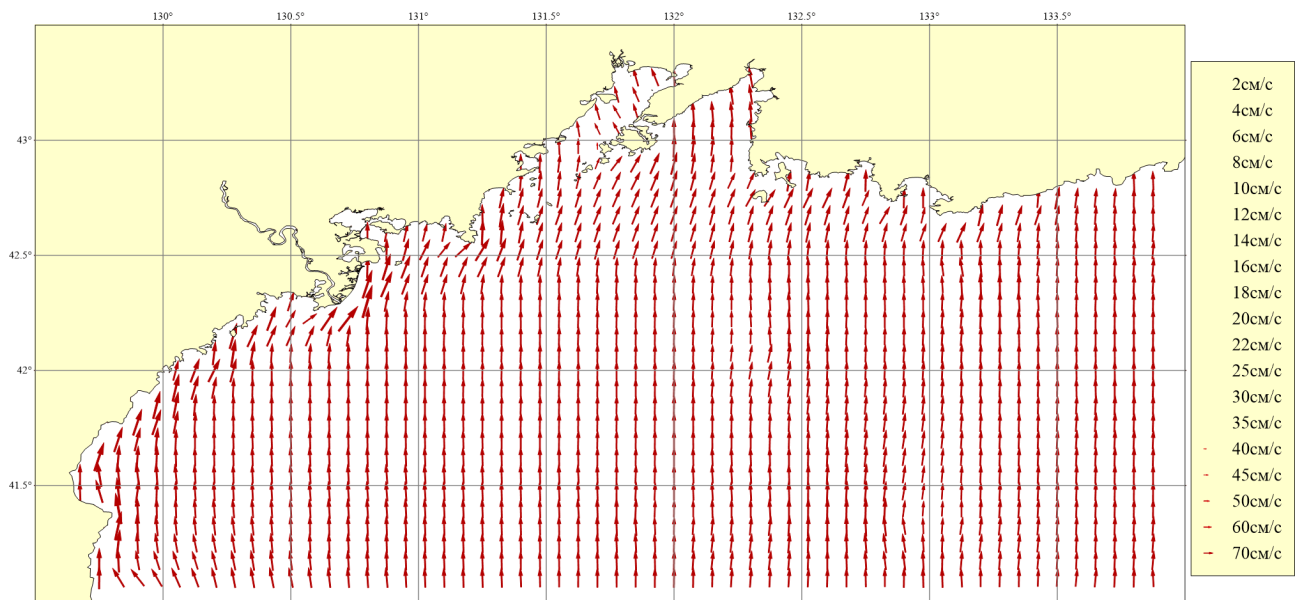
Рисунок 122. Месяц: Май; Горизонт: 0м; Ветер: Юго-Восточный сильный (16 м/сек)
