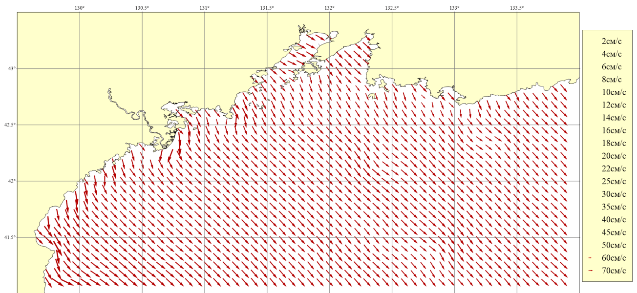
Рисунок 119. Месяц: Май; Горизонт: 0м; Ветер: Западный сильный (16 м/сек)
