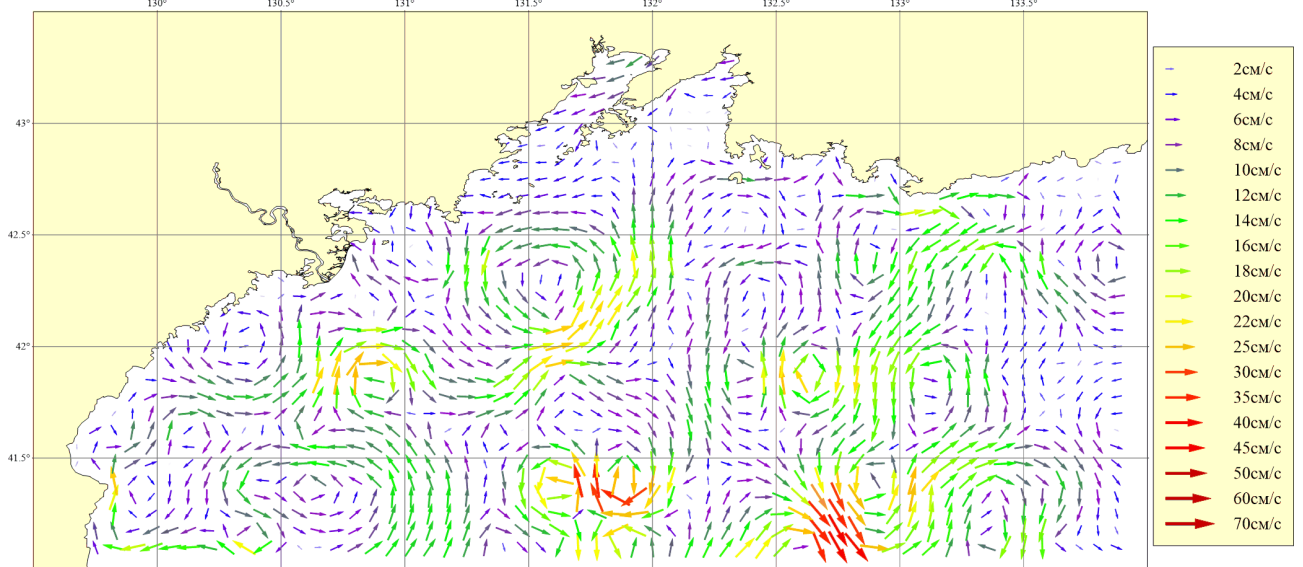
Рисунок 127. Месяц: Июнь; Горизонт: 0м; Ветер: Штиль
