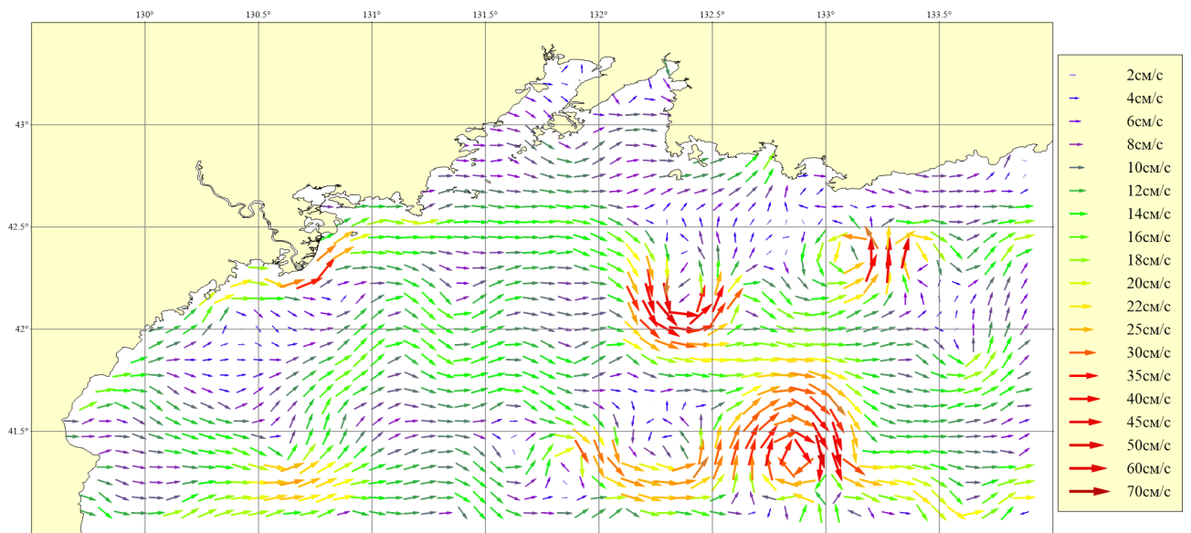
Рисунок 104. Месяц: Май; Горизонт: 0м; Ветер: Юго-Западный слабый (4 м/сек)
