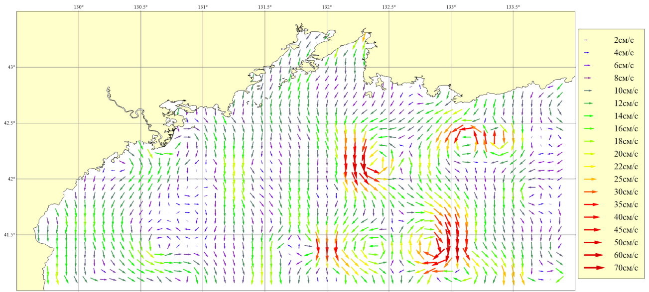
Рисунок 110. Месяц: Май; Горизонт: 0м; Ветер: Северо-Западный слабый (4 м/сек)
