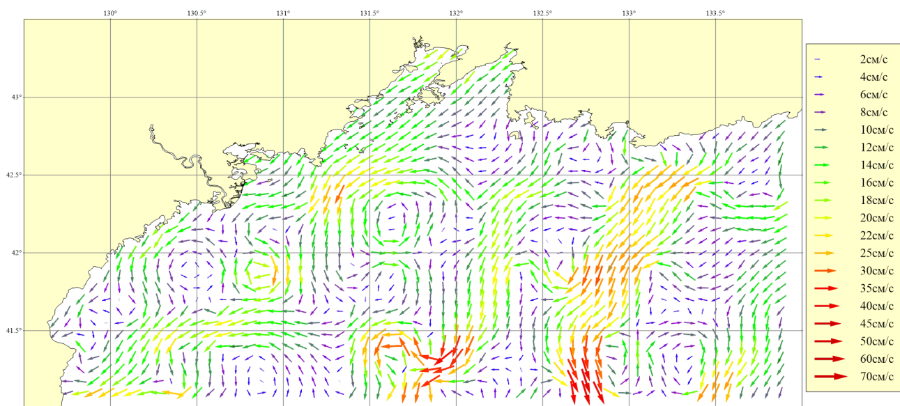
Рисунок 134. Месяц: Июнь; Горизонт: 0м; Ветер: Северный слабый (4 м/сек)
