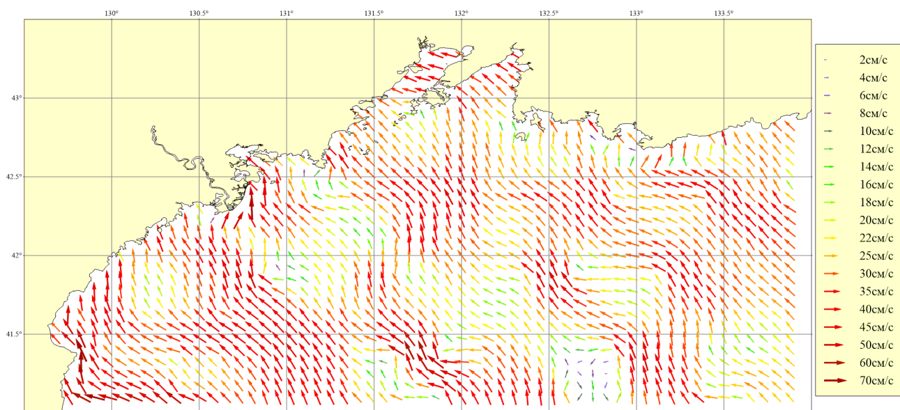
Рисунок 140. Месяц: Июнь; Горизонт: 0м; Ветер: Восточный умеренный (8 м/сек)
