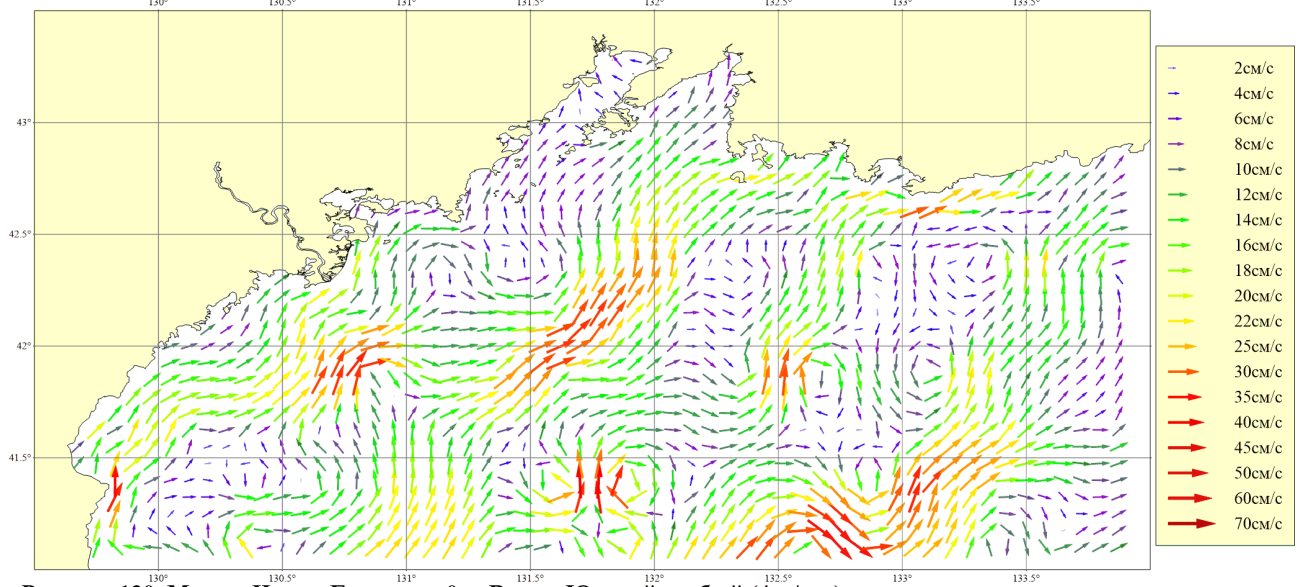
Рисунок 130. Месяц: Июнь; Горизонт: 0м; Ветер: Южный слабый (4 м/сек)
