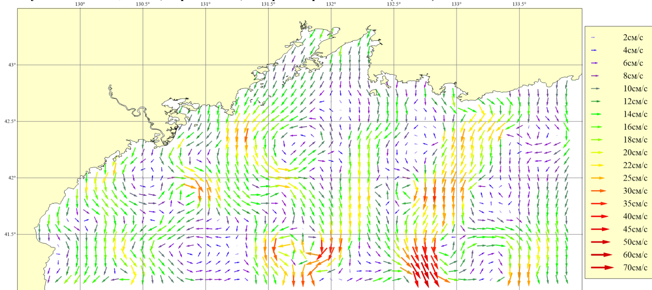
Рисунок 135. Месяц: Июнь; Горизонт: 0м; Ветер: Северо-Западный слабый (4 м/сек)
