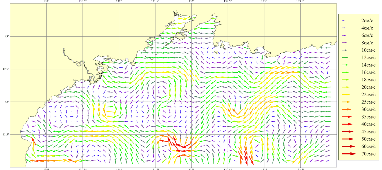
Рисунок 133. Месяц: Июнь; Горизонт: 0м; Ветер: Северо-Восточный слабый (4 м/сек)
