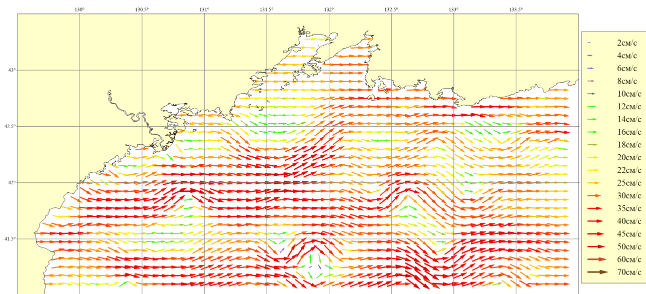
Рисунок 137. Месяц: Июнь; Горизонт: 0м; Ветер: Юго-Западный умеренный (8 м/сек)
