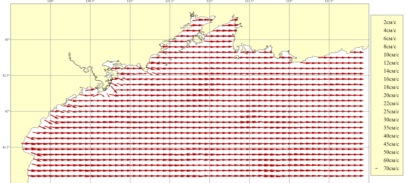
Рисунок 145. Месяц: Июнь; Горизонт: 0м; Ветер: Юго-Западный сильный (16 м/сек)
