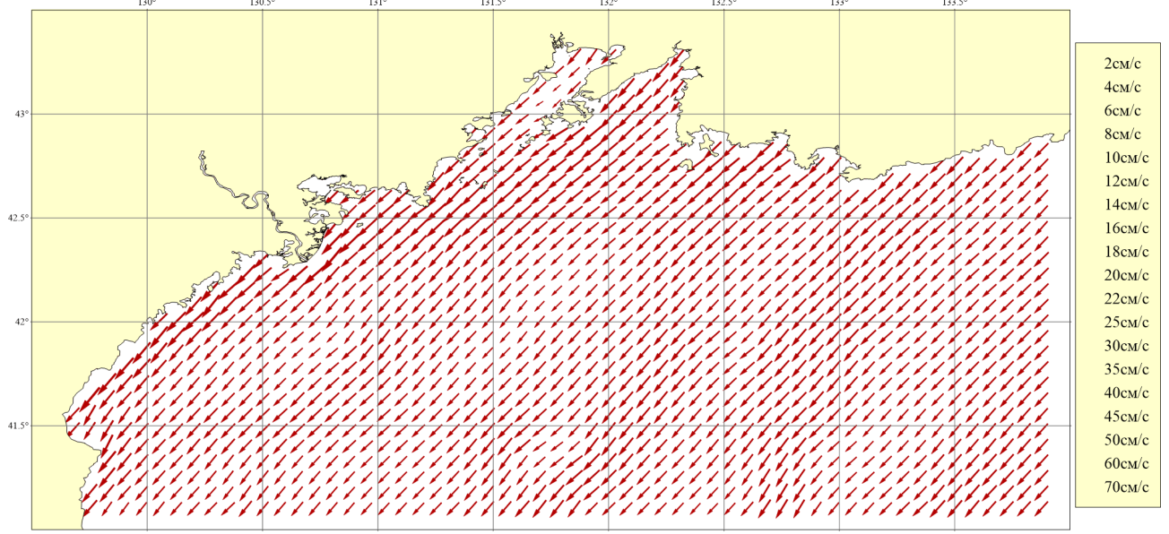
Рисунок 150. Месяц: Июнь; Горизонт: 0м; Ветер: Северный сильный (16 м/сек)
