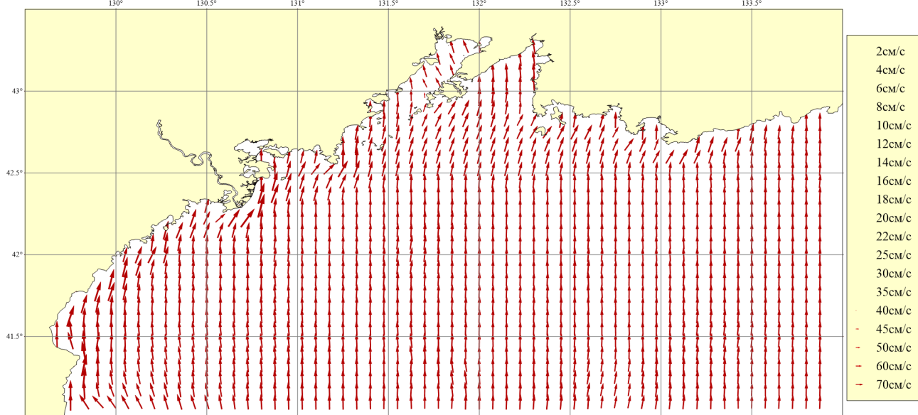
Рисунок 147. Месяц: Июнь; Горизонт: 0м; Ветер: Юго-Восточный сильный (16 м/сек)
