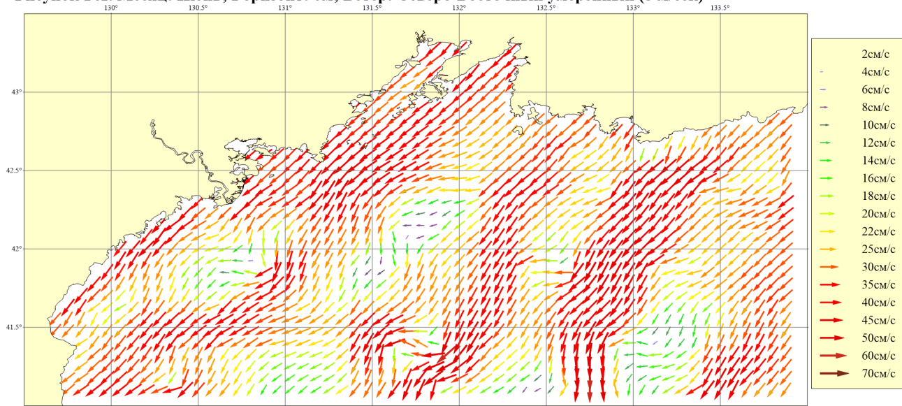
Рисунок 142. Месяц: Июнь; Горизонт: 0м; Ветер: Северный умеренный (8 м/сек)
