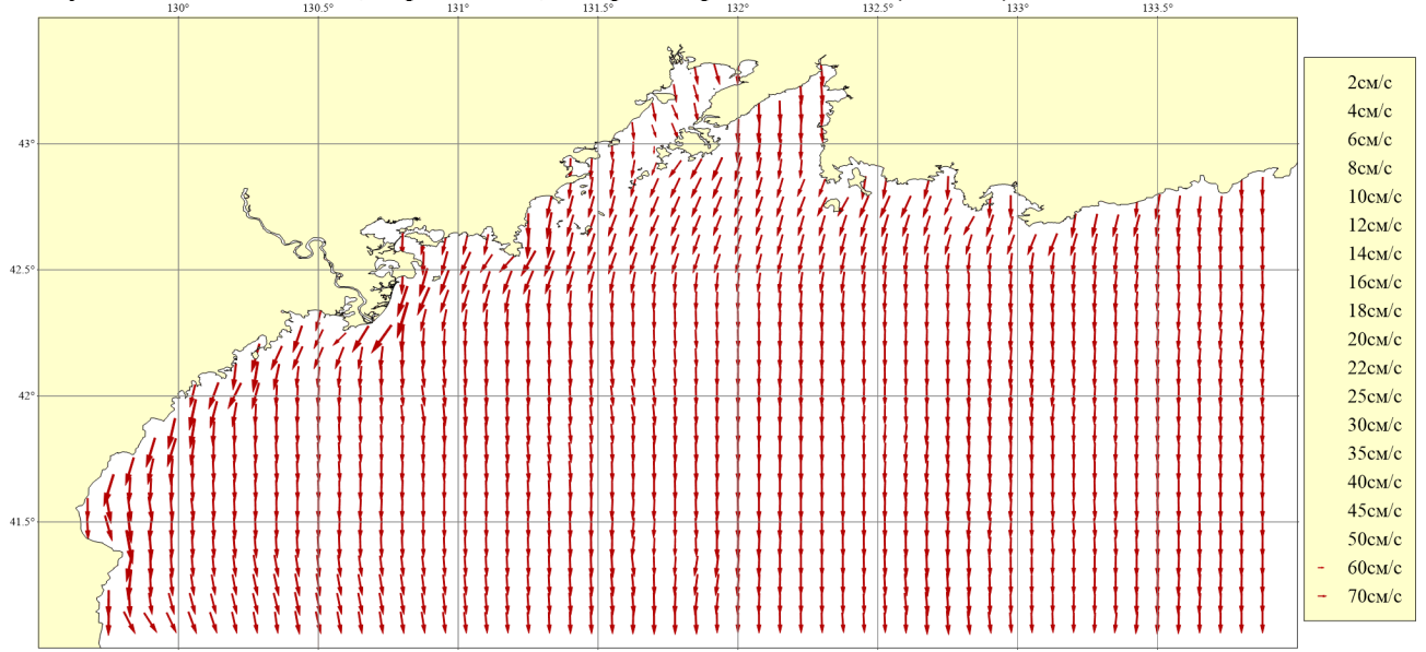
Рисунок 151. Месяц: Июнь; Горизонт: 0м; Ветер: Северо-Западный сильный (16 м/сек)
