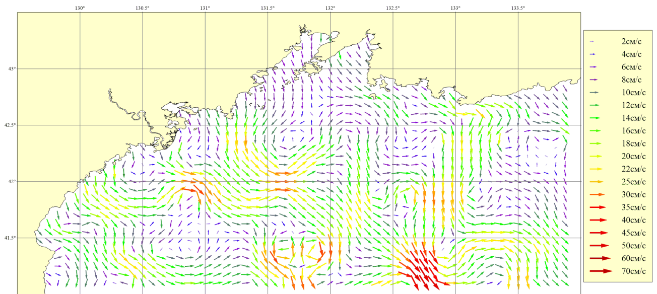
Рисунок 128. Месяц: Июнь; Горизонт: 0м; Ветер: Западный слабый (4 м/сек)
