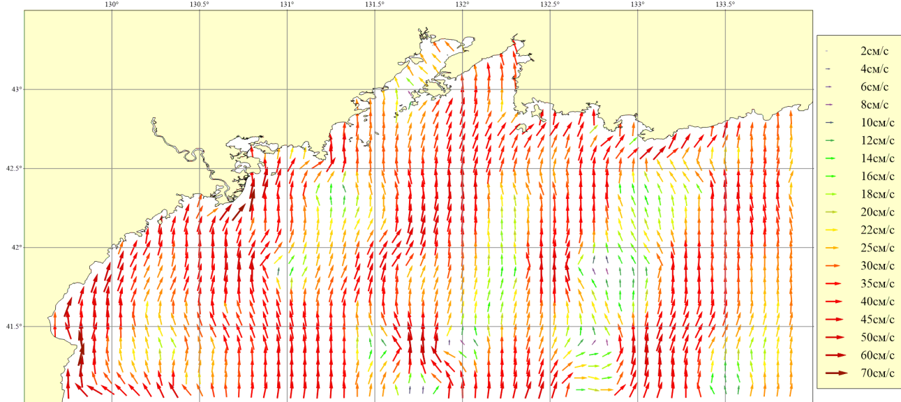
Рисунок 139. Месяц: Июнь; Горизонт: 0м; Ветер: Юго-Восточный умеренный (8 м/сек)
