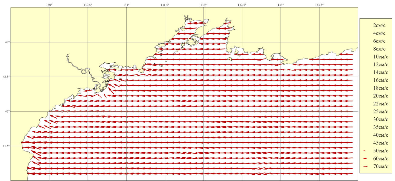
Рисунок 149. Месяц: Июнь; Горизонт: 0м; Ветер: Северо-Восточный сильный (16 м/сек)
