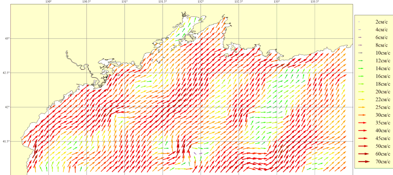
Рисунок 138. Месяц: Июнь; Горизонт: 0м; Ветер: Южный умеренный (8 м/сек)
