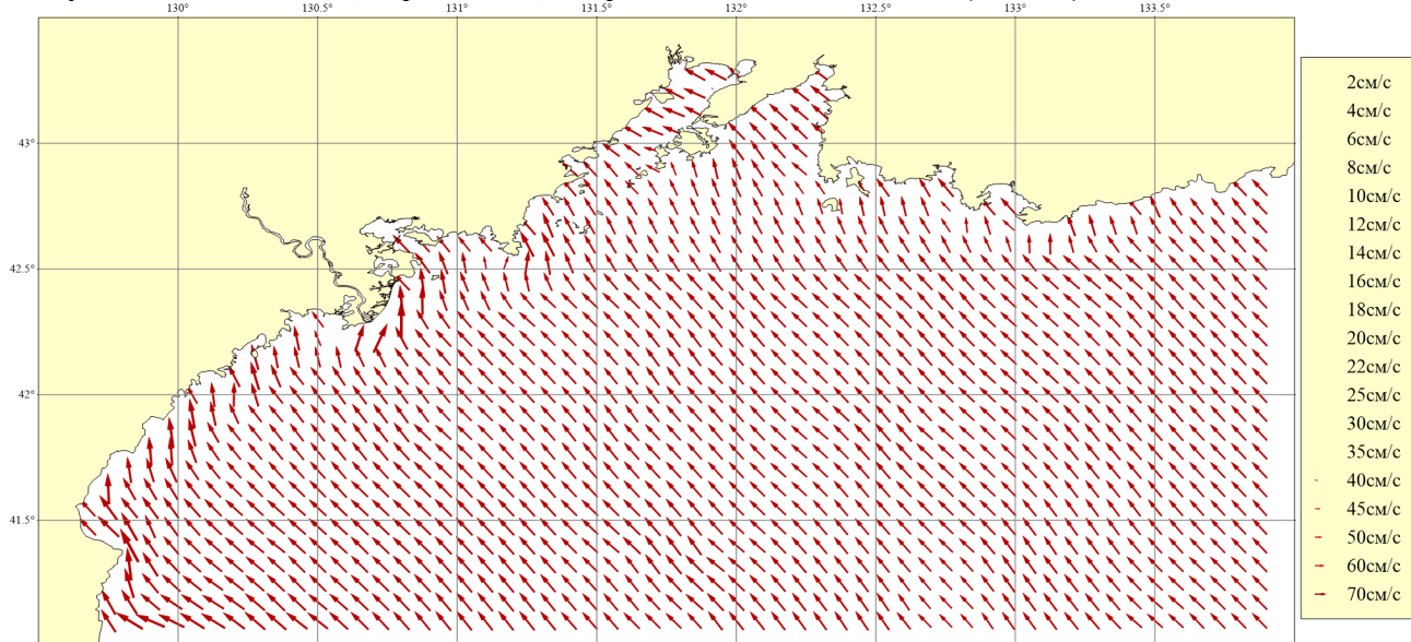
Рисунок 148. Месяц: Июнь; Горизонт: 0м; Ветер: Восточный сильный (16 м/сек)
