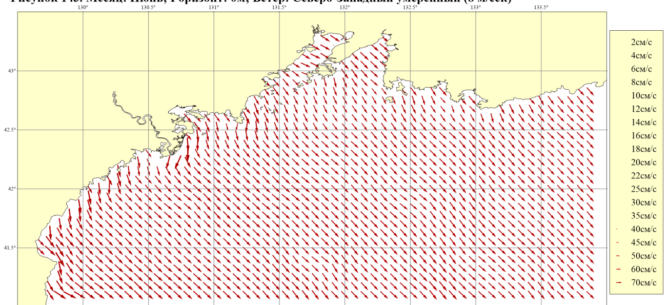
Рисунок 144. Месяц: Июнь; Горизонт: 0м; Ветер: Западный сильный (16 м/сек)
