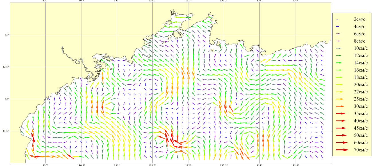
Рисунок 132. Месяц: Июнь; Горизонт: 0м; Ветер: Восточный слабый (4 м/сек)
