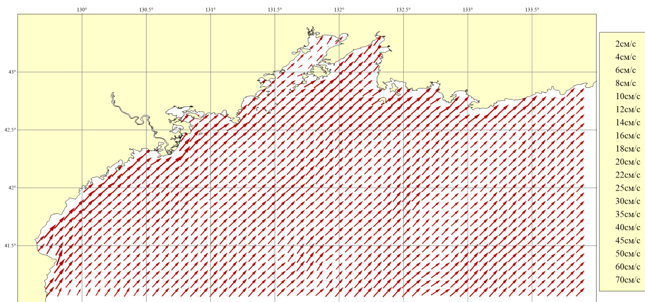
Рисунок 146. Месяц: Июнь; Горизонт: 0м; Ветер: Южный сильный (16 м/сек)
