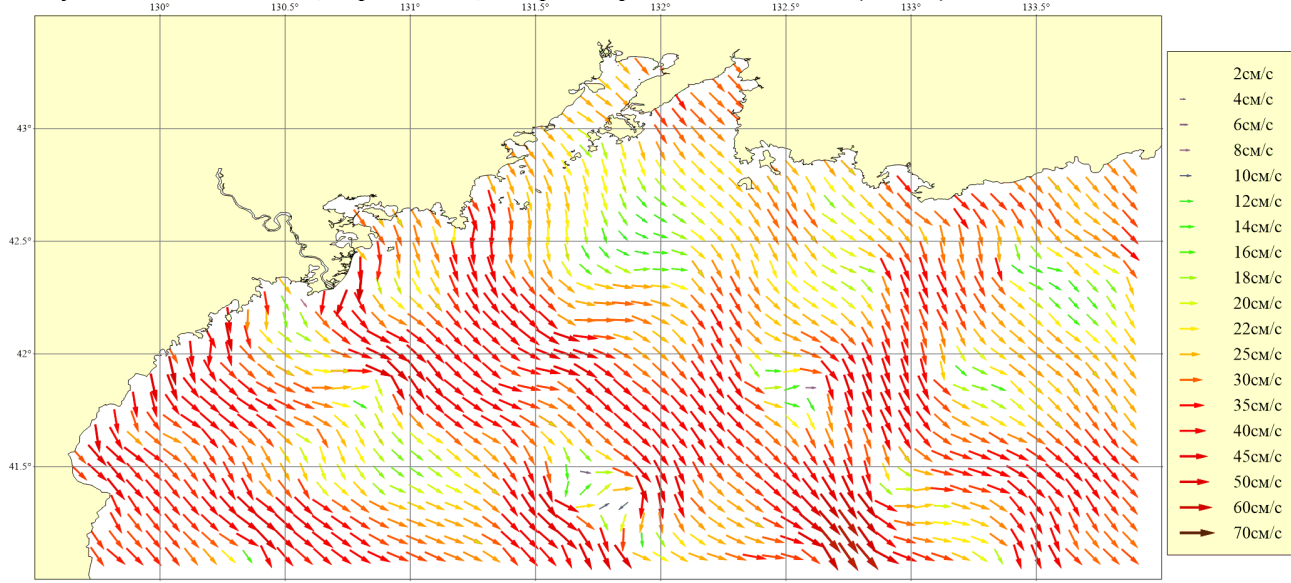
Рисунок 136. Месяц: Июнь; Горизонт: 0м; Ветер: Западный умеренный (8 м/сек)
