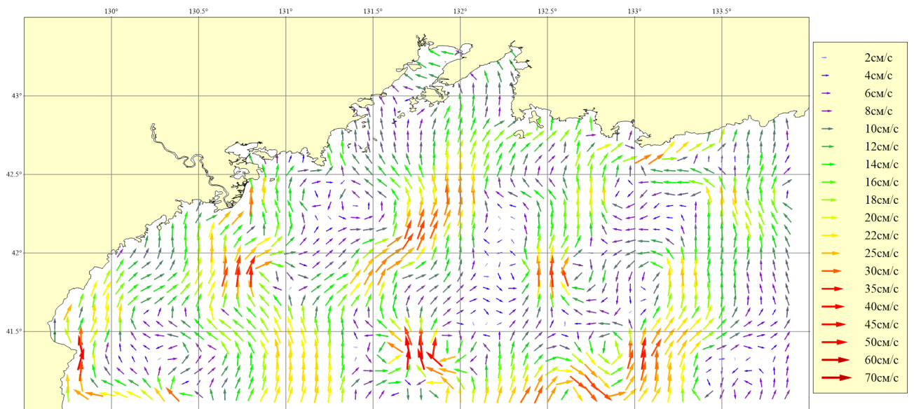
Рисунок 131. Месяц: Июнь; Горизонт: 0м; Ветер: Юго-Восточный слабый (4 м/сек)
