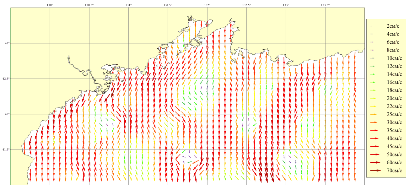
Рисунок 143. Месяц: Июнь; Горизонт: 0м; Ветер: Северо-Западный умеренный (8 м/сек)
